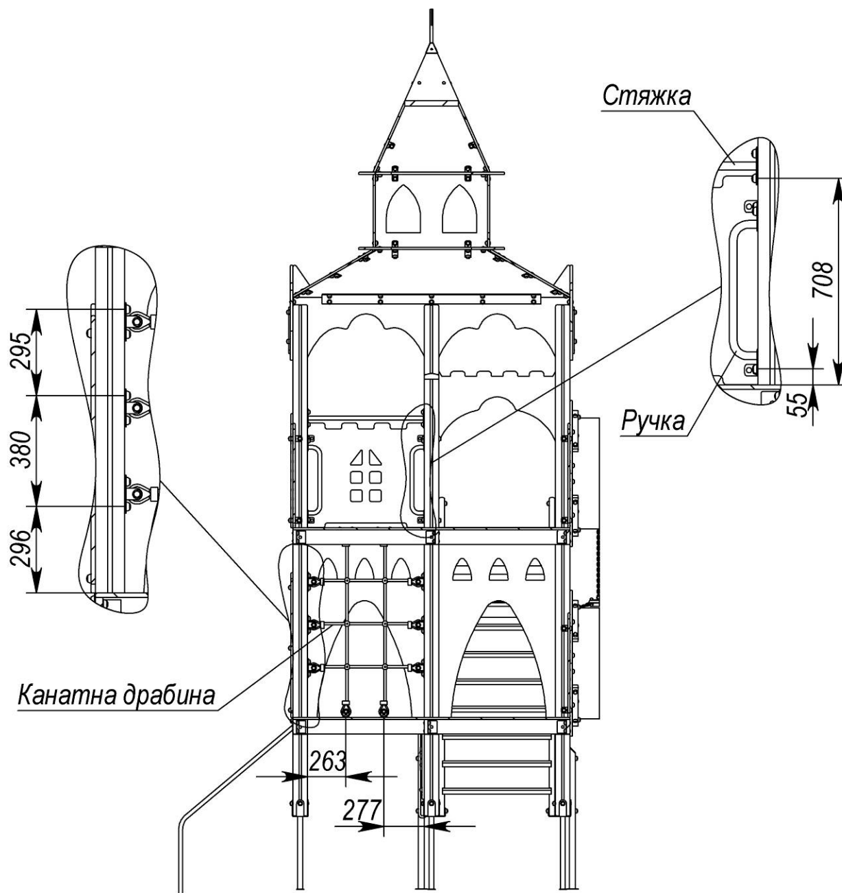
Рисунок 26 – Схема монтажу (Канатної драбини, ручки, стяжки) до вежі подвійної (1,9х1,9м) брус 3,5м
