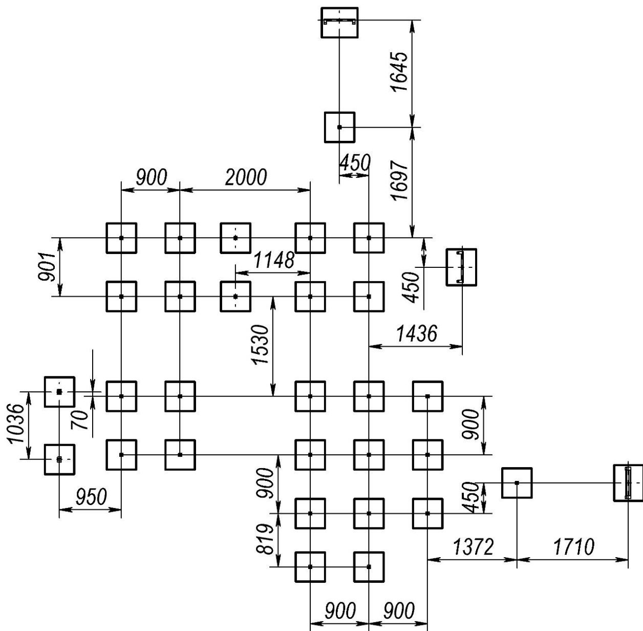
Рисунок 2 – Схема бетонування
