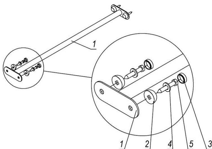
Рисунок 14 – Схема монтажу сходів похилих
