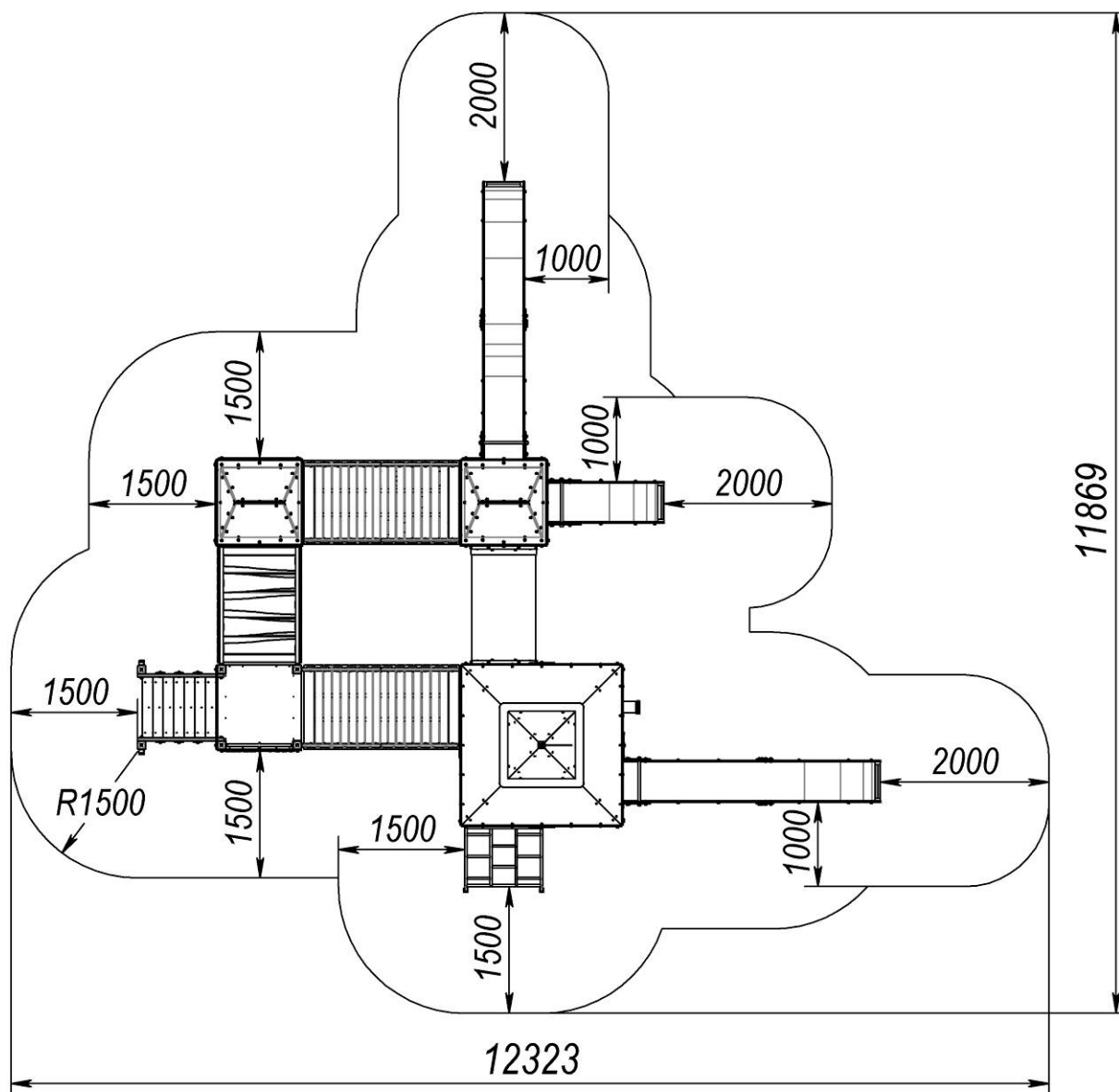
Рисунок 1 – Площа для монтажу та зона безпеки
