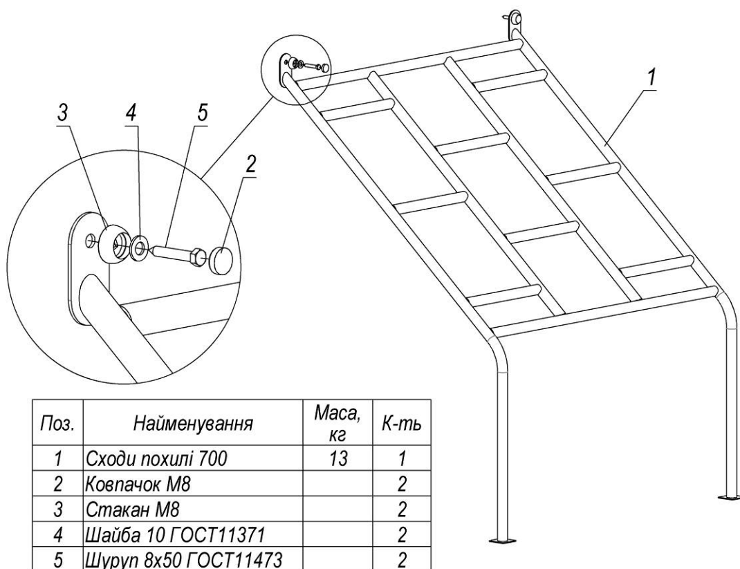
Рисунок 14 – Схема монтажу сходів похилих
