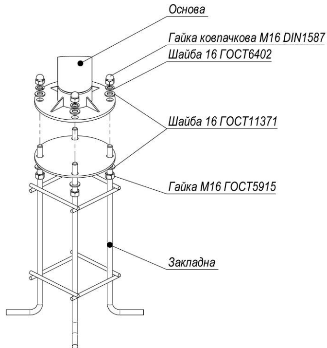
Рисунок 1 – Схема складання
