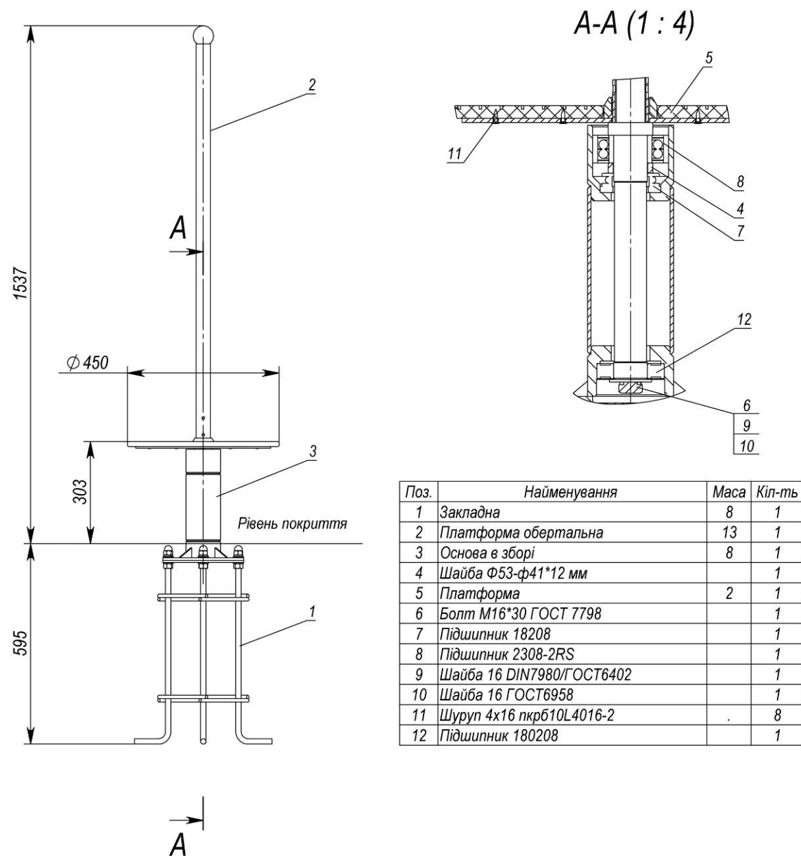
Рисунок 5 - Спінер L
