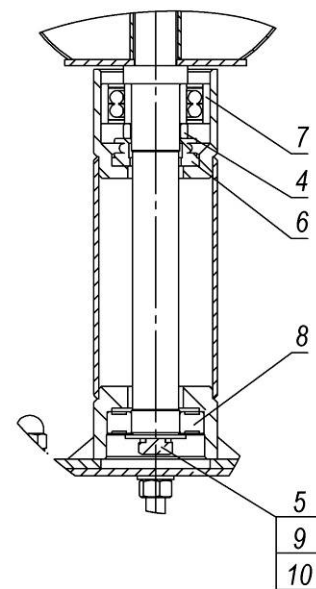
A-A (1 : 5)
