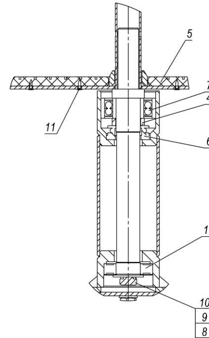
A-A (1 : 4)
