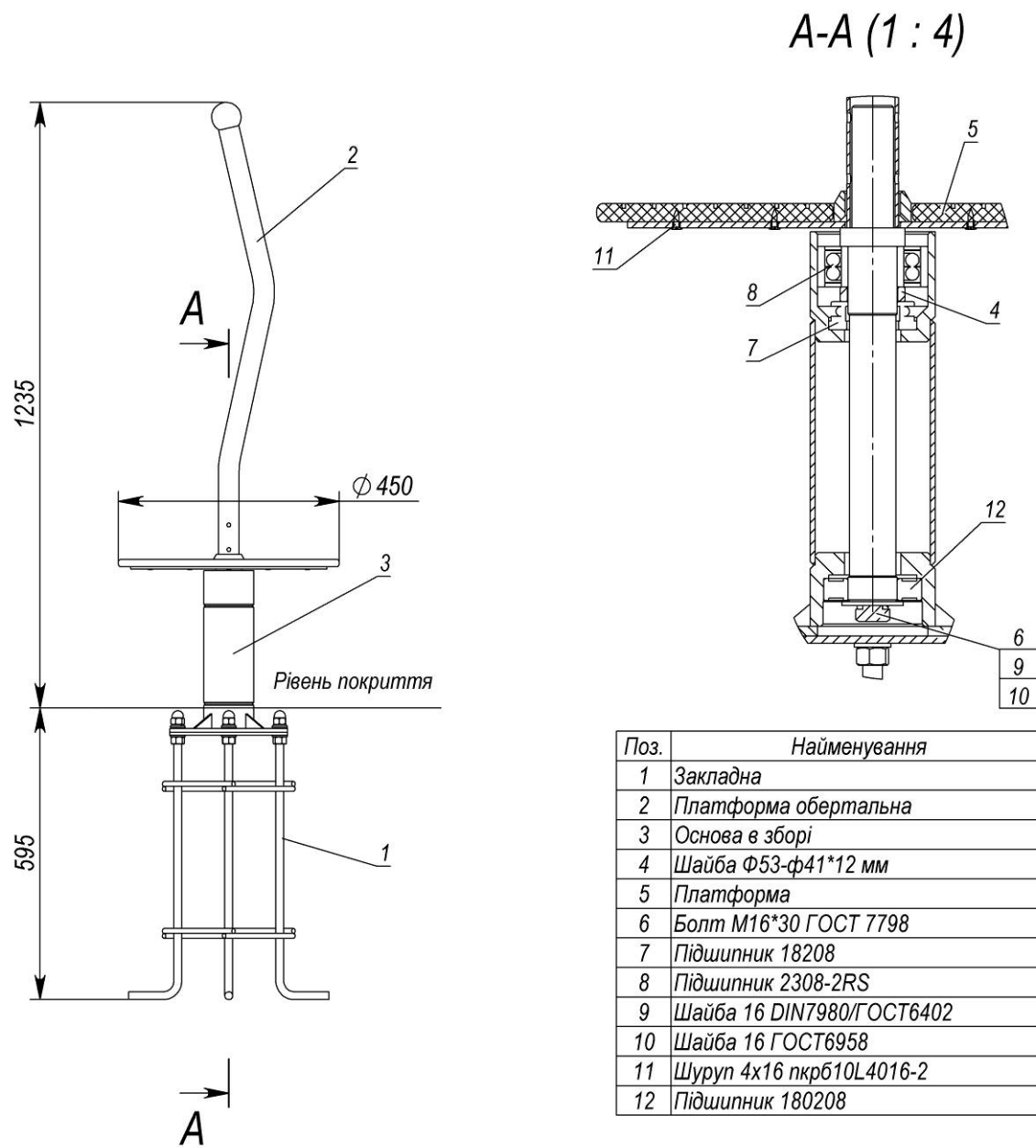
Рисунок 6 - Спінер SC
