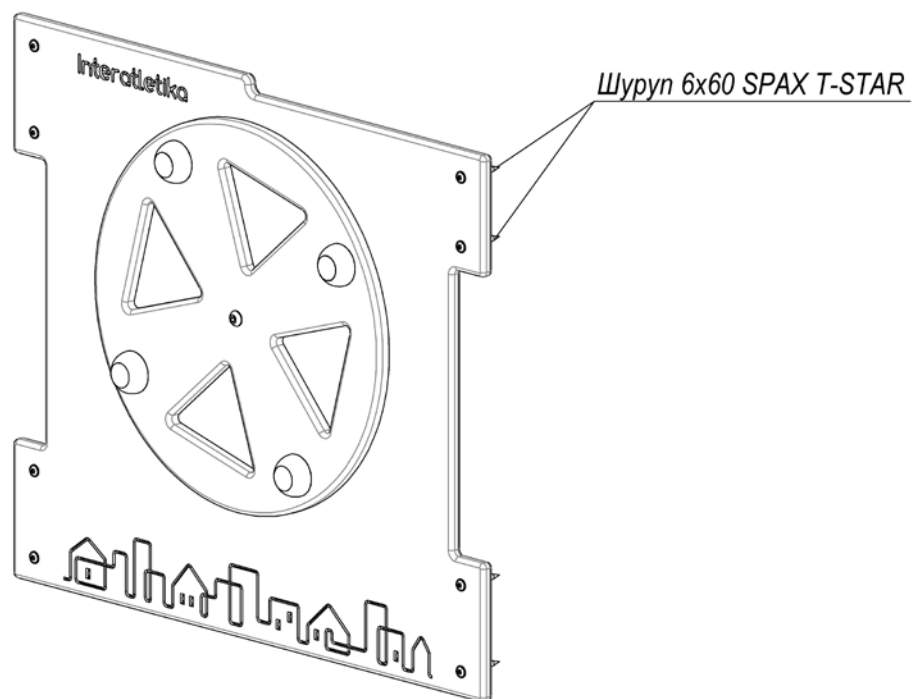
Рисунок 7 – Схема складання панелей ( Складання інших панелей ідентичне)
