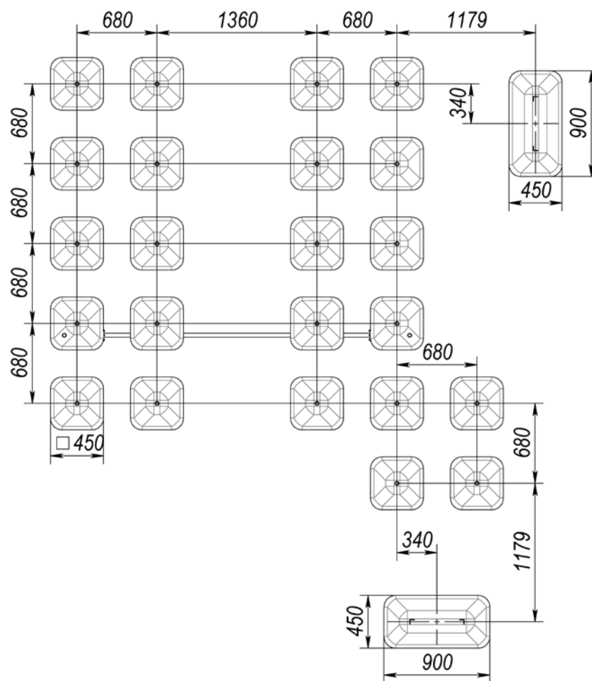
Рисунок 2 – Схема розташування фундаментів
