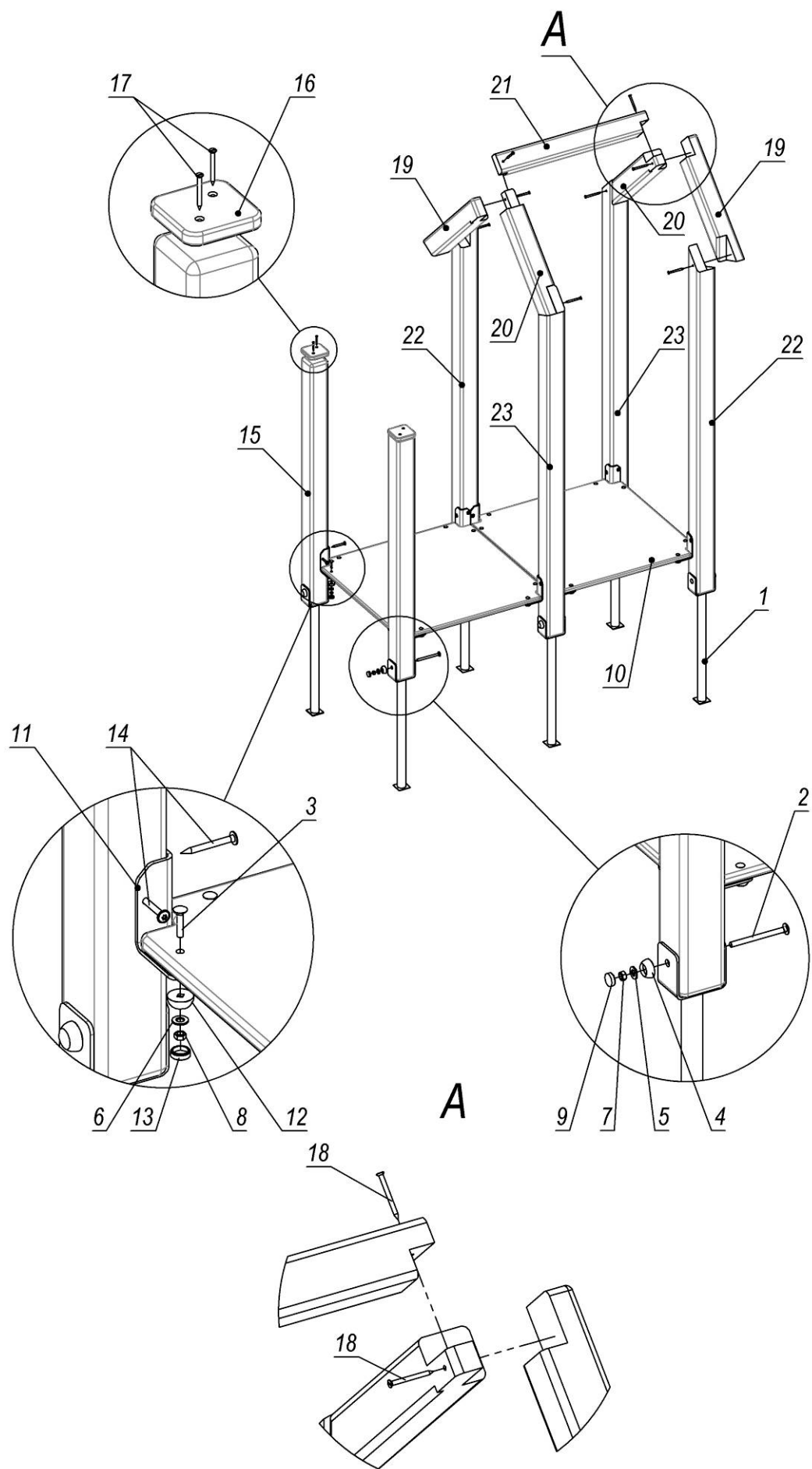
Рисунок 3 – Схема складання будиночка 0,76x1,44
