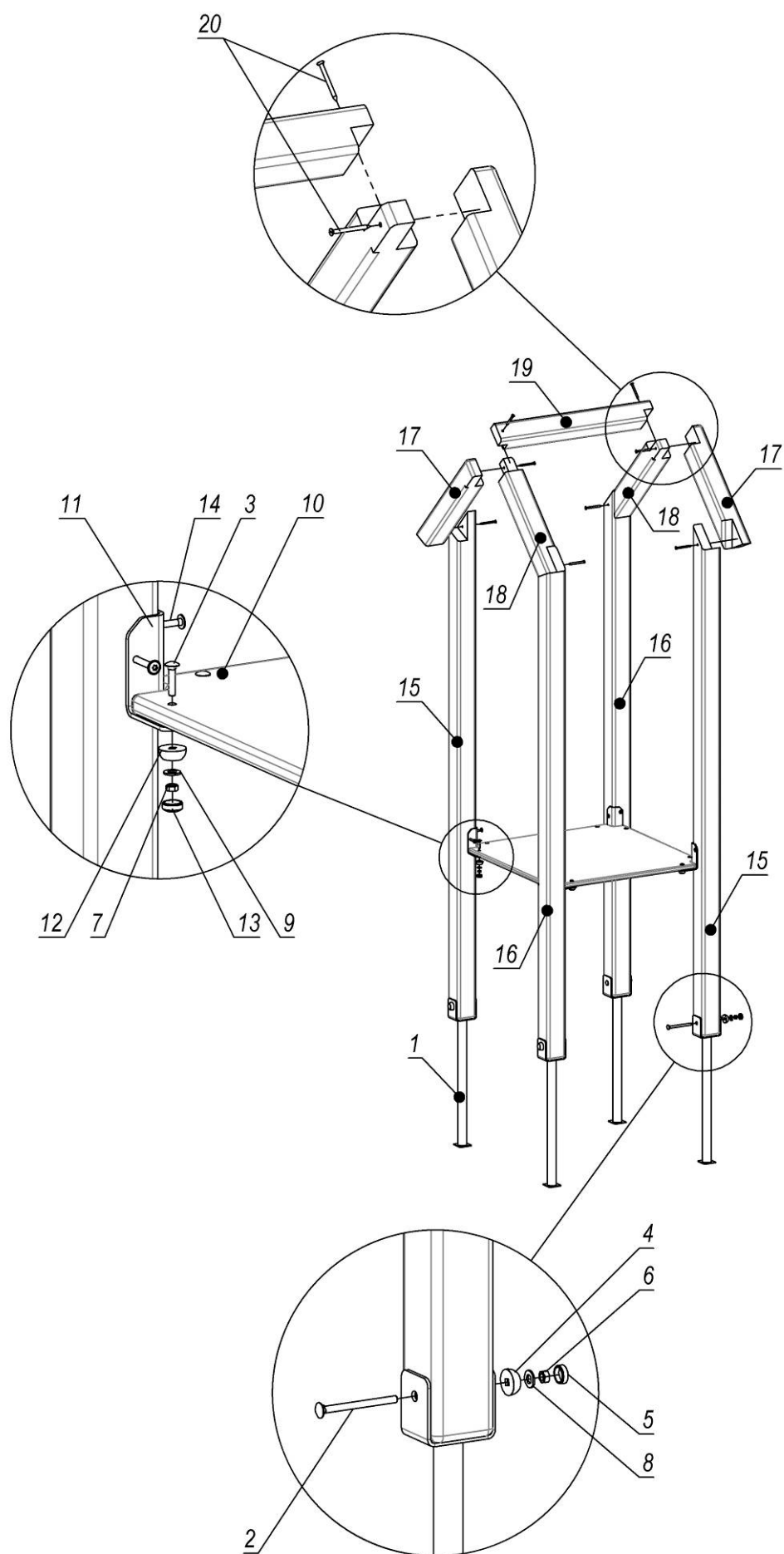
Рисунок 4 – Схема складання вежі
