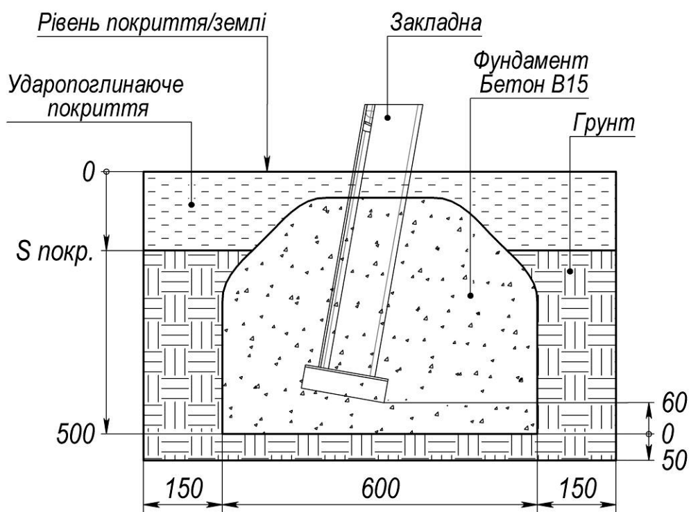
Рисунок 3 – Схема бетонування
