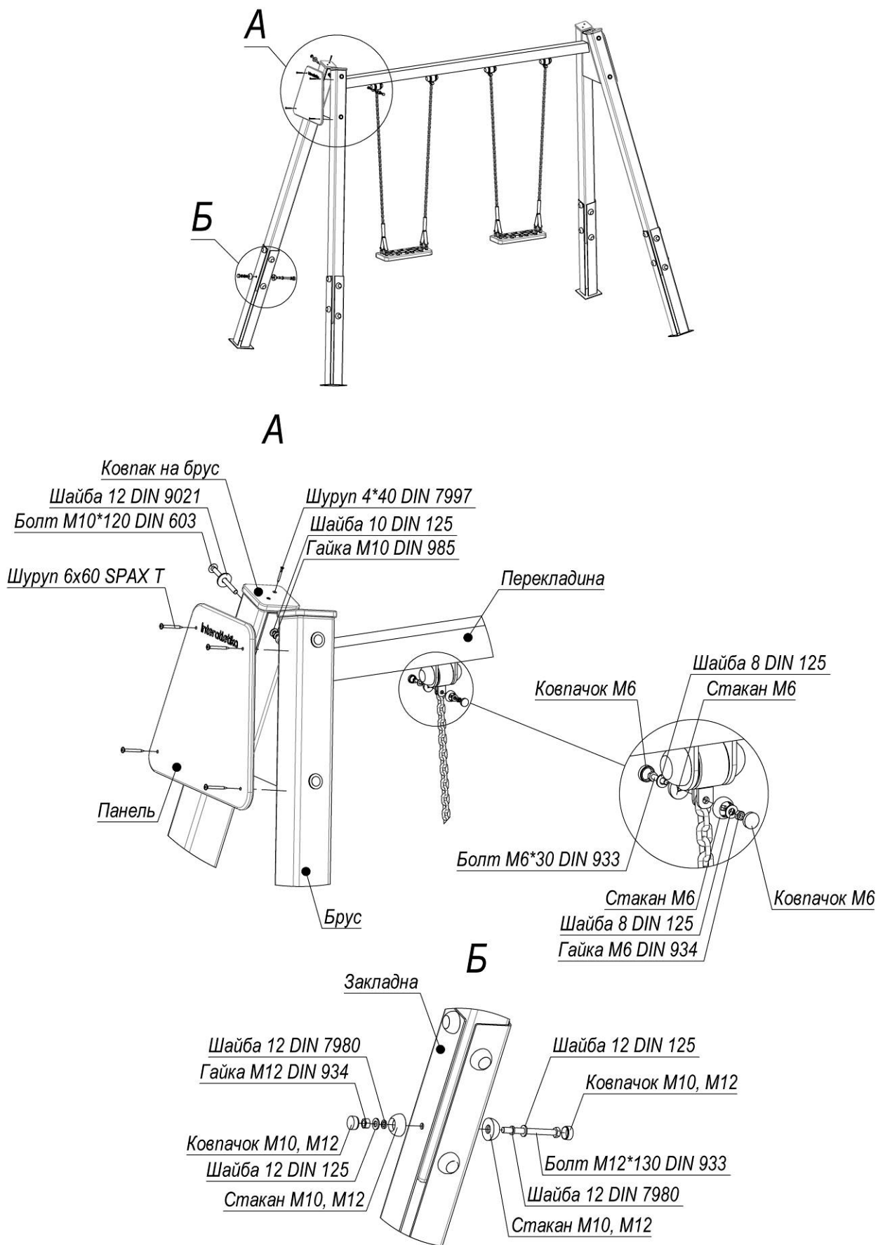
Рисунок 1 – Схема складання гойдалки
