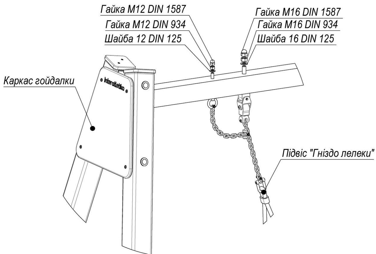
Рисунок 2 – Схема закріплення «Гнізда лелеки»
