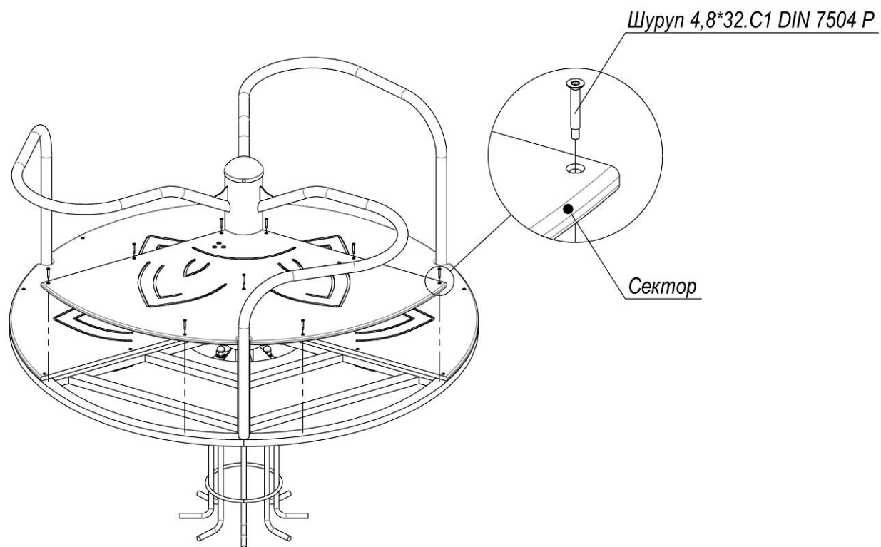
Рисунок 4 – Схема складання сектора для LK481, LK481-S, LK481.1, LK481.1-S, LK483, LK483.1, LK485, LK485.1, LK486, LK486.1, LK487, LK487.1
