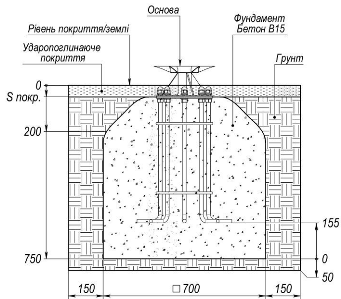
Рисунок 5 - Схема бетонування
