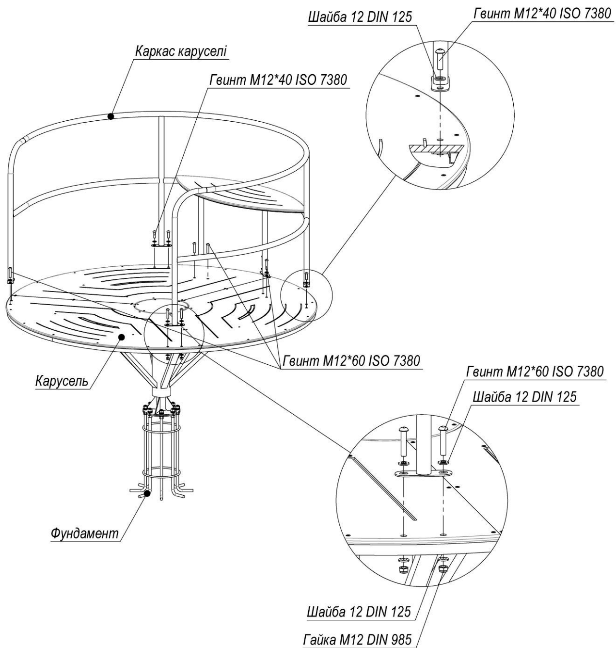
Рисунок 1 – Схема складання каркаса каруселі LK484, LK484.1
