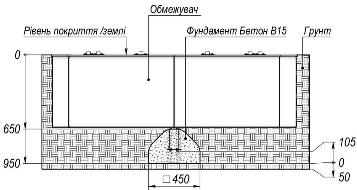
Рисунок 6 - Схема бетонування для LK484, LK484.1, LK488, LK488.1
