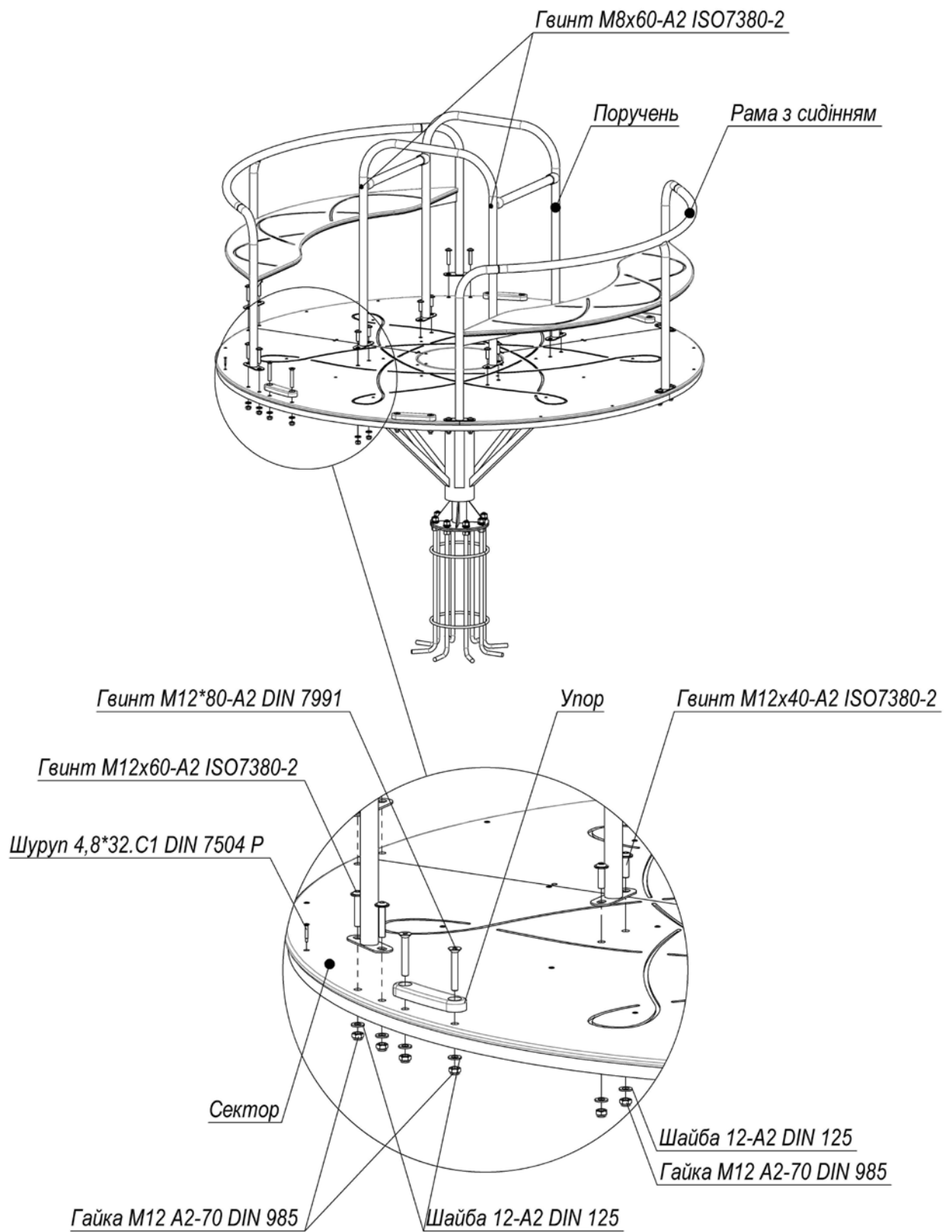
Рисунок 2 – Схема складання каруселі LK488, LK488.1
