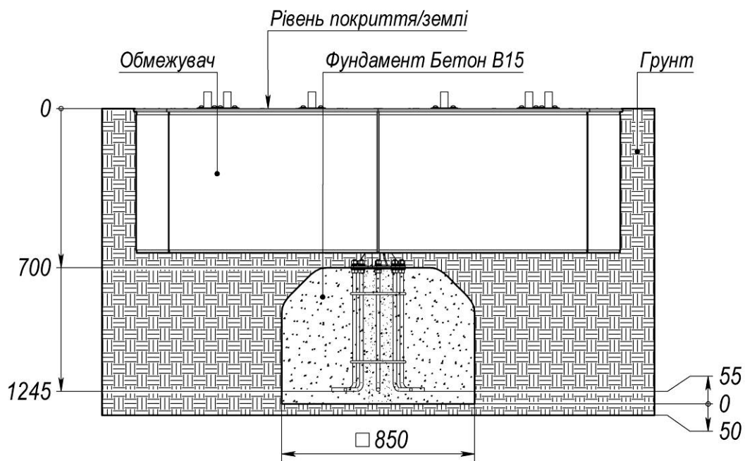
Рисунок 5 - Схема бетонування
