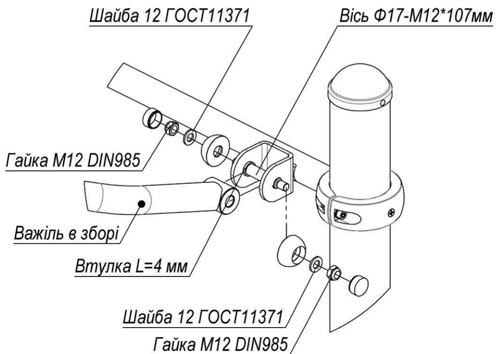
Рисунок 12 – Встановлюємо важіль
