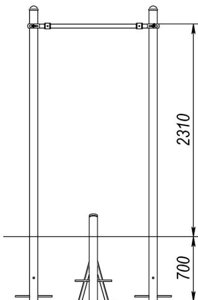
Рисунок 11 – Закріплюємо стійку з зв'язком
