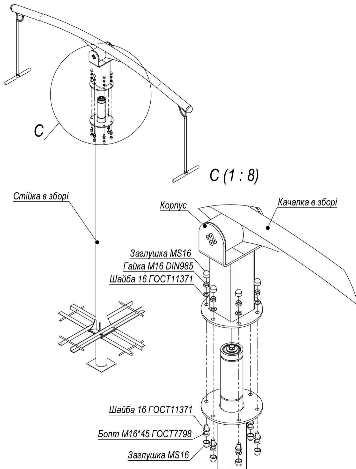
Рисунок 9 – Закріплюємо качалку з корпусом до стійки для TE224
