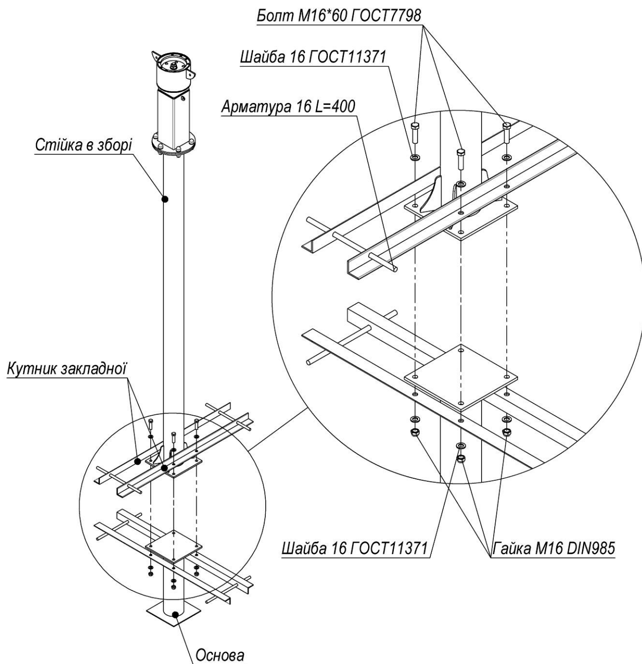
Рисунок 1 – Закріплюємо між собою стійку і основу
