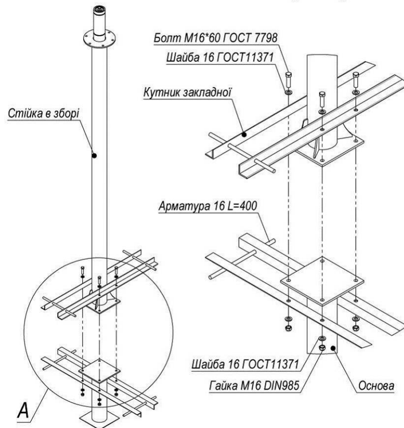
Рисунок 7 – Закріплюємо між собою стійку і основу
