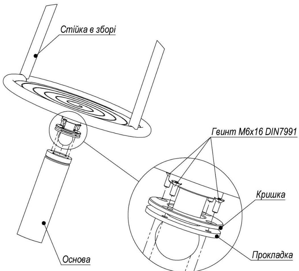
Рисунок 13 – Схема з'єднання стійки з основою
