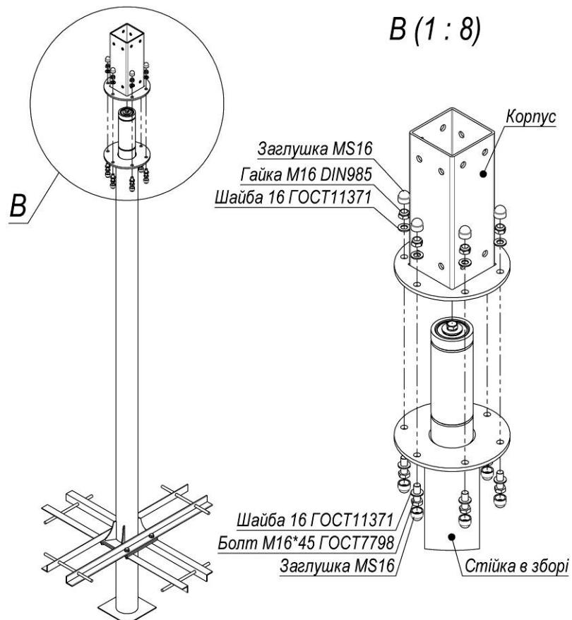
Рисунок 8 – Встановлюємо корпус до стійки для ТЕ225
