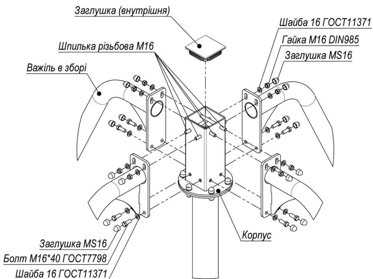
Рисунок 6 – Закріплюємо важелі до корпусу
