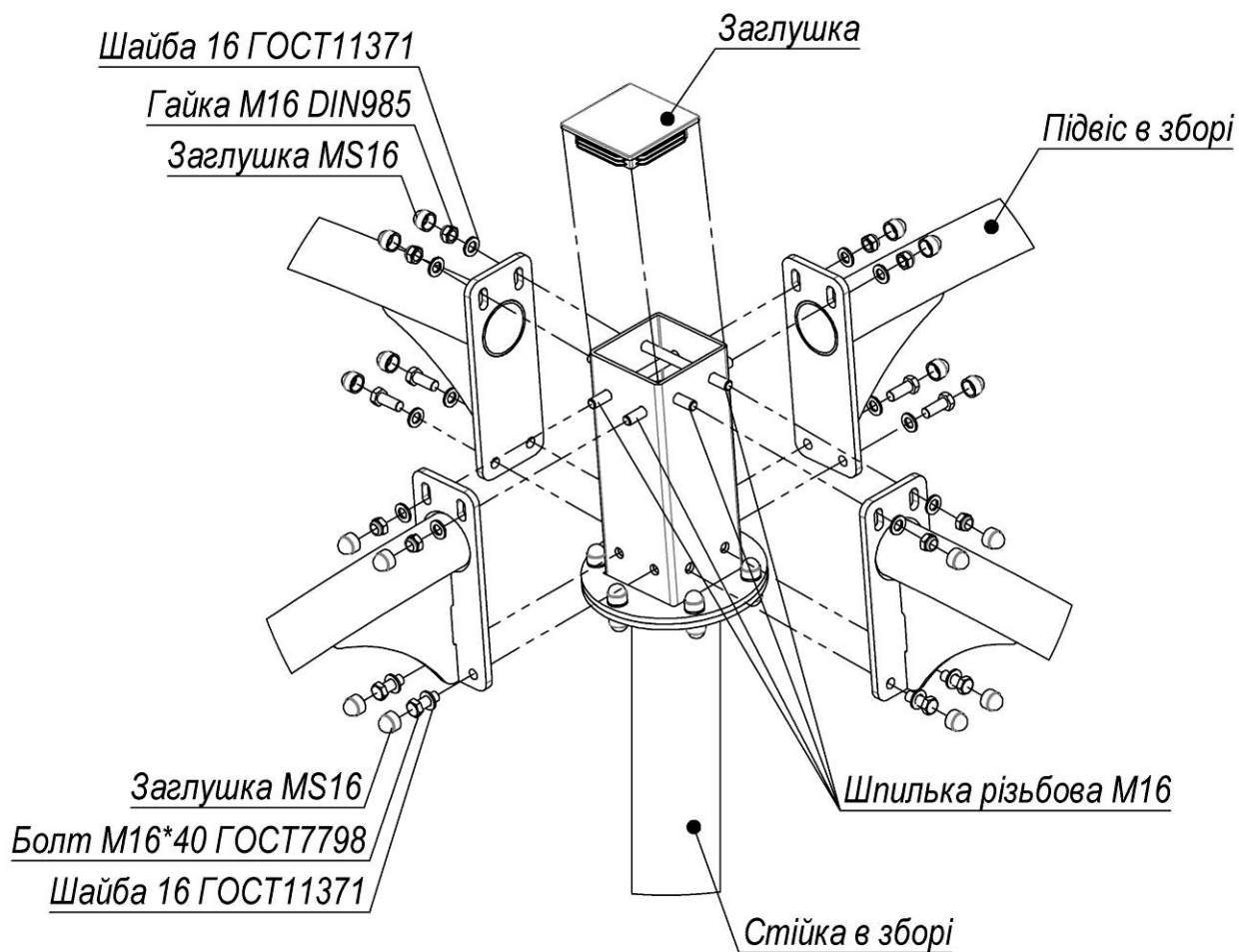
Рисунок 10 – З'єднуємо підвіси з корпусом для TE225
