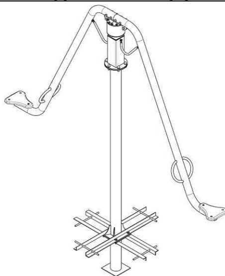
TE223 Карусель-балансир (2 місця)
