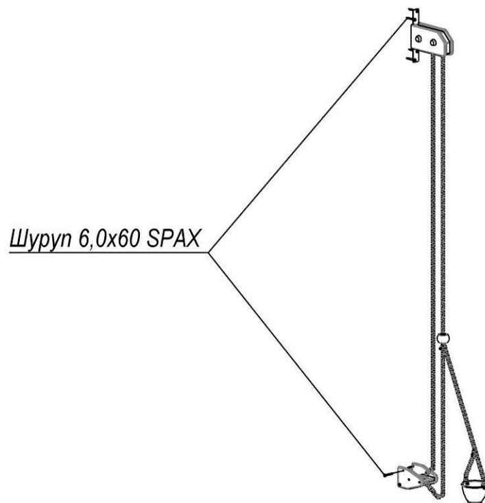
Рисунок 6 – Схема з'єднання відра на ланцюгах
