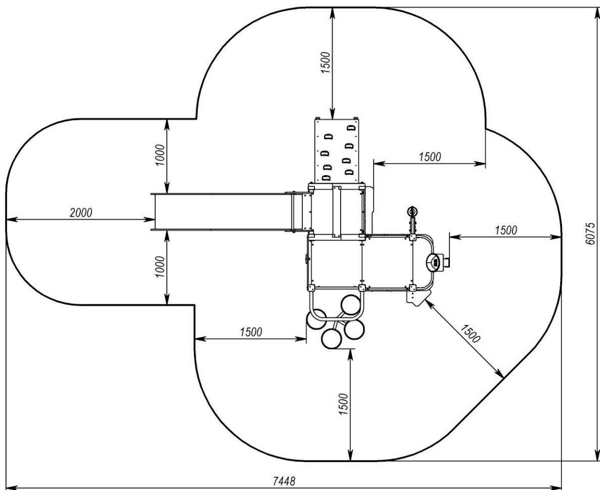
Рисунок 1 -Площа для монтажу та зона приземлення
