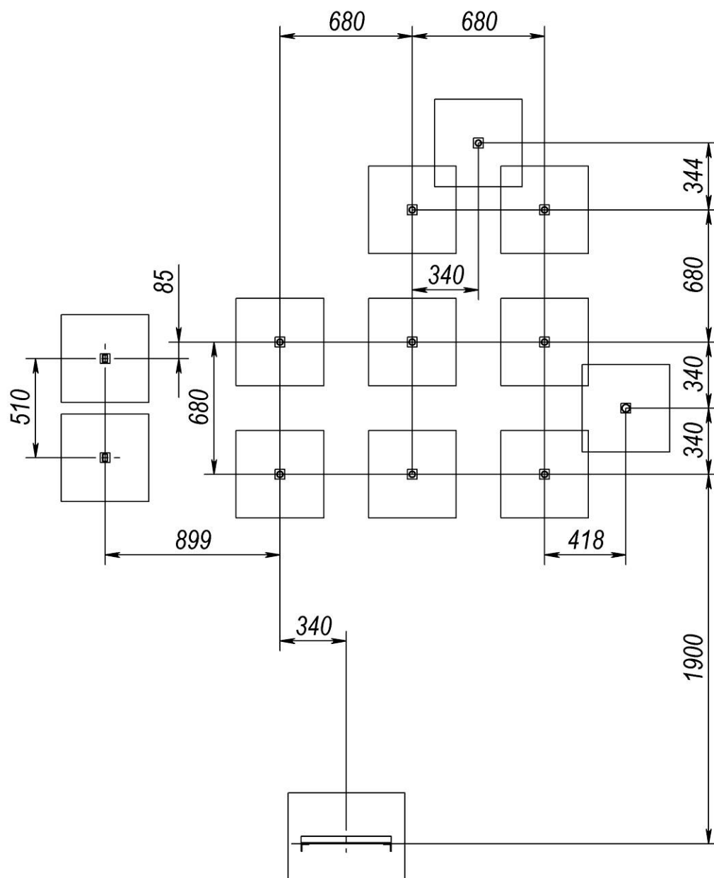
Рисунок 2 – Схема розташування фундаментів
