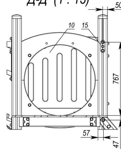
Д-Д (1 : 15)
