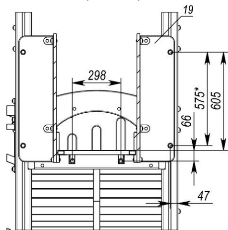
Г-Г (1 : 15)
