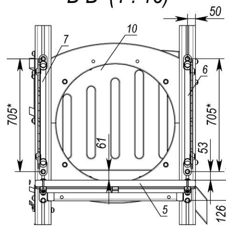
Б-Б (1 : 15)
