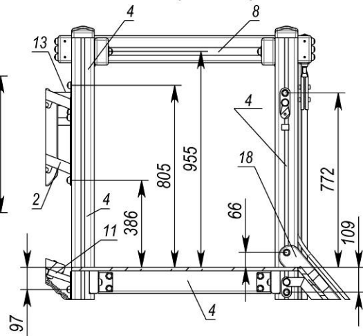
В-В (1 : 15)
