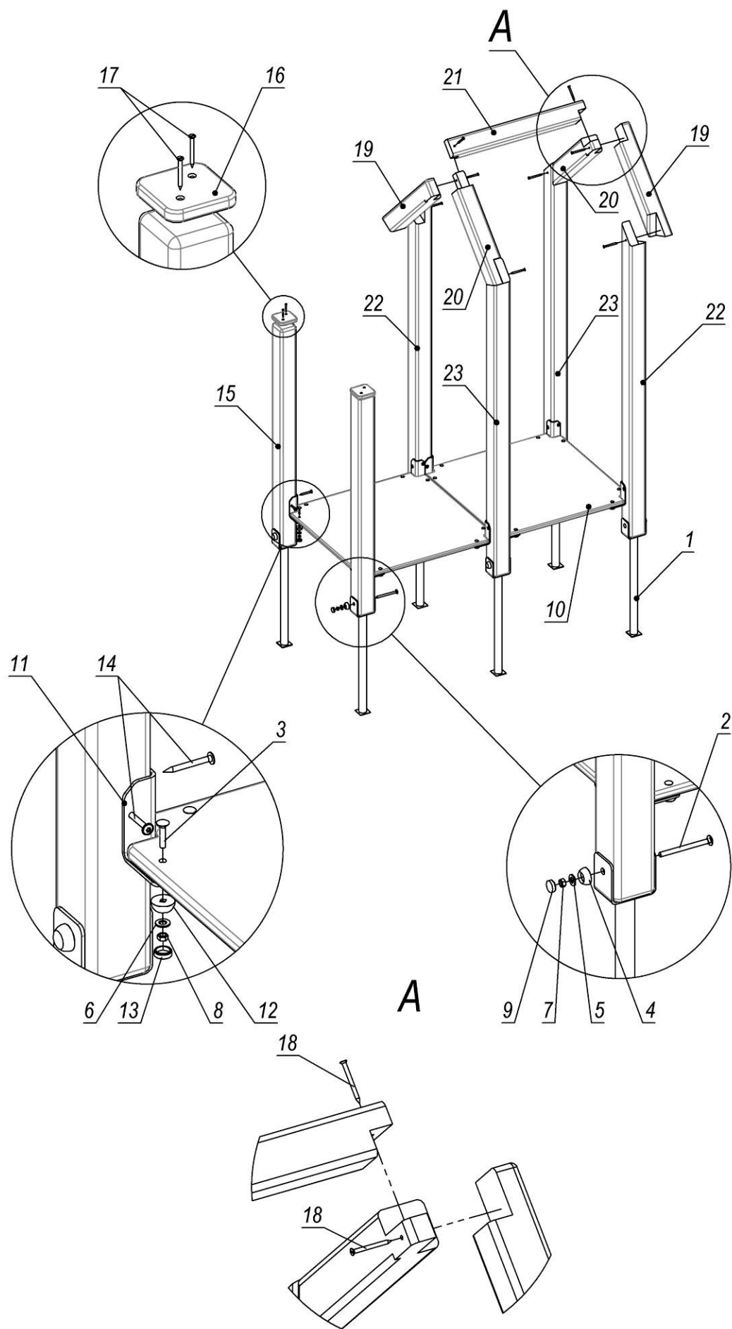
Рисунок 4 – Схема складання будиночка 0,76x1,44
