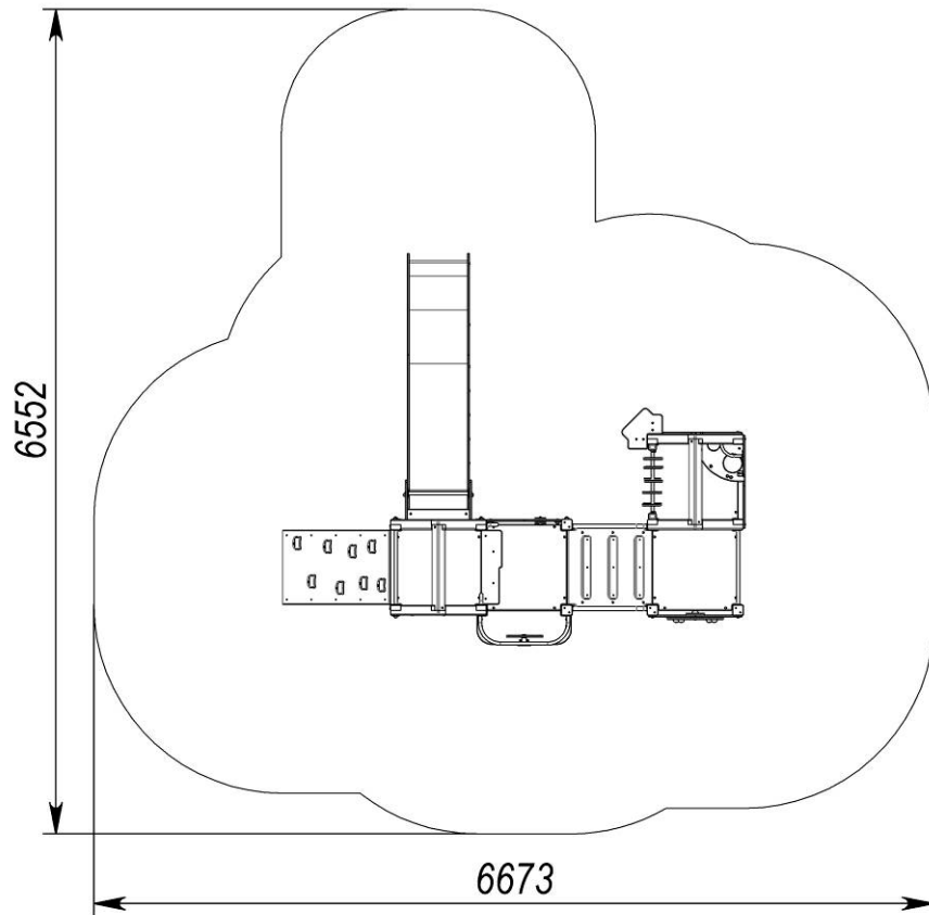
Рисунок 1 -Площа для монтажу та зона приземлення
