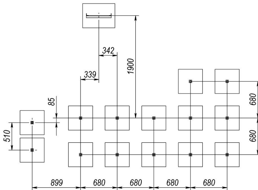
Рисунок 2 – Схема розташування фундаментів
