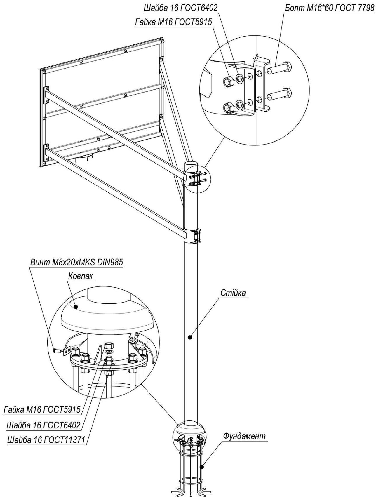
Рисунок 4 – Схема монтажу 2
