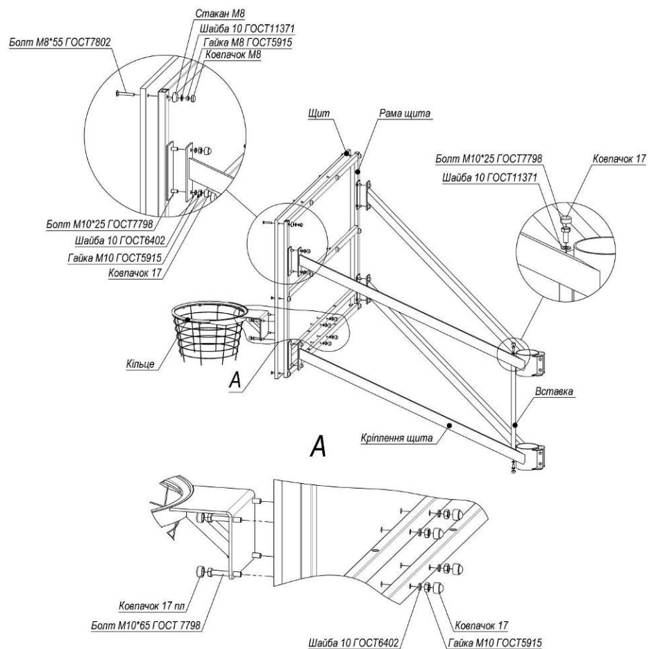
Рисунок 2 – Схема монтажу 1
