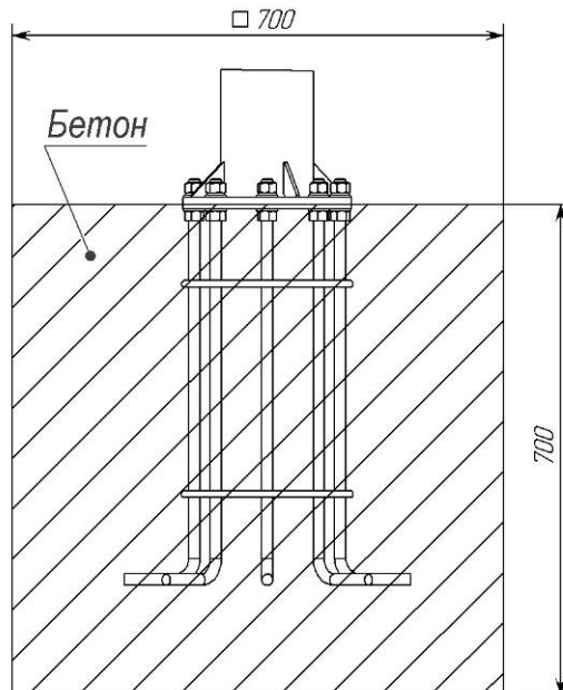
Рисунок 5 – Схема Бетонування
