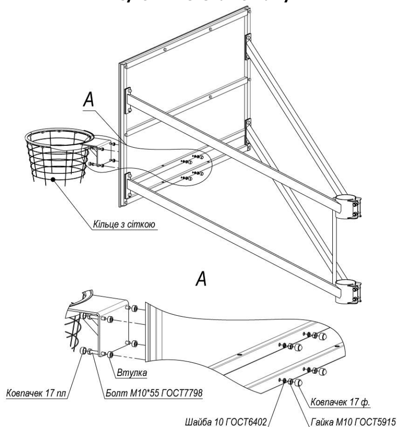
Рисунок 2 – Схема монтажу 1
