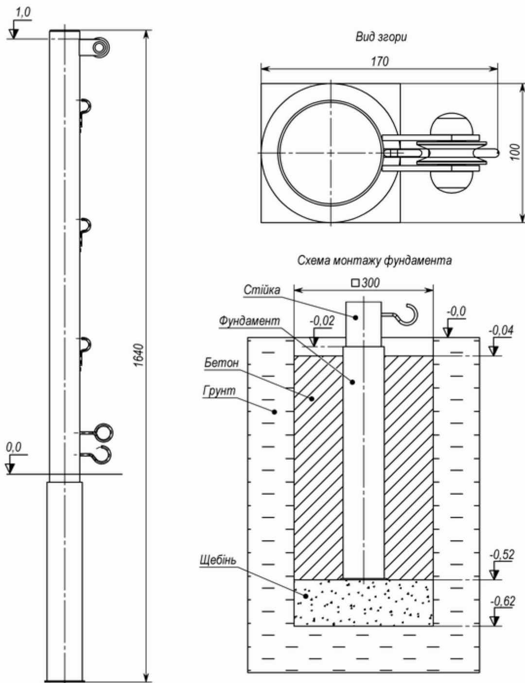
МАЛЮНОК 2 «Габаритні розміри виробу та схема монтажу»
