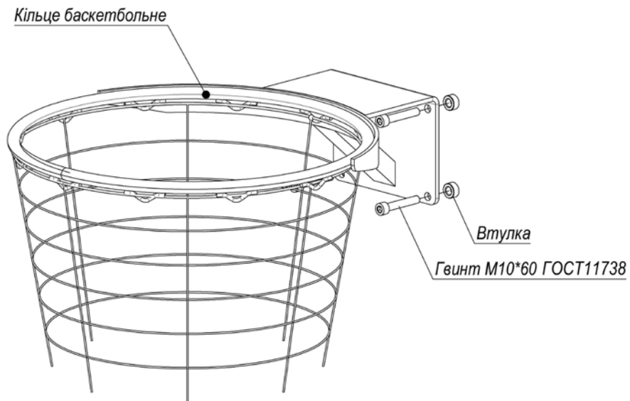
Рисунок 5 – Кріплення кільця баскетбольного під щит акриловий (для УТ408-01)
