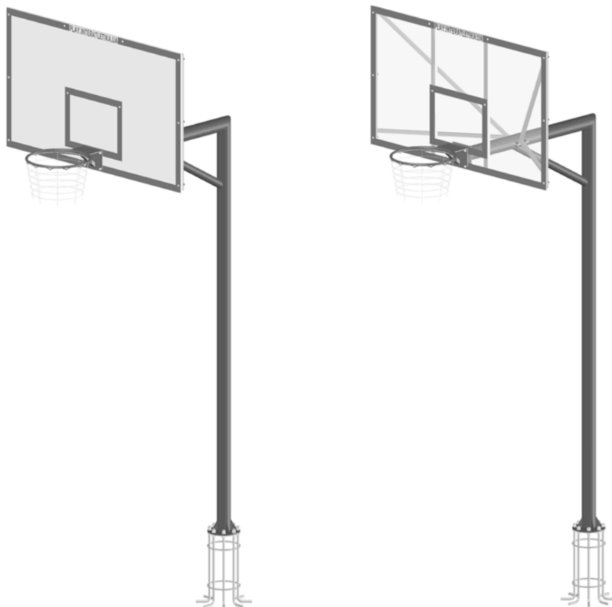
Рисунок 1 – Загальний вигляд
