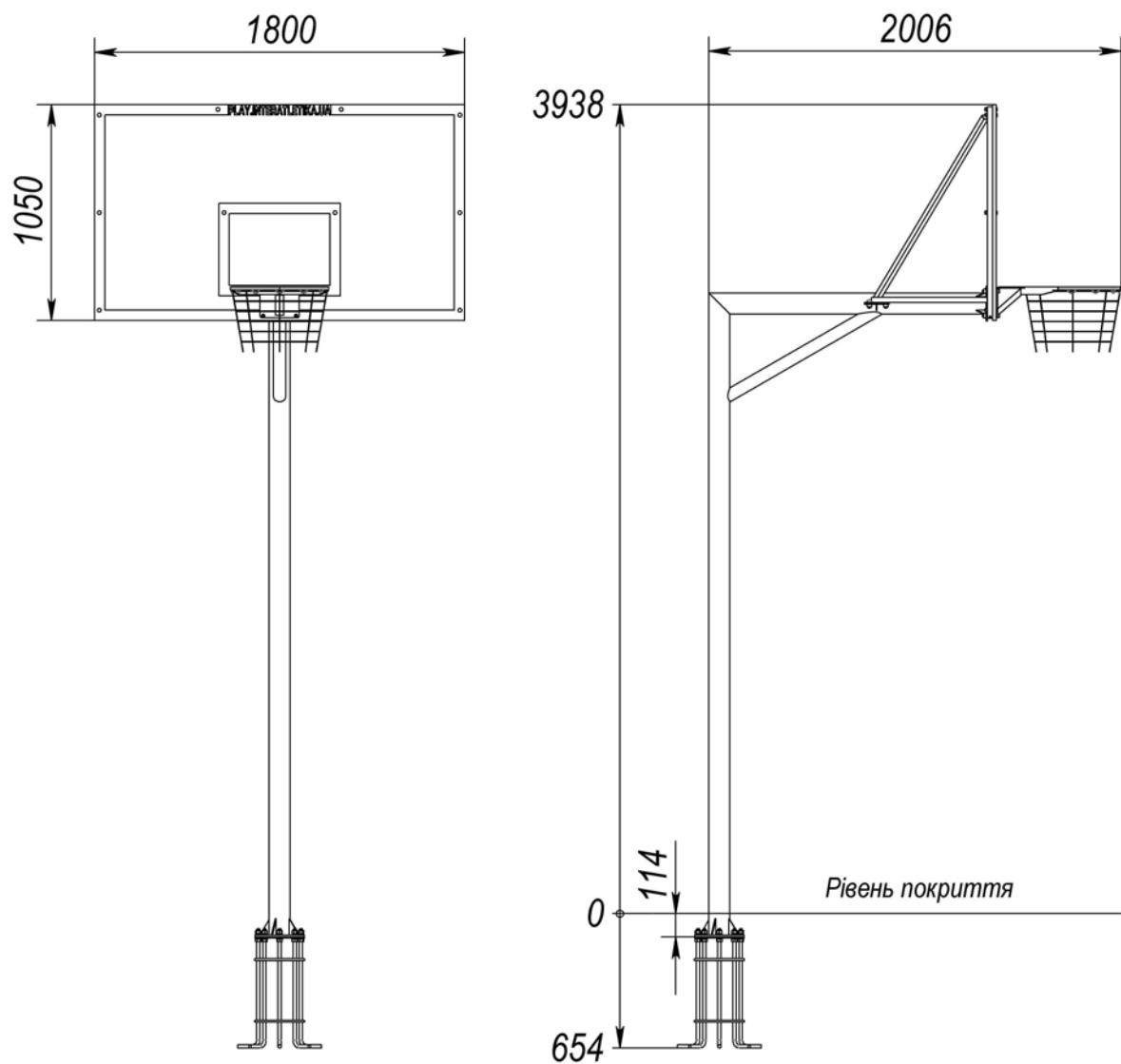
Рисунок 2 – Габаритні розміри
