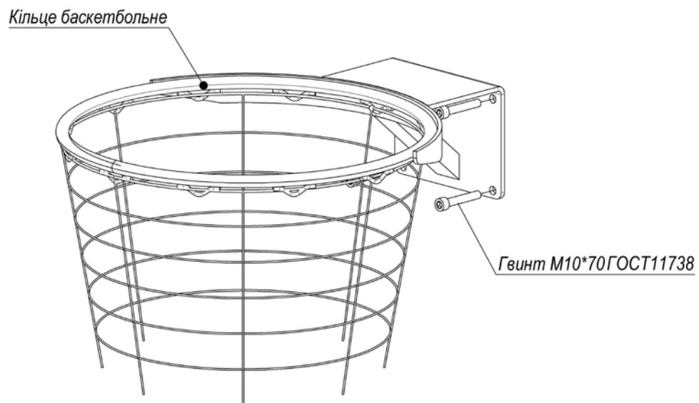
Рисунок 6 – Кріплення кільця баскетбольного під щит фанерний (для УТ408.1-01)
