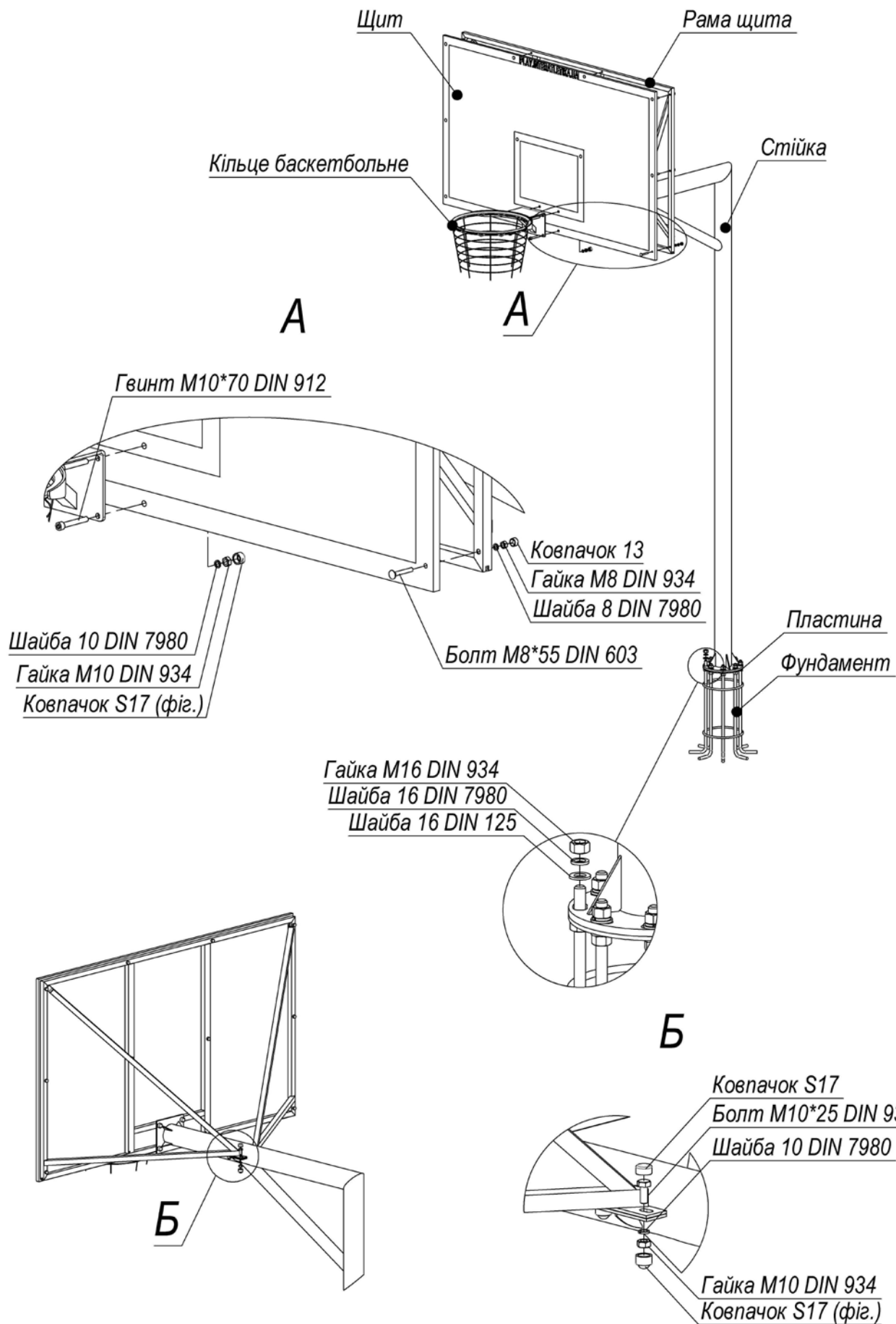
Рисунок 4 – Схема складання
