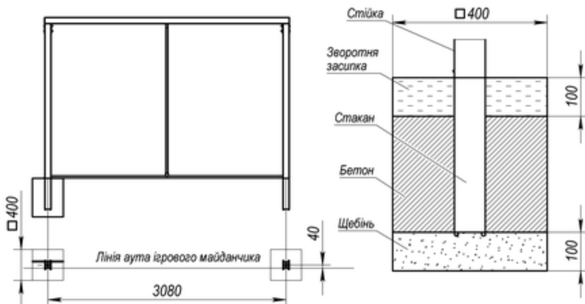
МАЛЮНОК 2 «Габаритні розміри, схема зборки та схема монтажу виробу»
