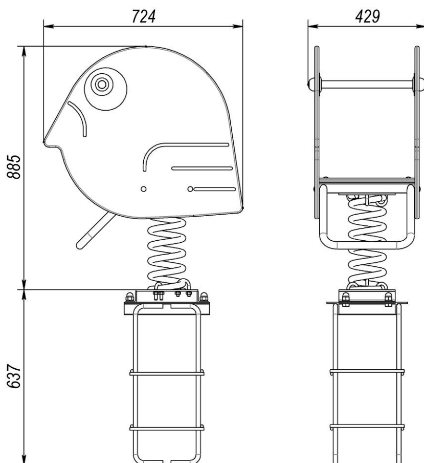
Рисунок 5 - Гойдалка на пружині «Пташка» TE243
