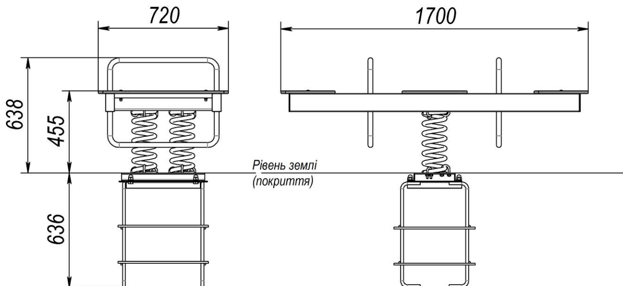
Рисунок 6 - Гойдалка - балансир на пружині TE246
