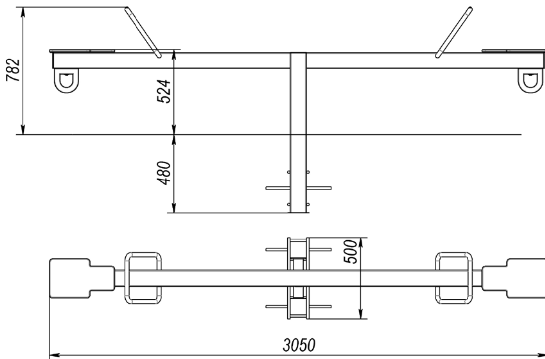
Рисунок 4 - Балансир Місто TE242
