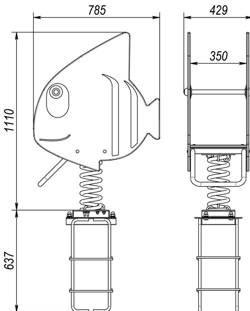
Рисунок 6 - Гойдалка - балансир на пружині TE246
