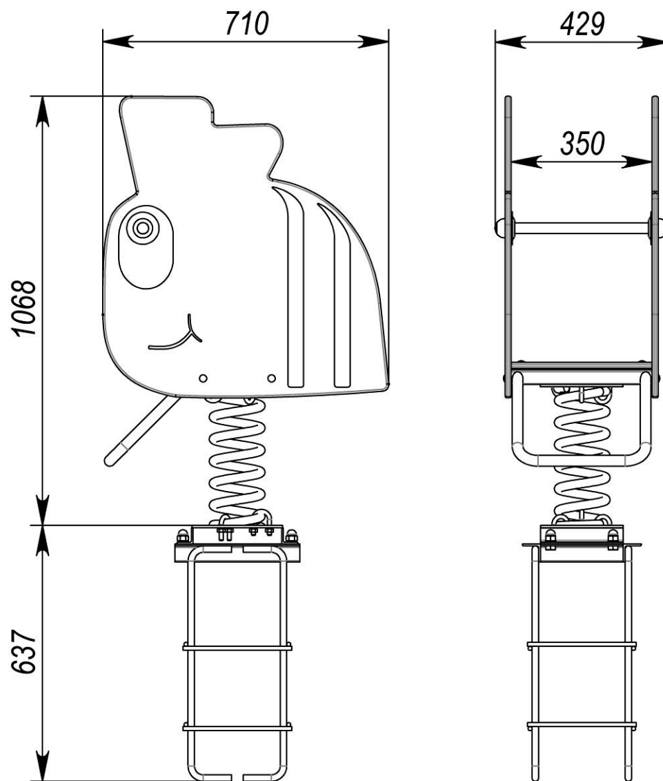
Рисунок 8 – Гойдалка на пружині «Бджілка» TE248
