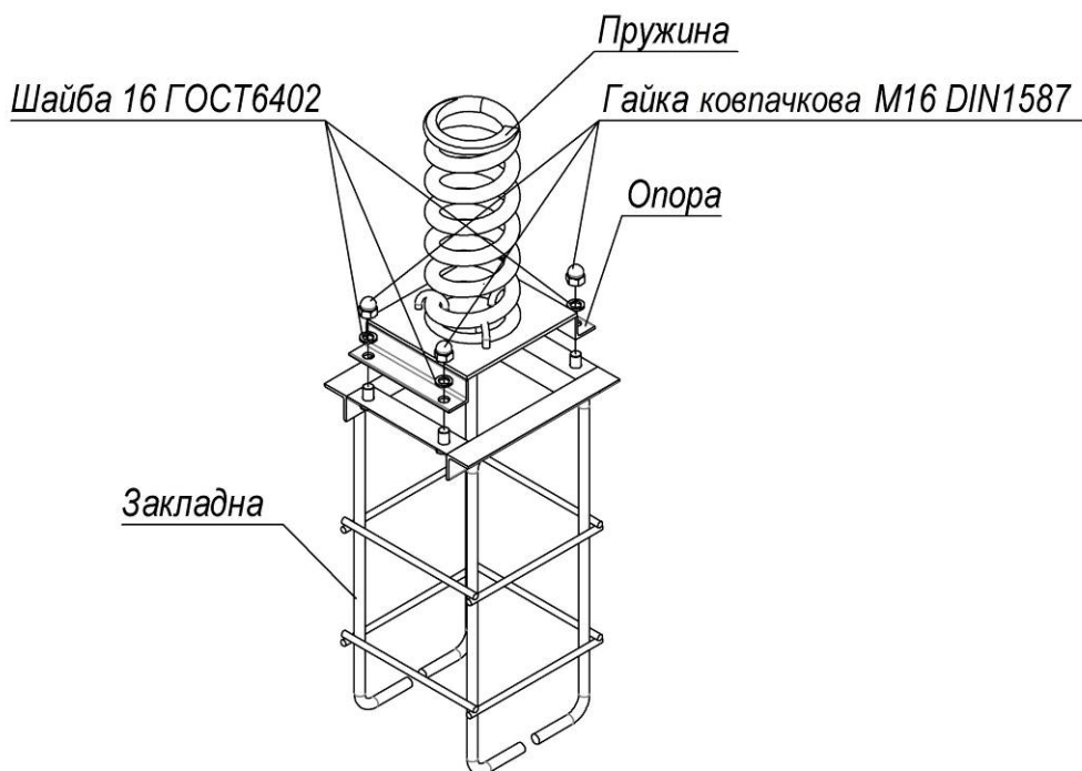
Рисунок 1 - Для ТЕ243, ТЕ247, ТЕ248
