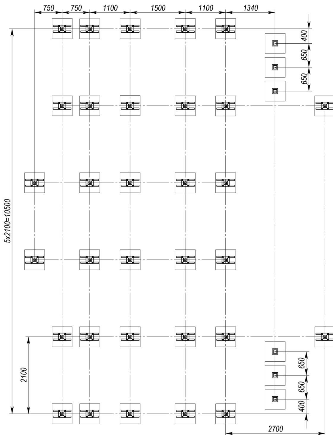
Рисунок 3 – Зона бетонування для УТ131
