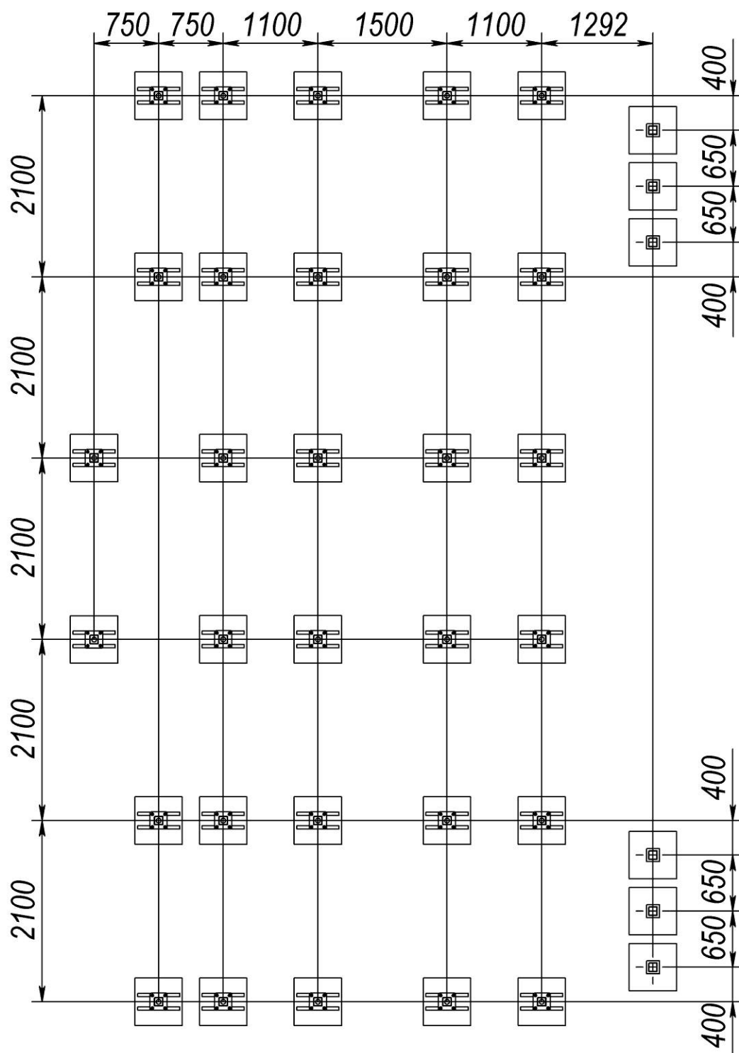
Рисунок 4 – Зона бетонування для УТ131-584
