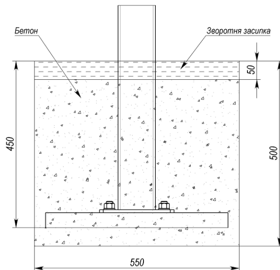
Рисунок 5 – Схема монтажу фундаментів
