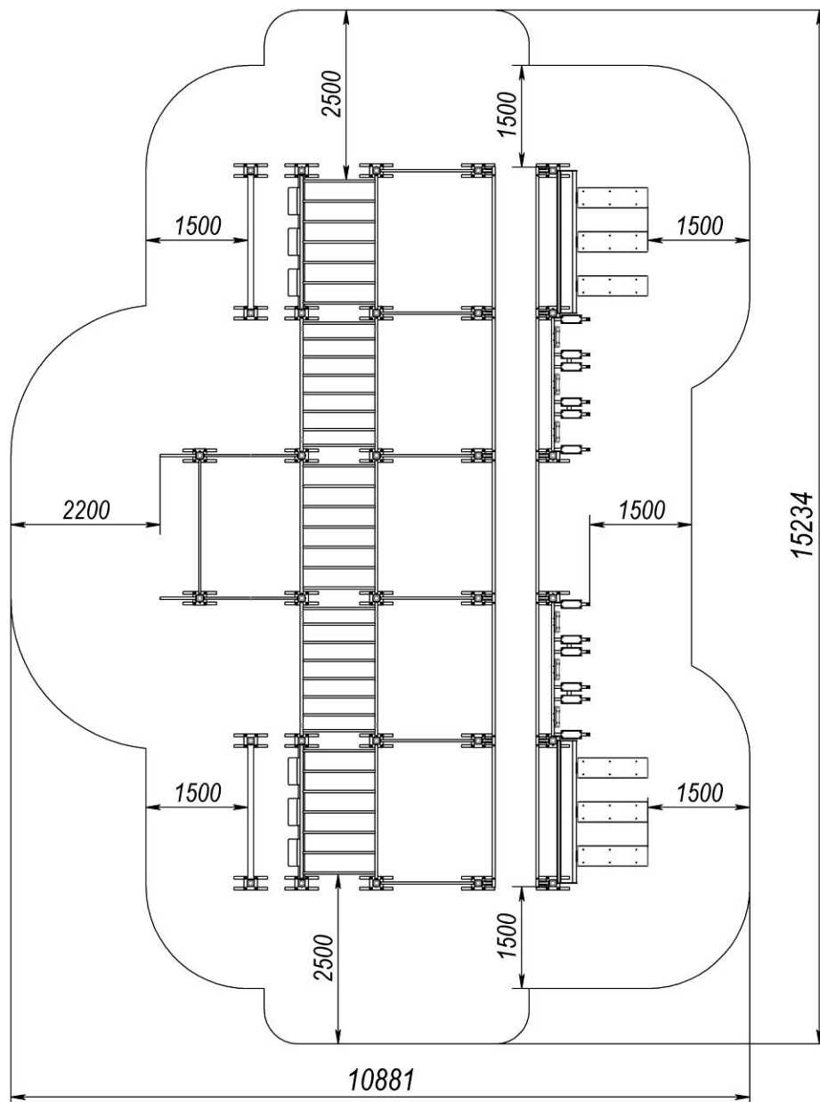
Рисунок 7 – Зона безпеки для УТ131-584
