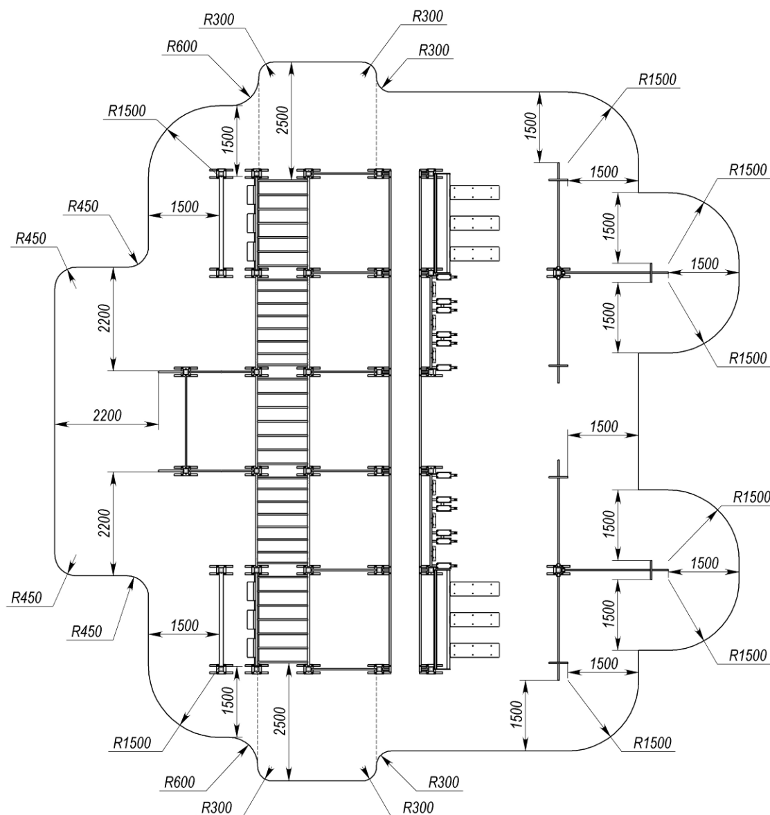
Рисунок 6 – Зона безпеки для УТ131
