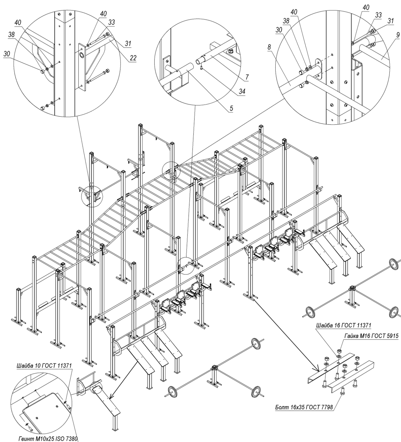
Рисунок 2 – Комплектація та порядок складання
