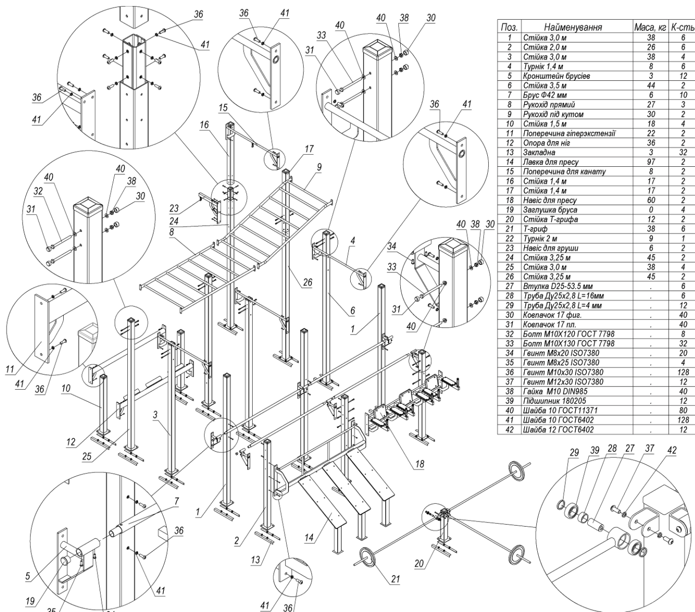
Рисунок 1 – Комплектація та порядок складання
