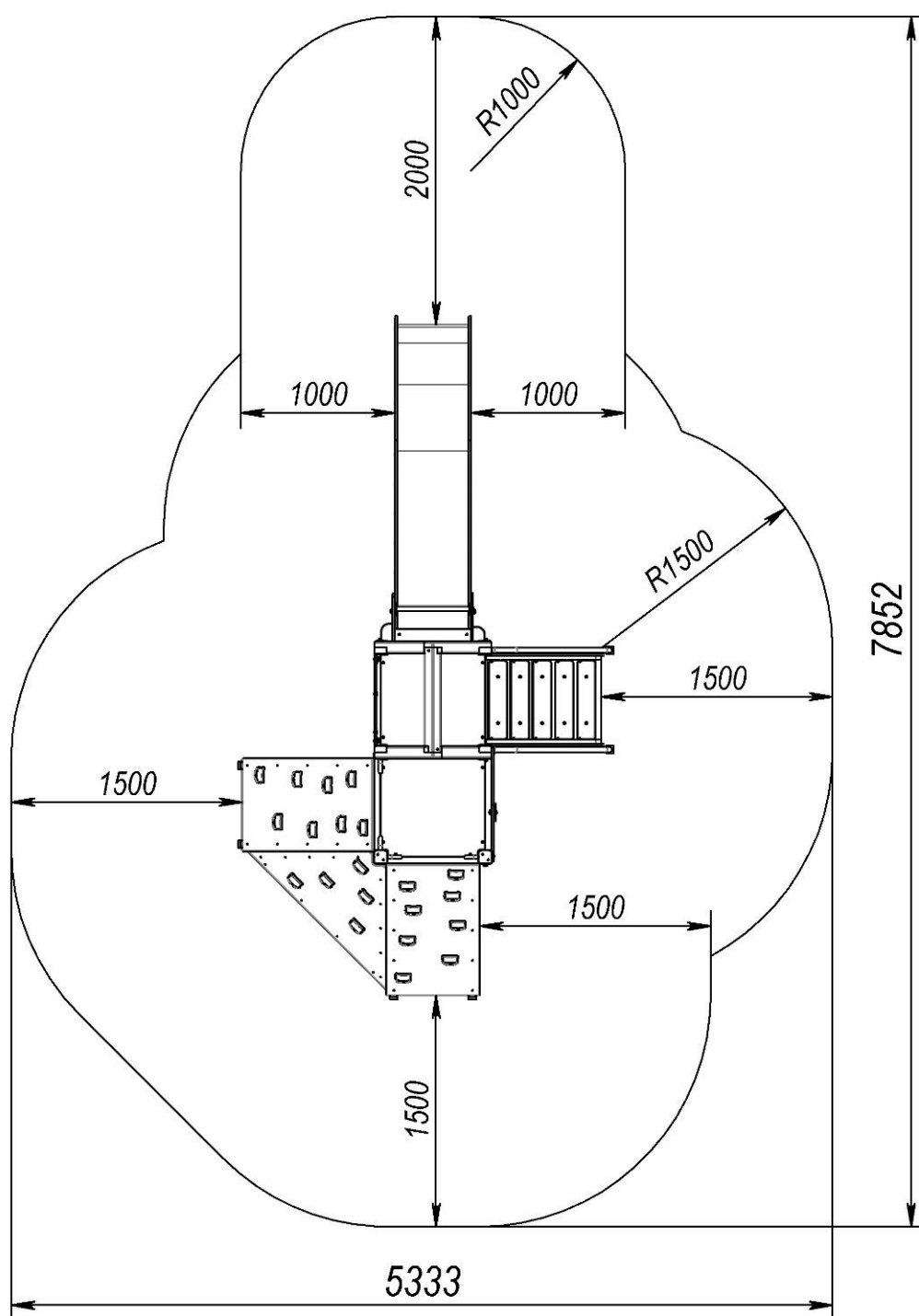
Рисунок 1 -Площа для монтажу та зона приземлення
