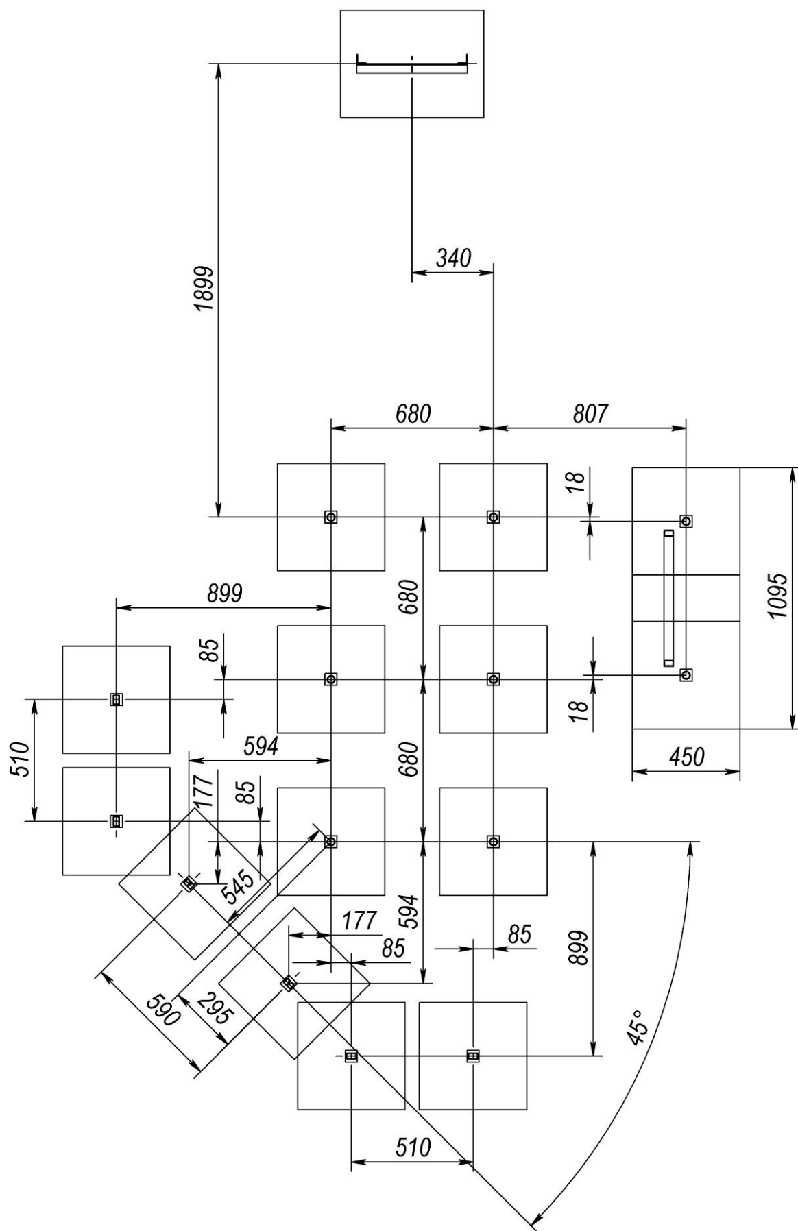
Рисунок 2 – Схема розташування фундаментів
