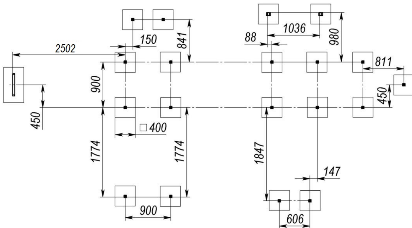
Мал. 19 - Схема розташування фундаментів
