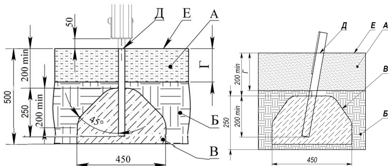
Мал. 19 - Схема розташування фундаментів
