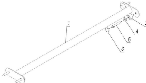
Рисунок 16 - Комплектність та схема складання стяжки з канатом
