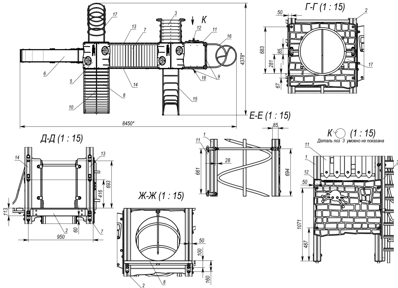
Рисунок 1 - Комплектація та характеристики складових частин виробу
