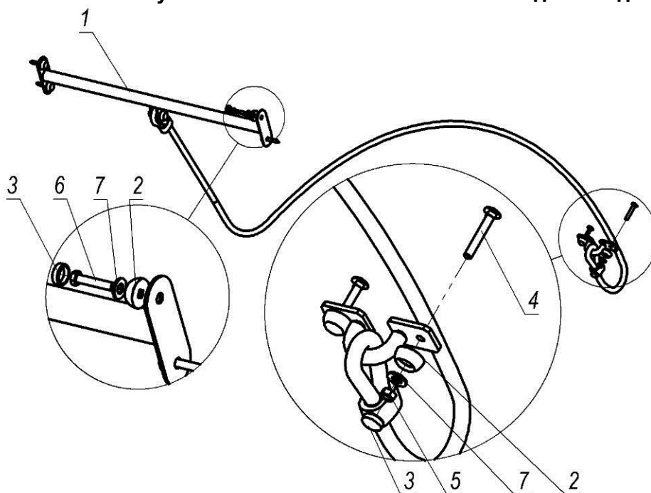
Рисунок 15 - Комплектність та схема складання підйому радіального
