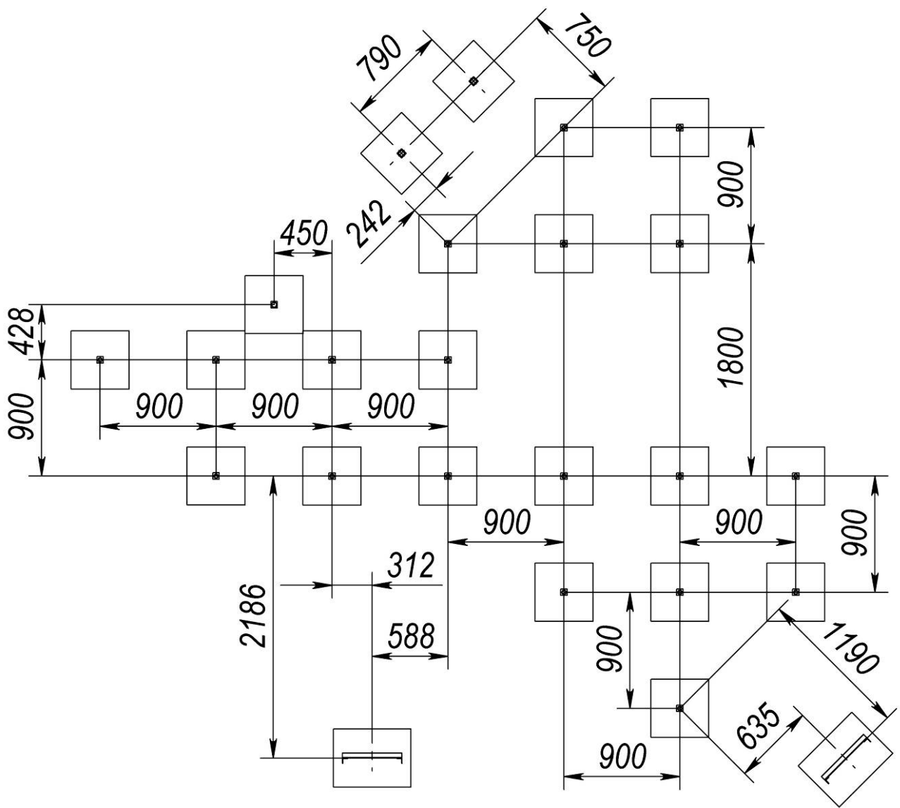
Рисунок 2 – Схема розташування фундаментів
