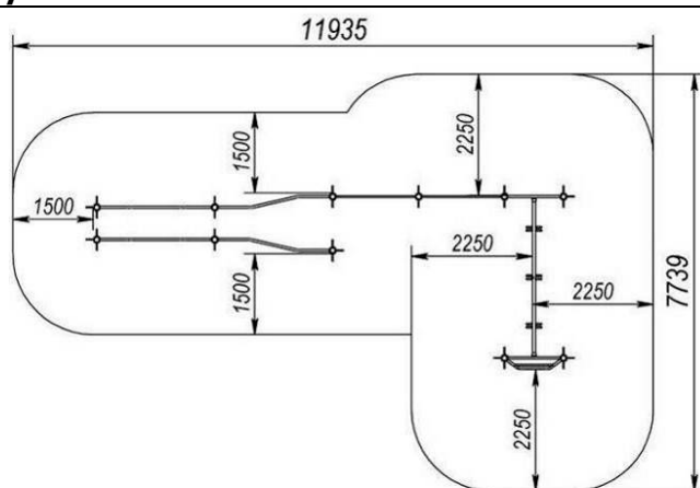
Варіант монтажу №1
