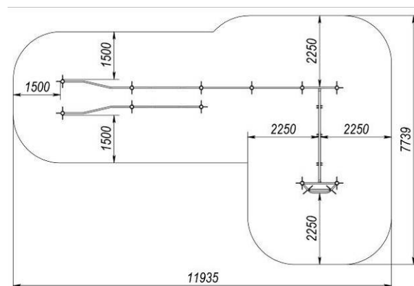
Варіант монтажу №2
