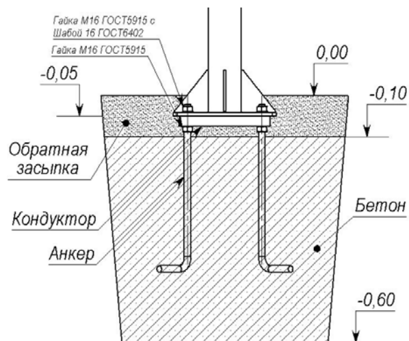
Рисунок 1 – Монтаж анкерів
