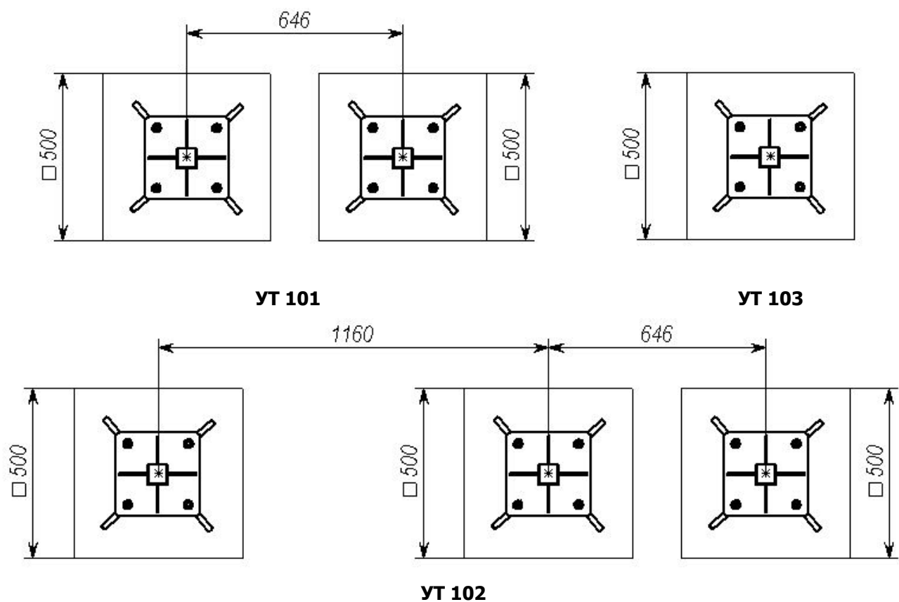
Рисунок 1 – Монтаж анкерів
