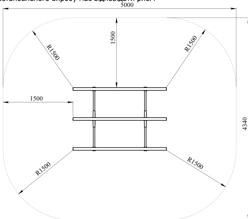
Рис. 4 Зона безпеки
