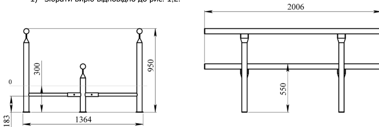
Рис. 2 Габаритні розміри
