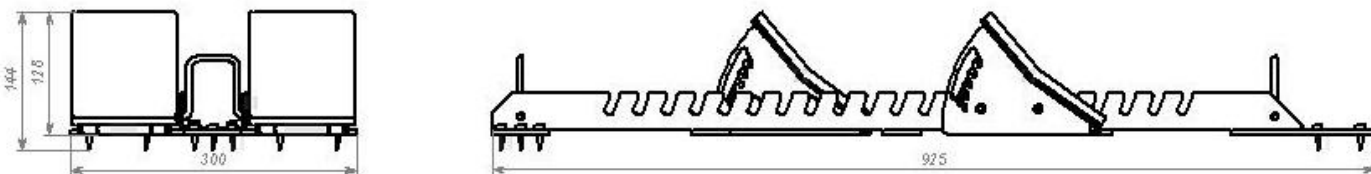
МАЛЮНОК 2 «Габаритні розміри виробу»
