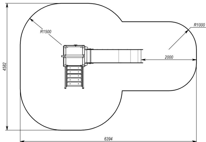
Рисунок 1 -Площа для монтажу та зона приземлення
