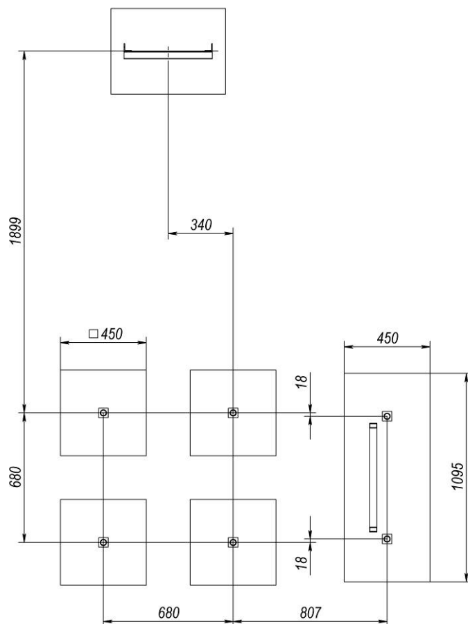
Рисунок 2 – Схема розташування фундаментів
