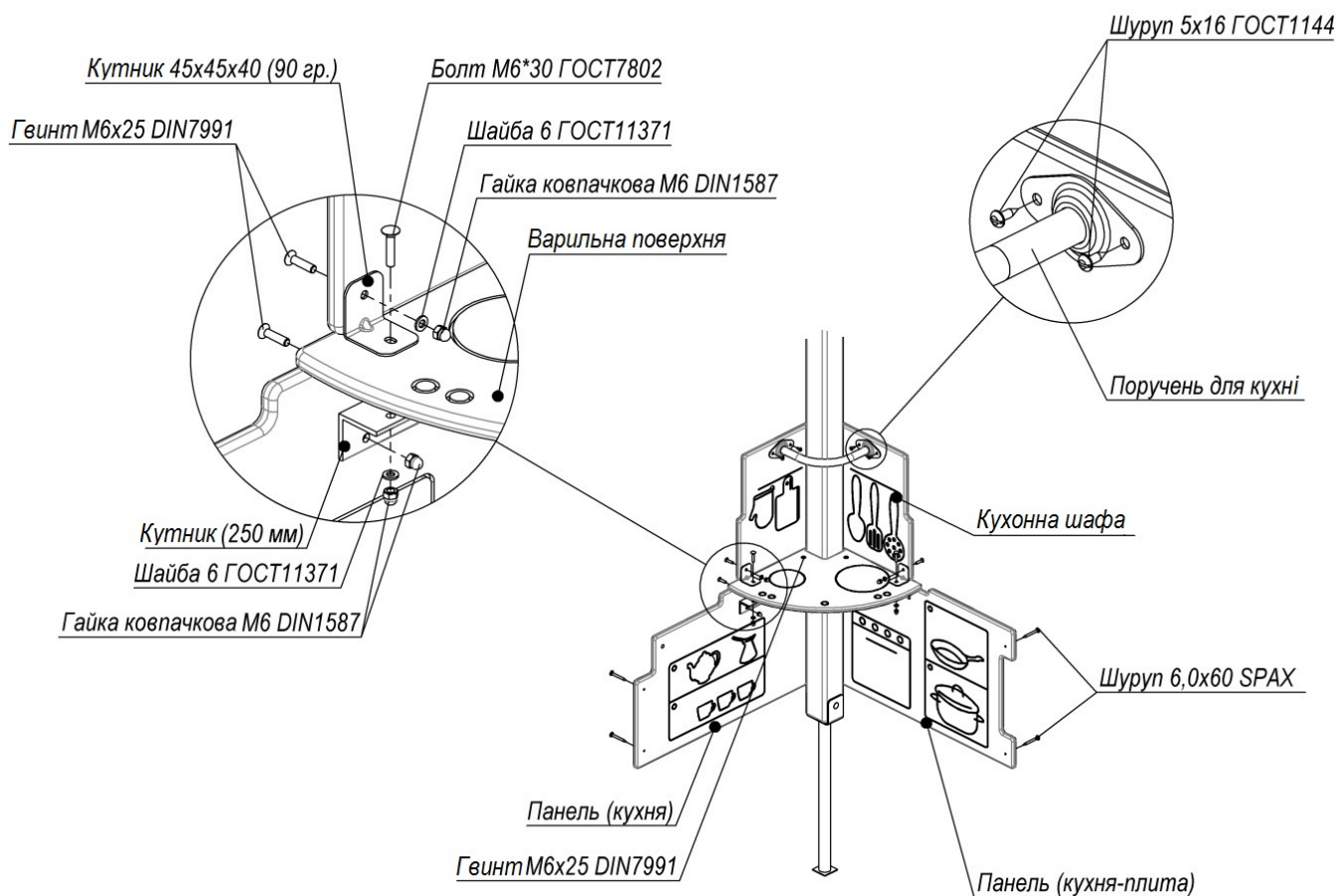
Рисунок 7 – Схема складання варильної поверхні
