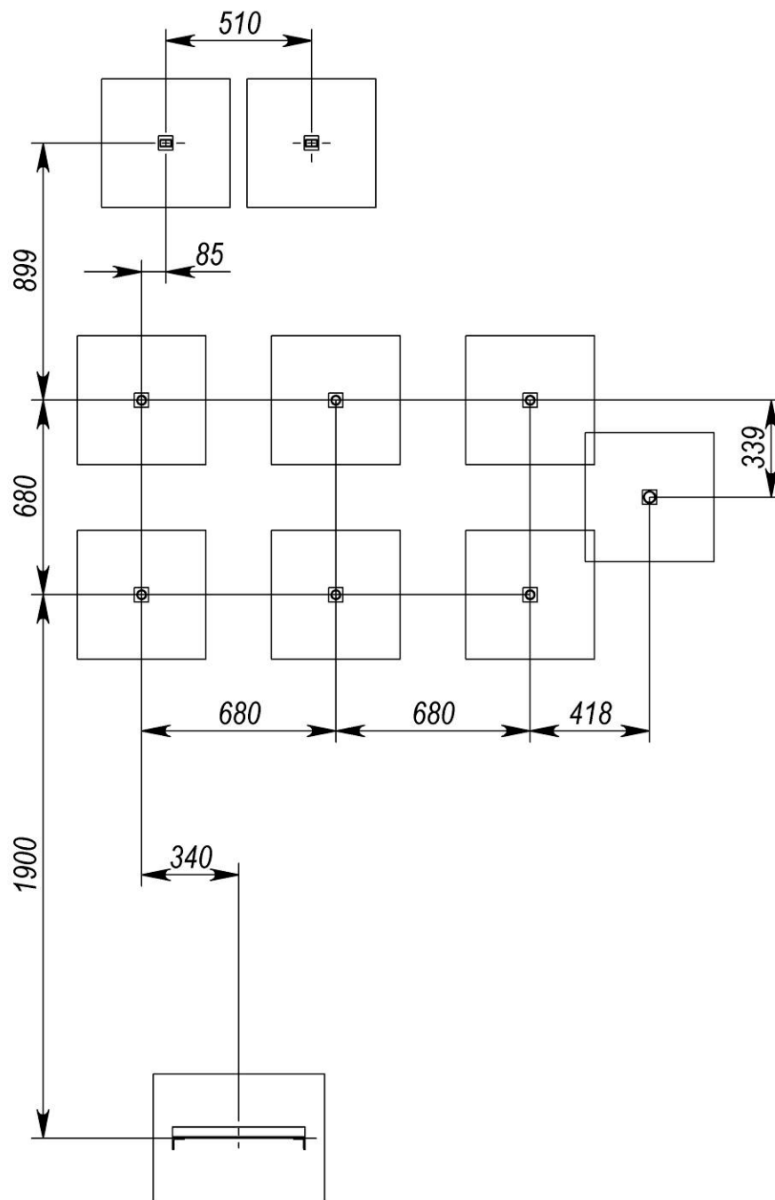
Рисунок 2 – Схема розташування фундаментів
