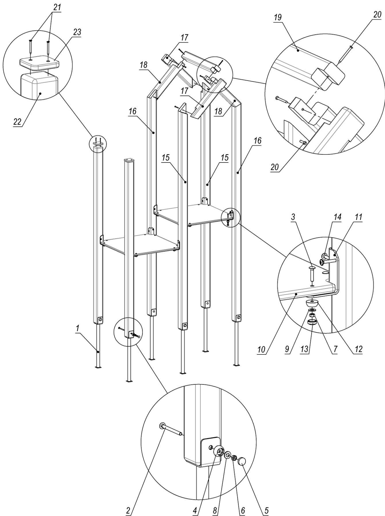
Рисунок 3 – Схема складання вежі подвійної
