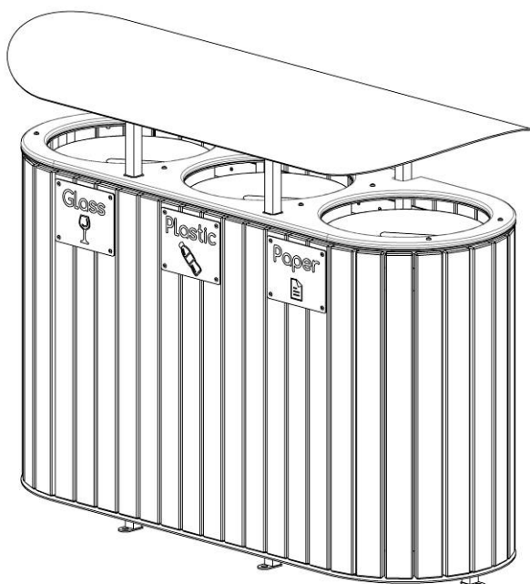
LP213.1 Урна сортувальна Elite 3x70 л (з кришкою)
