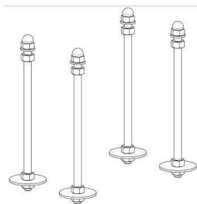
Рисунок 7 – Заклада для урн LP700
