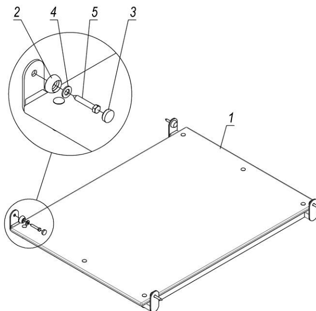
Рисунок 22 – Схема складання перил прямих
