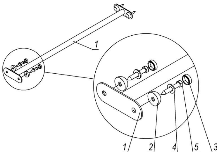
Рисунок 20 – Схема складання огорожі
