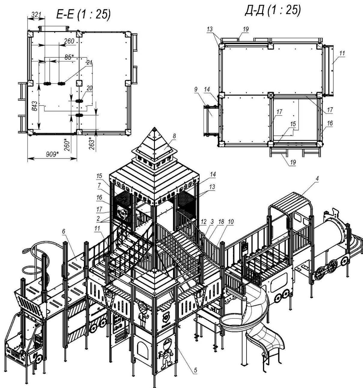
Рисунок 4- Габаритні розміри комплексу
