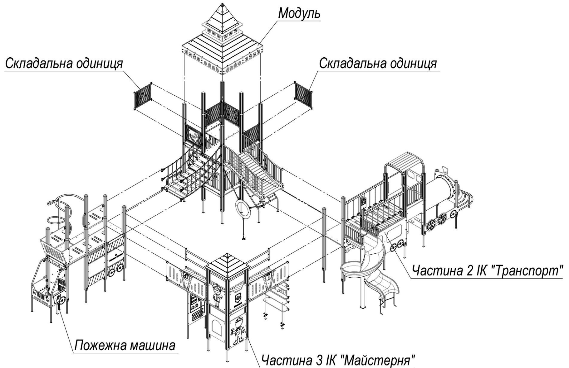
Рисунок 1 – Розбивка ігрового комплексу на частини
