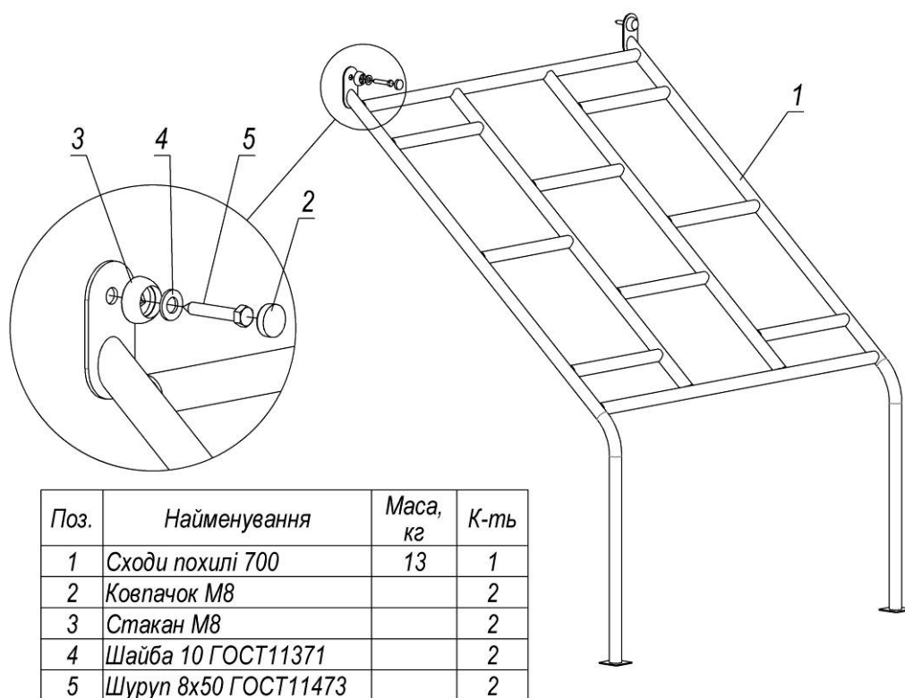
Рисунок 18 – Схема складання сходів похилих
