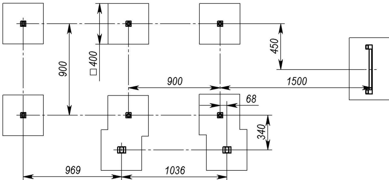
Рисунок 10 - Схема розташування фундаментів
