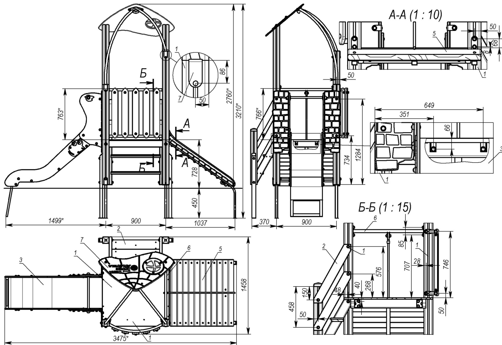
Рисунок 1 - Комплектація та характеристики складових частин виробу
