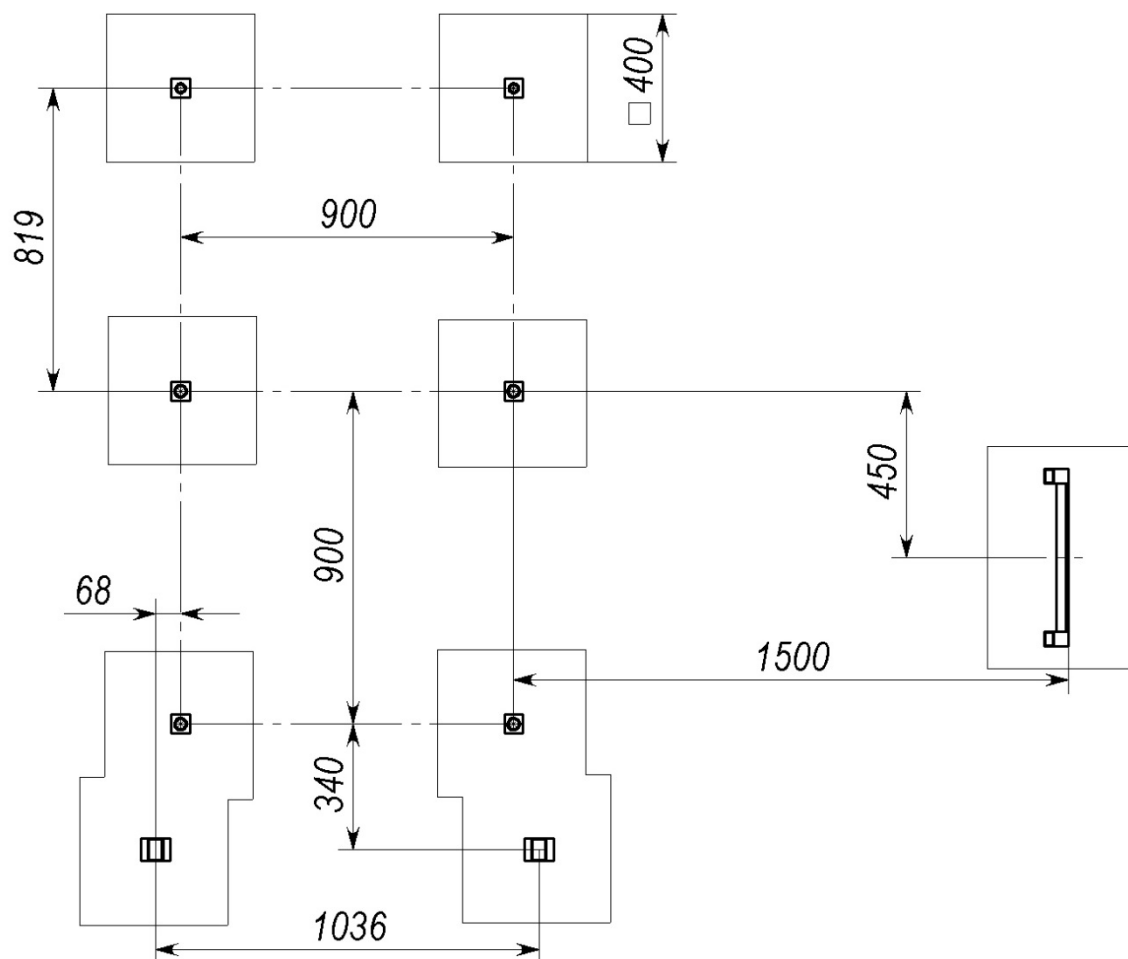
Рисунок 9 - Схема розташування фундаментів
