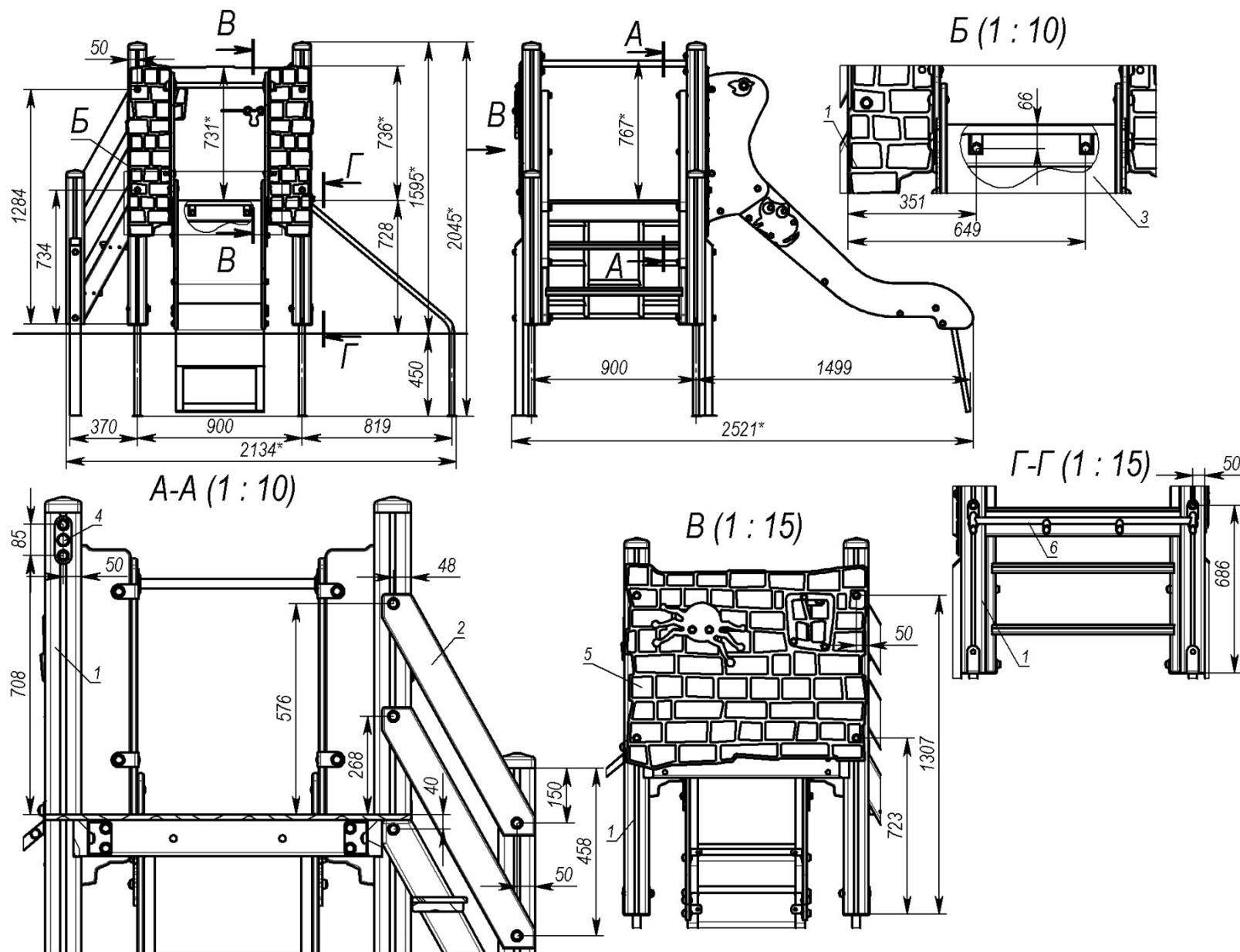
Рисунок 1 - Комплектація та характеристики складових частин виробу
