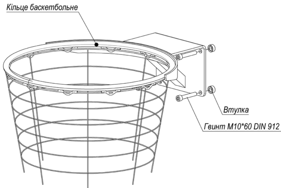
Рисунок 5 – Кріплення кільця баскетбольного під щит акриловий (для УТ405.1-01, УТ405.1-1,5)
