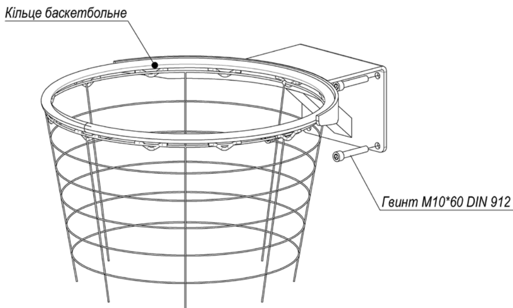
Рисунок 5 – Кріплення кільця баскетбольного під щит акриловий (для УТ405.1-01, УТ405.1-1,5)
