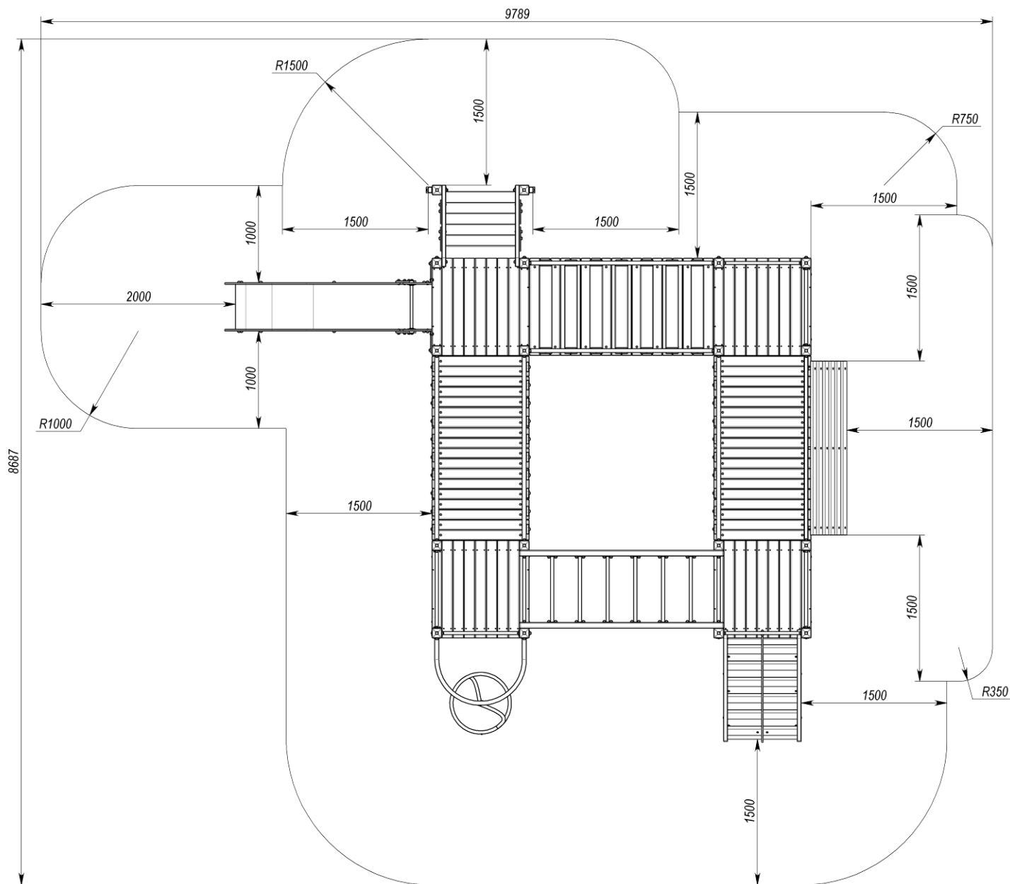
Рисунок 1 - Площа для монтажу та зона безпеки
