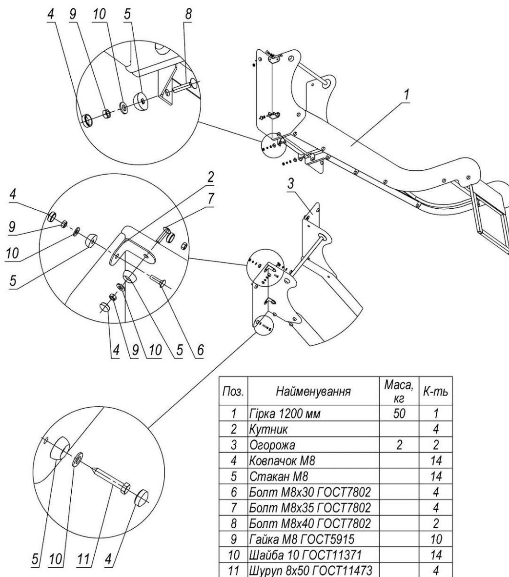
Рисунок 9 – Схема збирання гірки 1200мм
