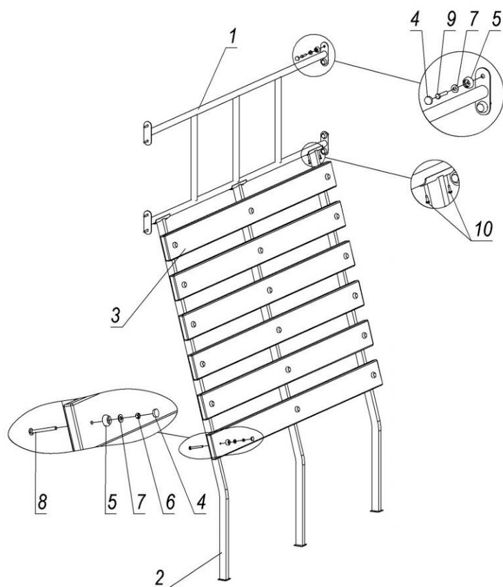
Рисунок 6 - Зібрати та встановити драбину спіральну
