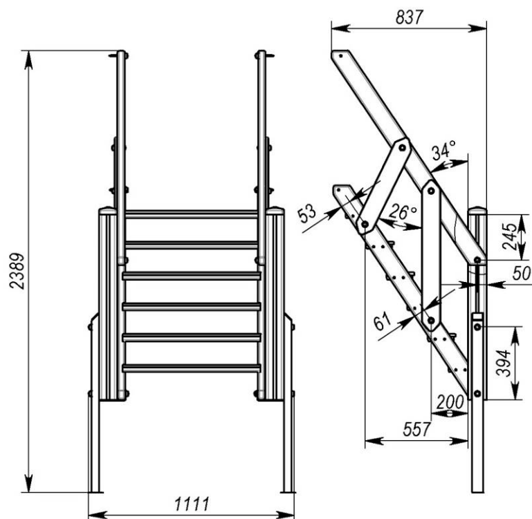
Рисунок 8 – Зібрати та встановити сходи дерев'яні
