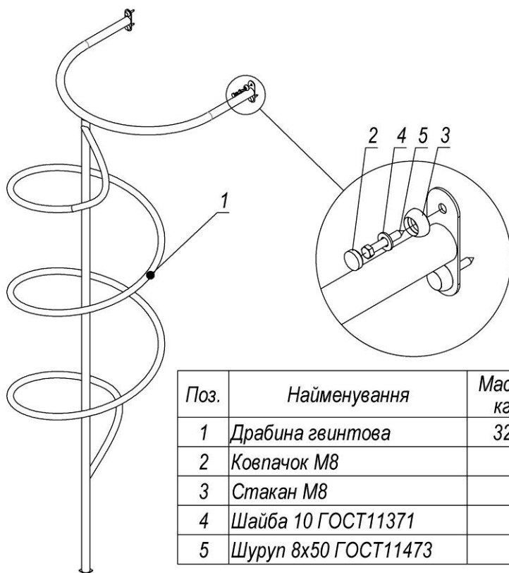
Рисунок 6 - Зібрати та встановити драбину спіральну
