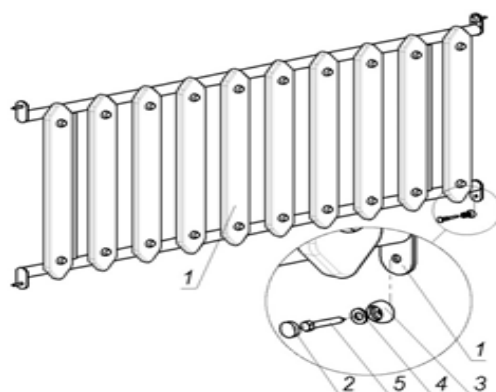
Рисунок 11 – Схема складання рукоходу
