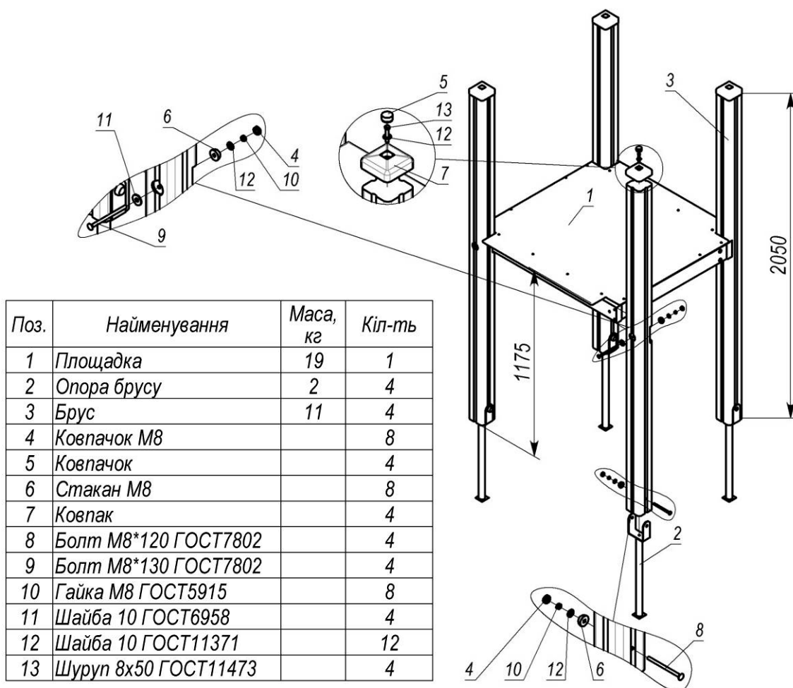
Рисунок 3 - Зібрати та встановити вежу
