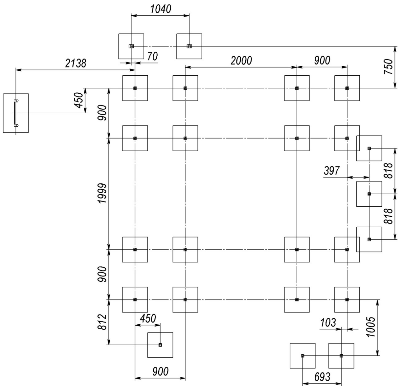
Рисунок 2 – Схема розміщення фундаментів
