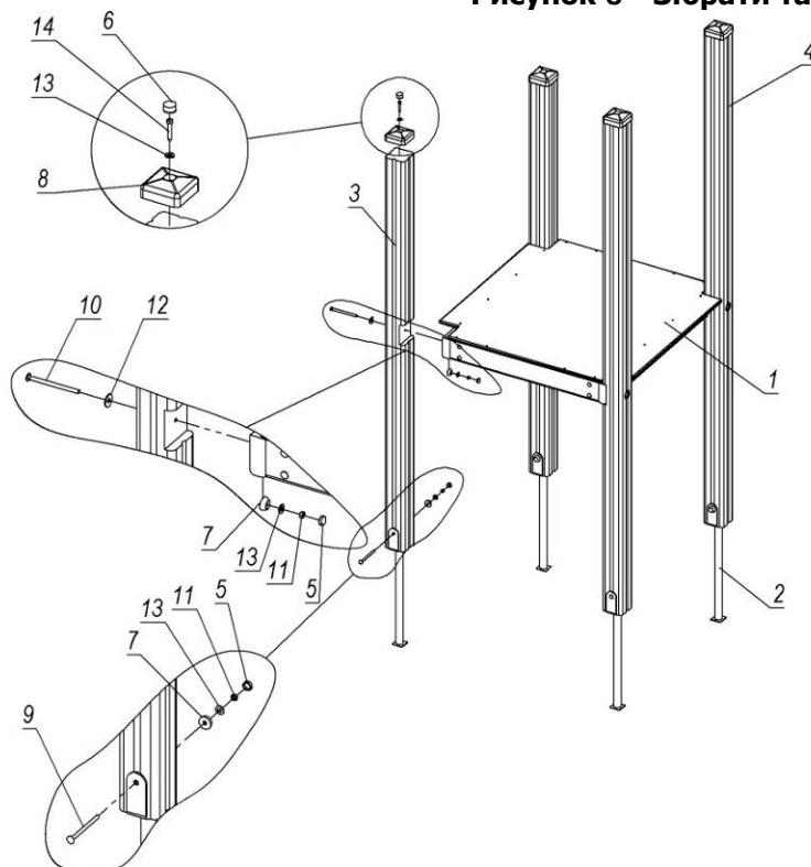
Рисунок 3 - Зібрати та встановити вежу
