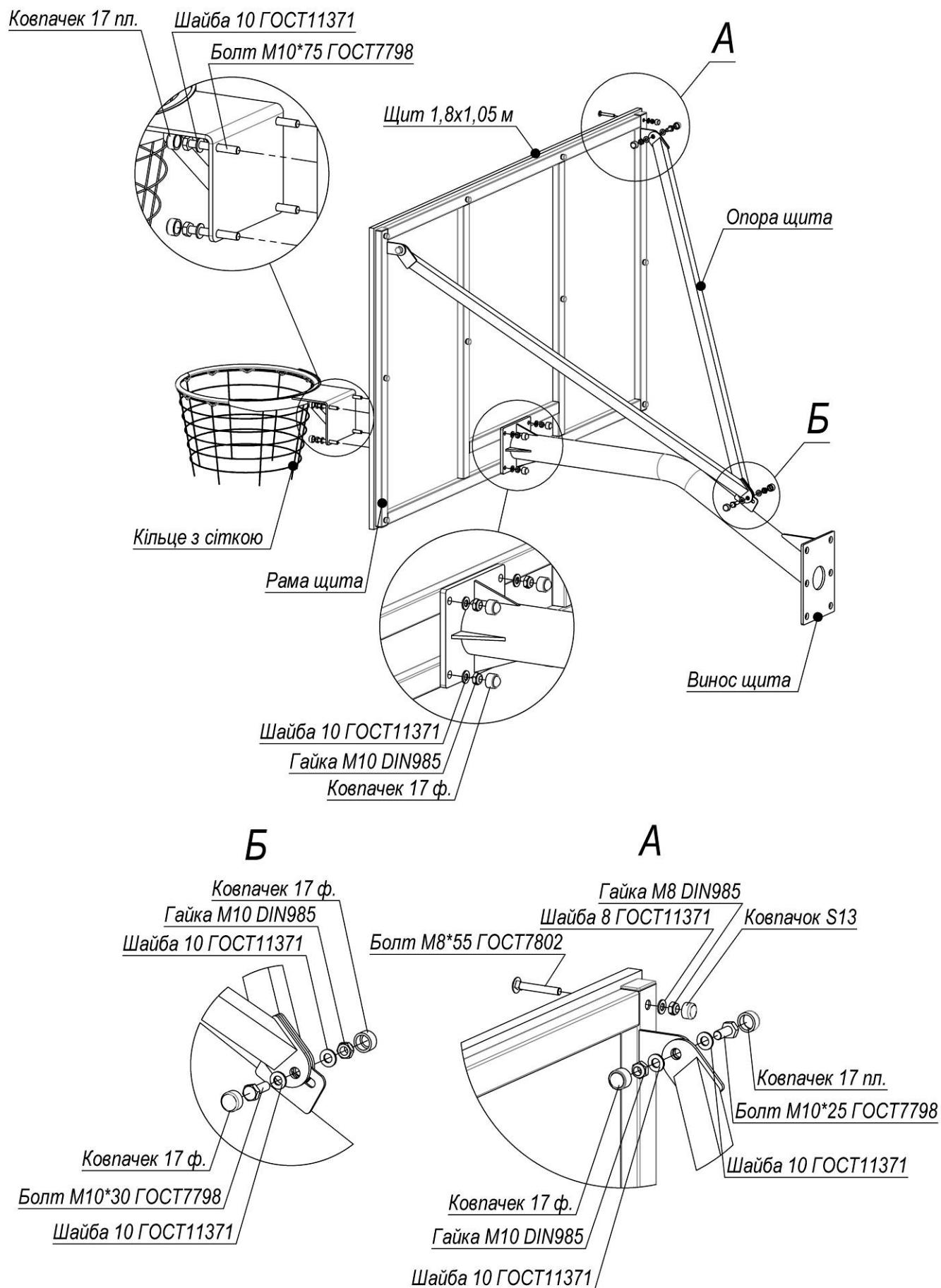
Рисунок 2 – Схема монтажу 1
