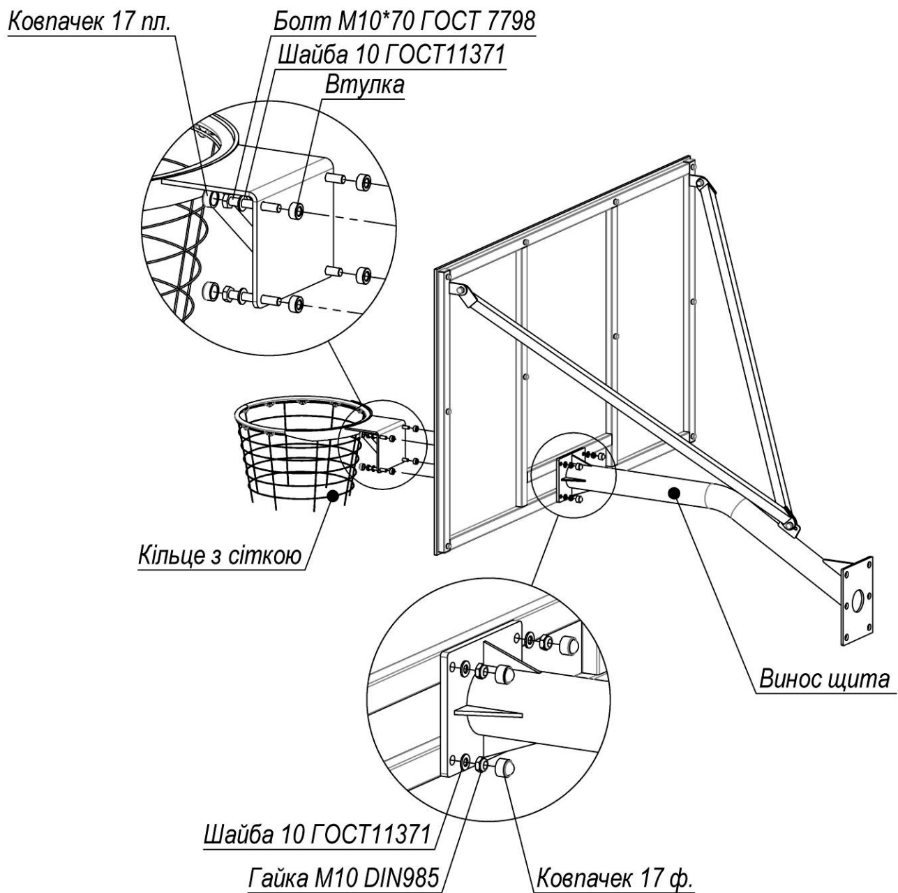
Рисунок 3 – Схема кріплення кільця баскетбольного для УТ410.1
