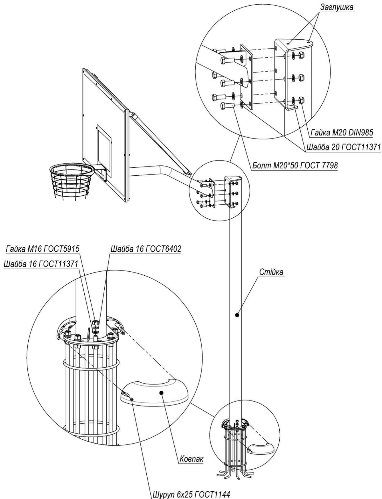
Рисунок 4 – Схема монтажу 3
