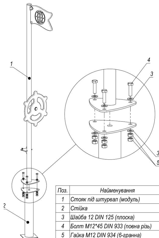
Рисунок 2 – Схема складання сидіння
