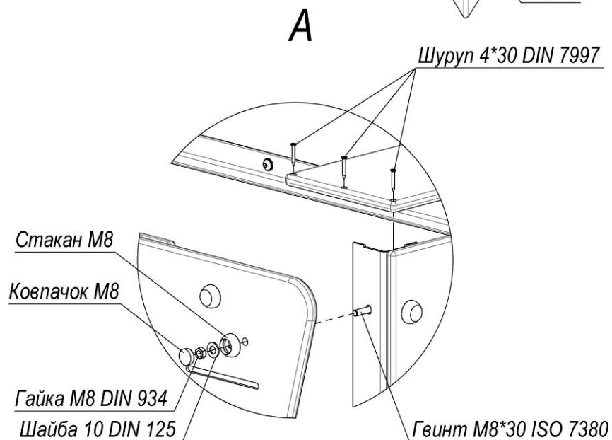
Рисунок 1 – Схема встановлення бортиків
