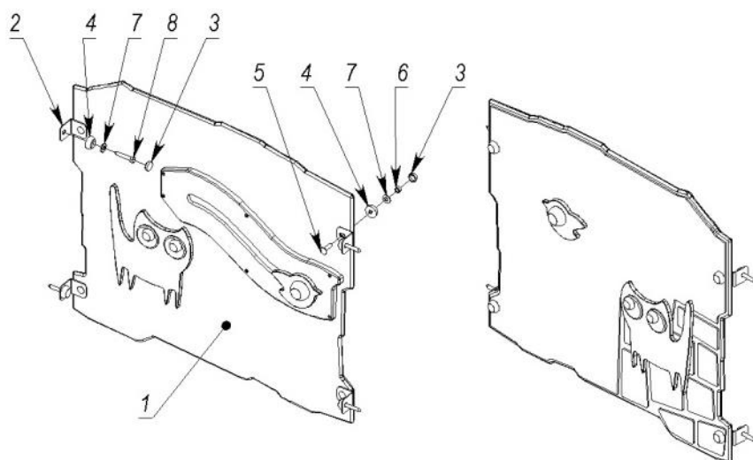
Рисунок 15 - Комплектність та схема складання кільцевих сходів
