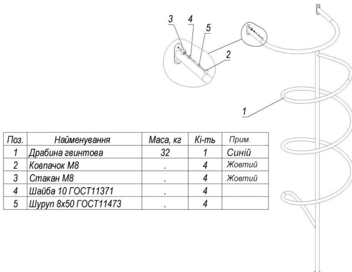
Рисунок 6 - Комплектність та схема складання спіральних сходів
