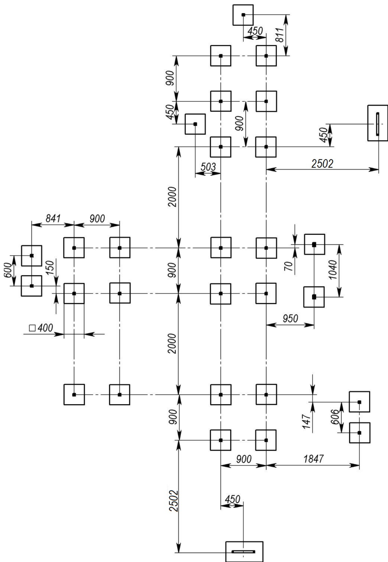
Рисунок 21 - Схема розташування фундаментів
