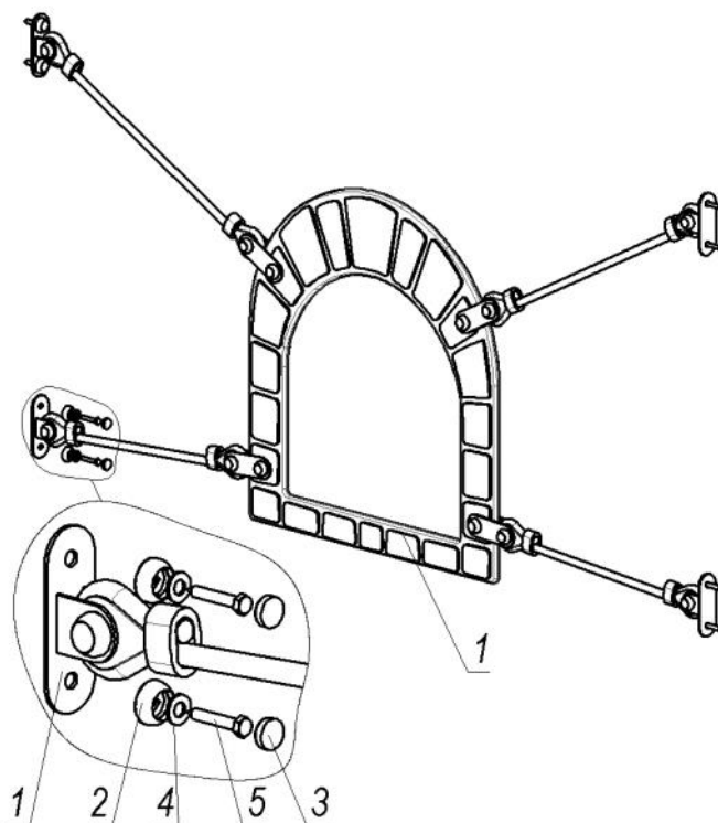
Рисунок 19 - Комплектність та схема складання стяжок металевих
