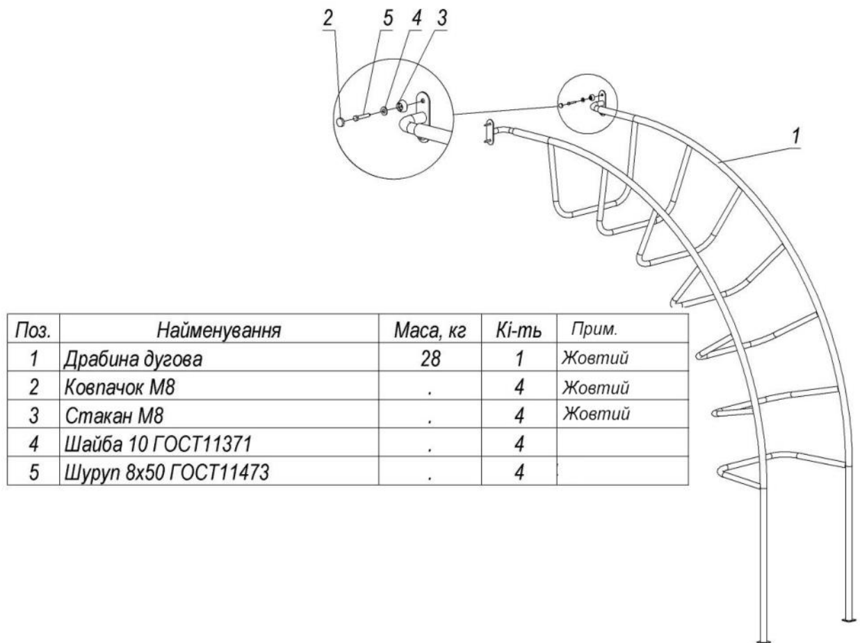
Рисунок 17 - Комплектність та схема складання драбини дугової 1500мм
