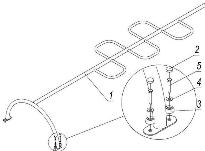
Рисунок 17 - Комплектність та схема складання драбини дугової 1500мм
