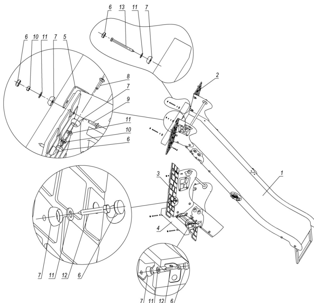
Рисунок 8 - Комплектність та схема складання огороження Павук
