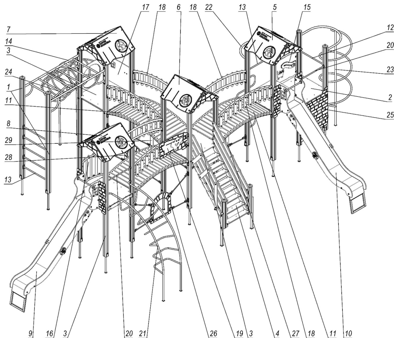
Рисунок 1 - Комплектація та характеристики складових частин виробу
