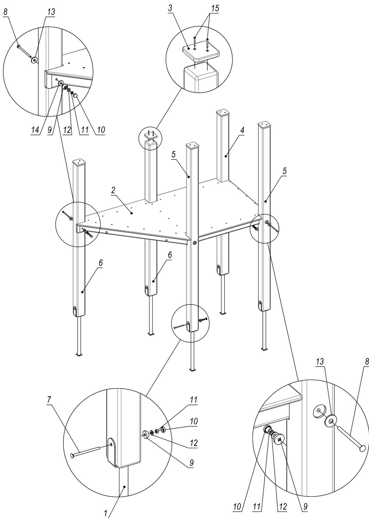
Рисунок 3 – Схема складання вежі
