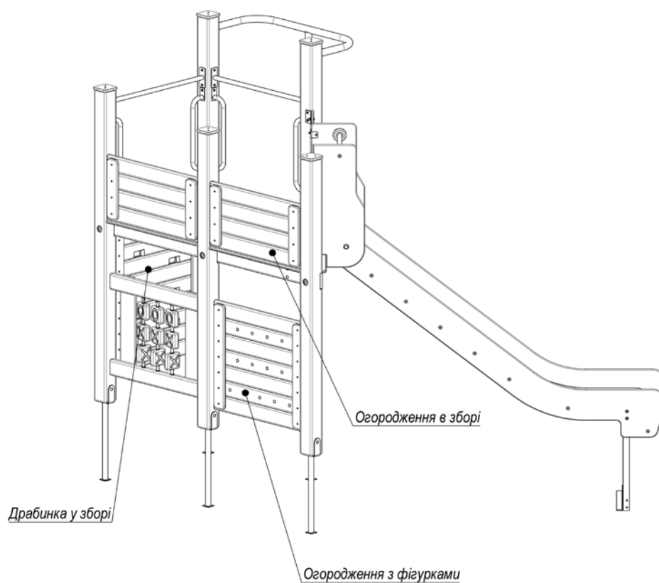
Рисунок 7 – Схема збирання панелі
