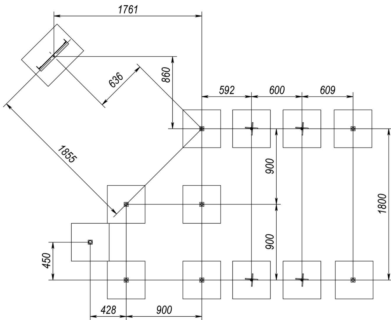
Рисунок 2 – Схема розташування фундаментів
