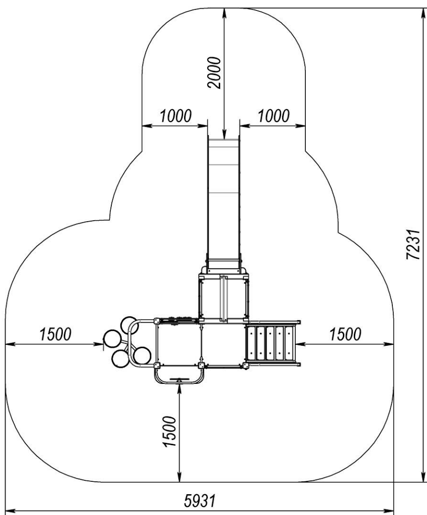
Рисунок 1 -Площа для монтажу та зона приземлення
