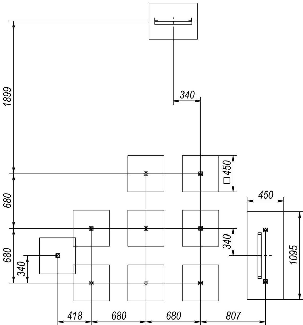
Рисунок 2 – Схема розташування фундаментів
