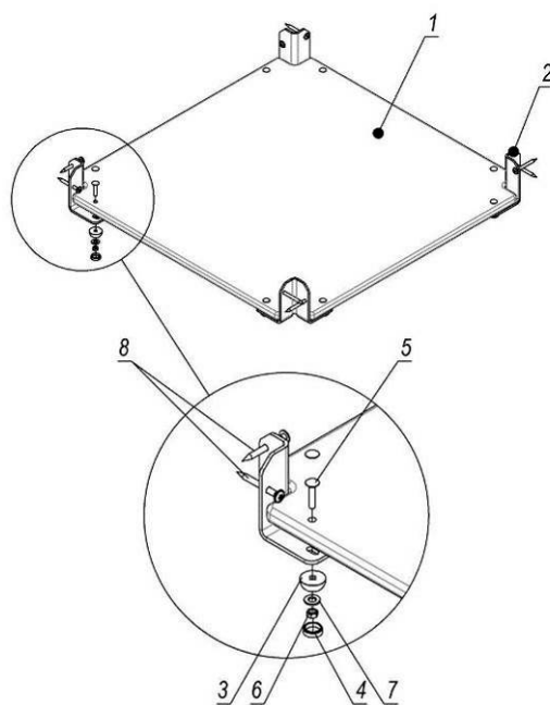
Рисунок 5 – Схема складання стійки 2м
