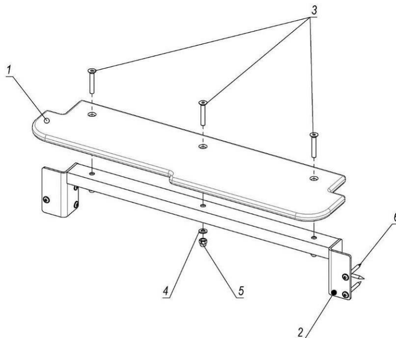
Рисунок 7 – Схема складання панелі (складання інших панелей ідентична)
