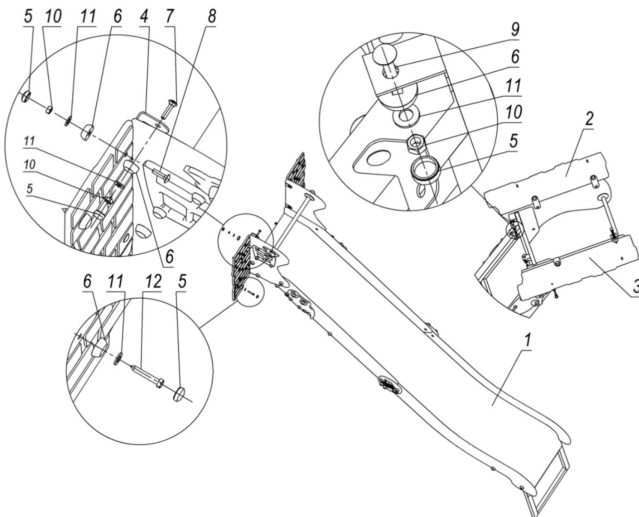
Рисунок 9 - Комплектність та схема складання панелі
