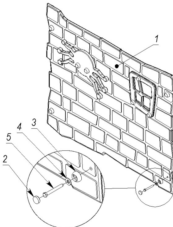
Рисунок 8 - Комплектність та схема складання підйому
