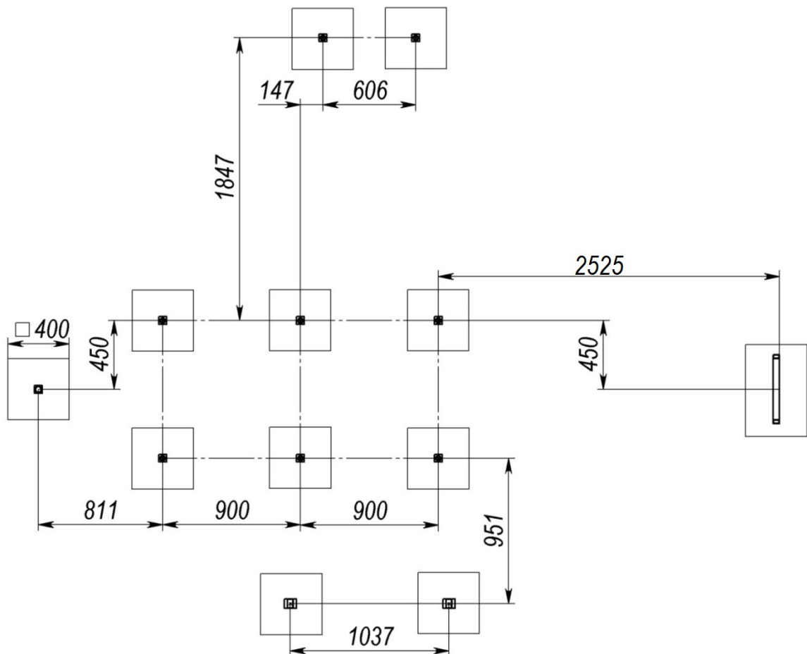
Рисунок 11 - Схема розташування фундаментів
