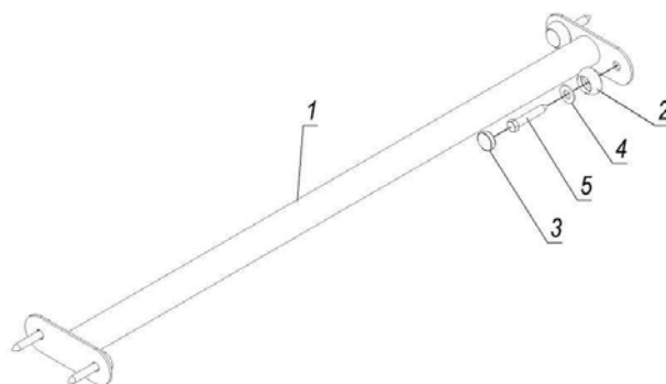
Рисунок 5 - Комплектність та схема спіральних сходів
