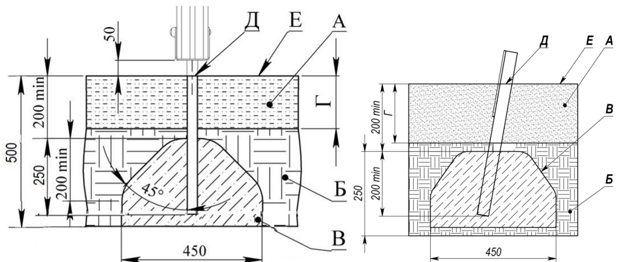
Рисунок 11 - Схема розташування фундаментів
