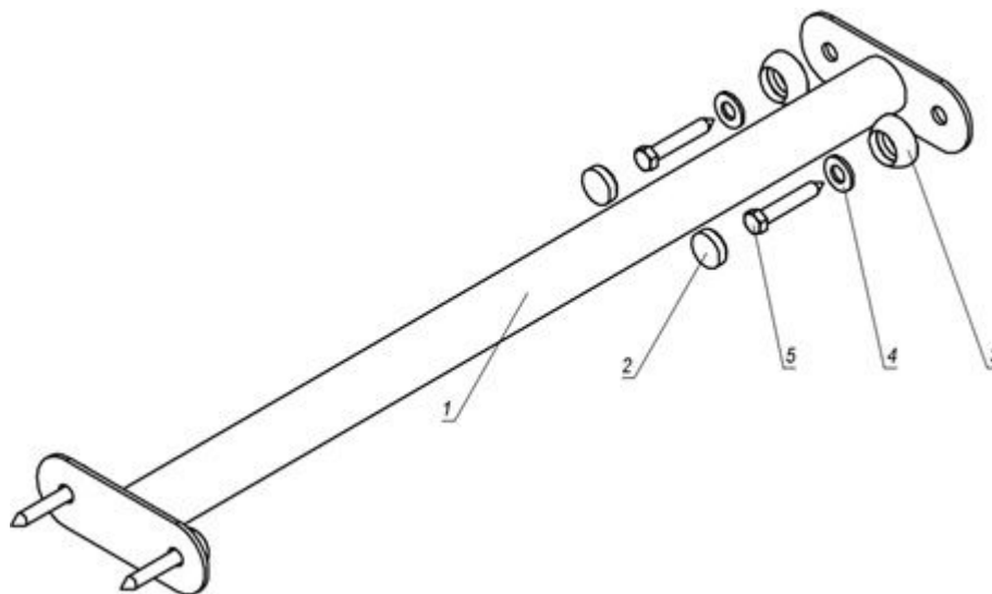
Мал. 5 - Комплектність та схема драбини дугової
