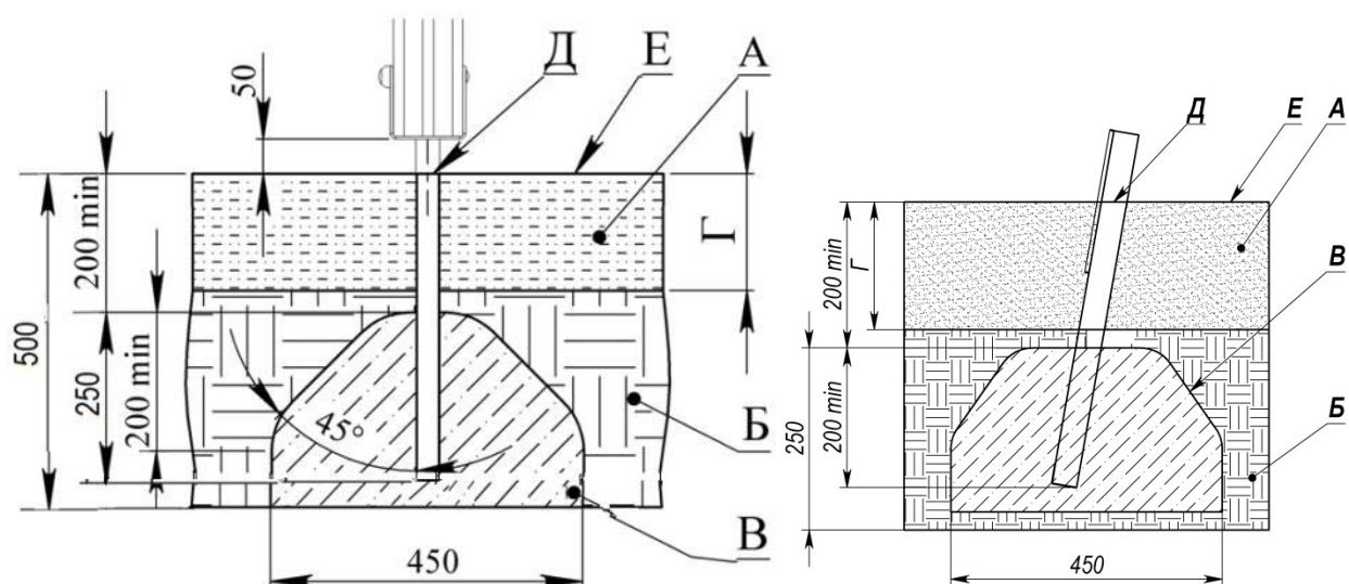
Мал. 8 - Схема розташування фундаментів
