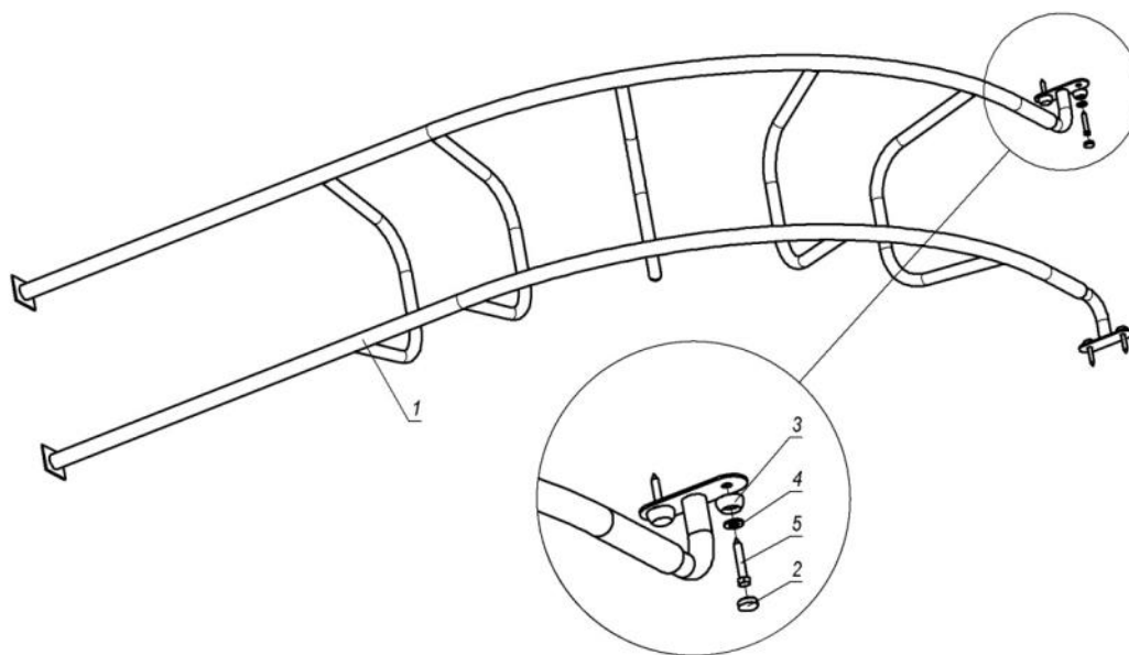
Мал. 4 - Комплектність та схема драбини східчастої
