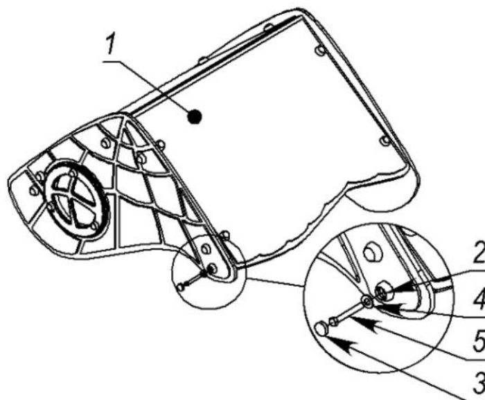
Мал. 1 - Комплектність та схема складання вежі
