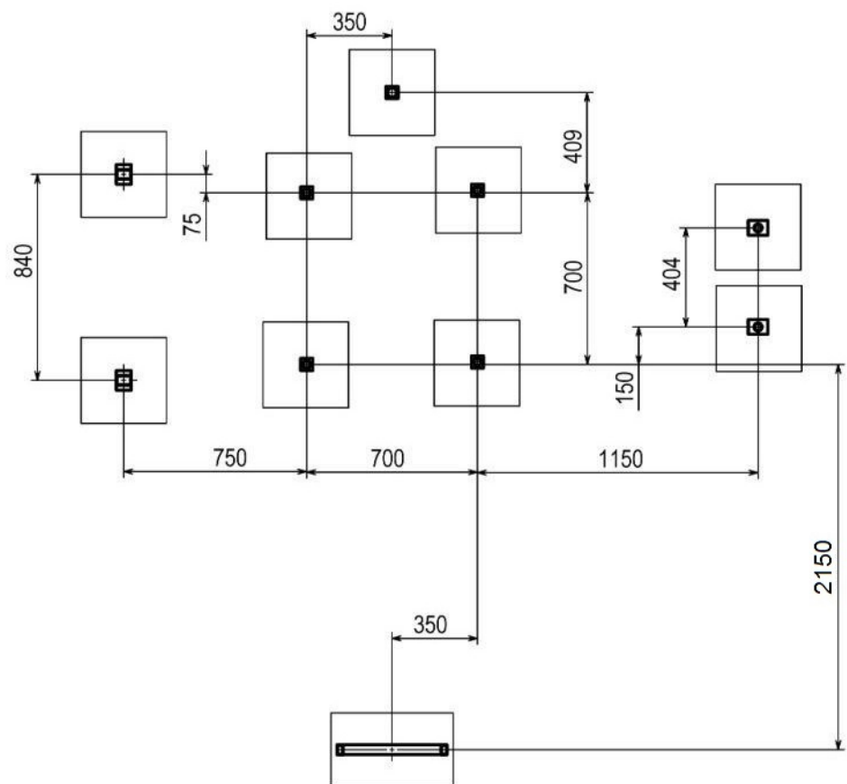
Мал. 8 - Схема розташування фундаментів
