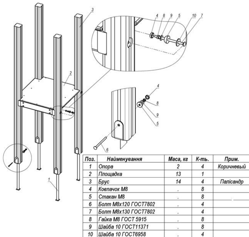
Мал. 1 - Комплектність та схема складання вежі
