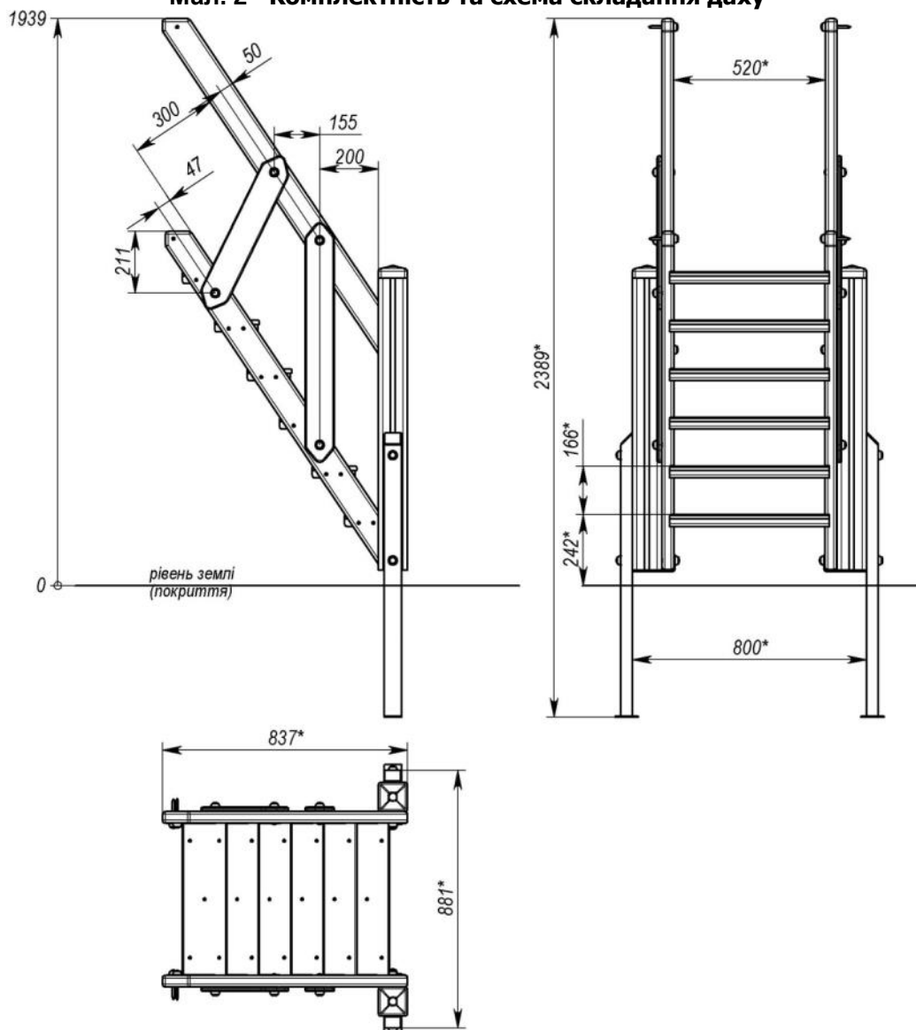
Мал. 2 - Комплектність та схема складання даху
