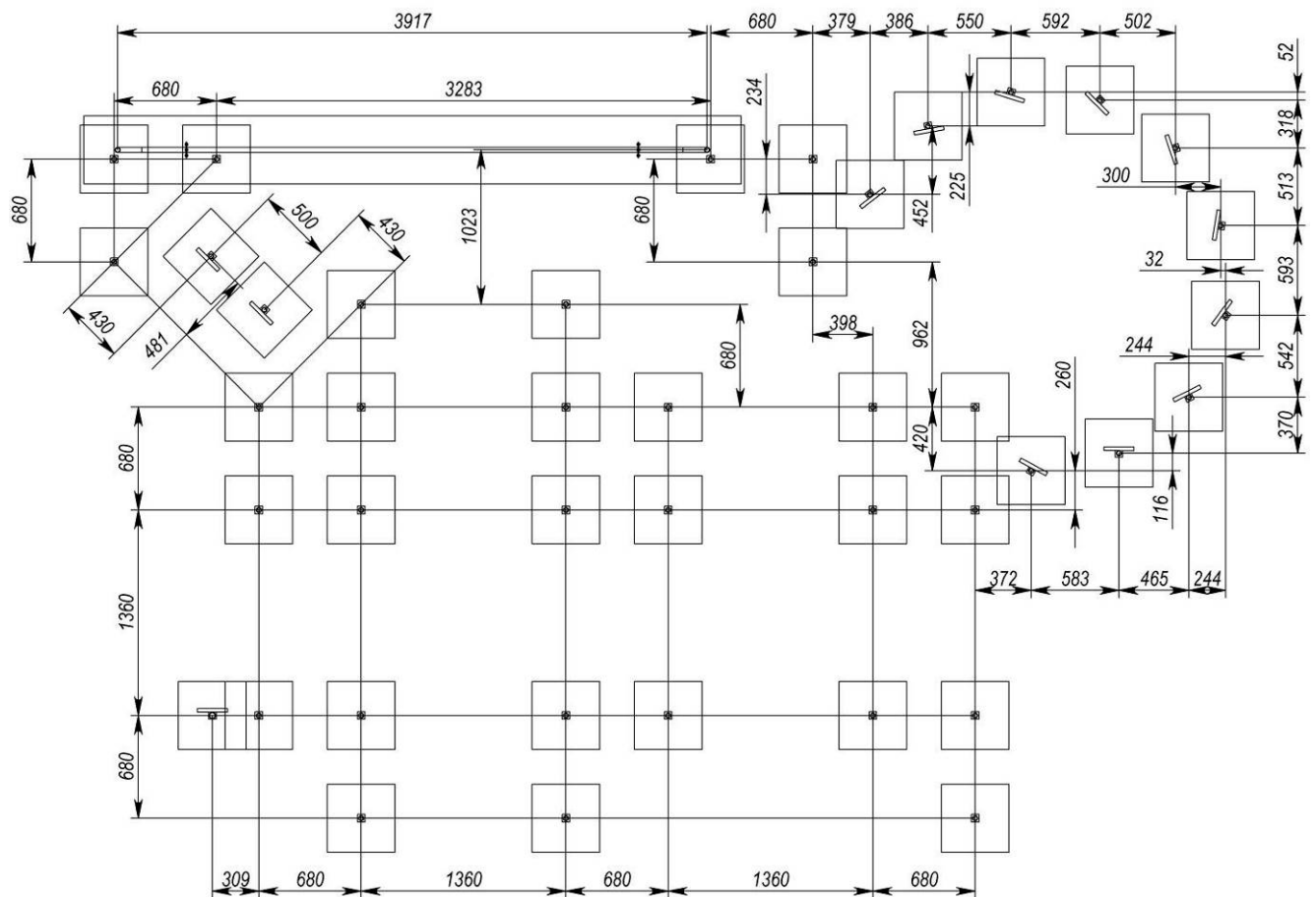
Рисунок 2 – Схема розташування фундаментів
