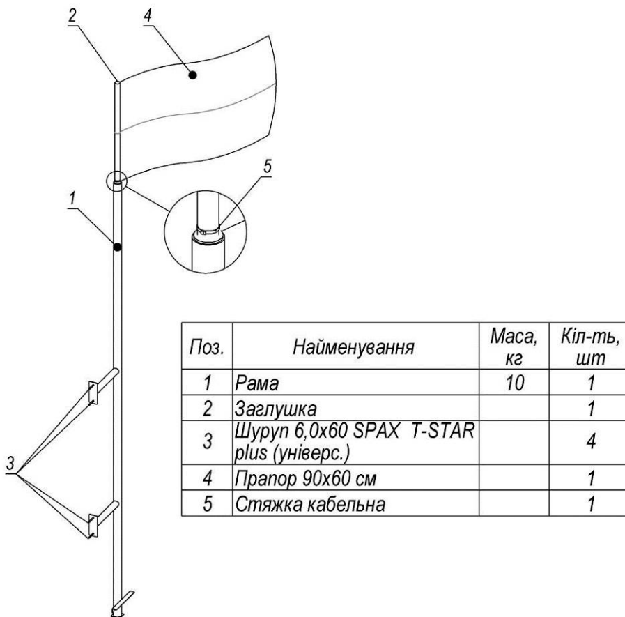
Рисунок 11 – Схема закріплення прапора
