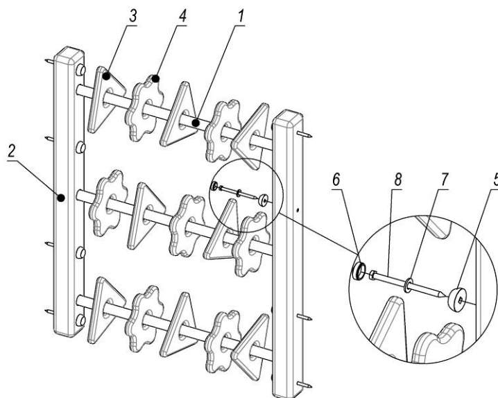
Рисунок 11 – Схема закріплення прапора
