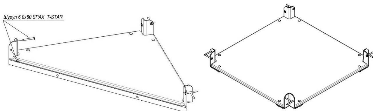
Рисунок 4 – Схема складання платформ
