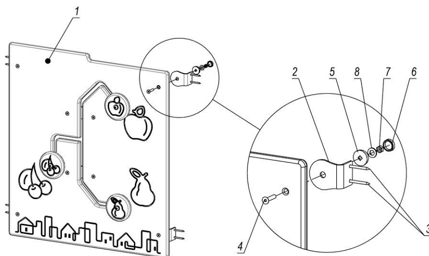
Рисунок 6 – Схема складання пенька
