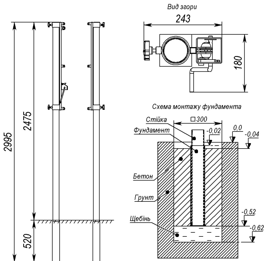
Рис. 2 - Габаритні розміри виробу та схема монтажу
