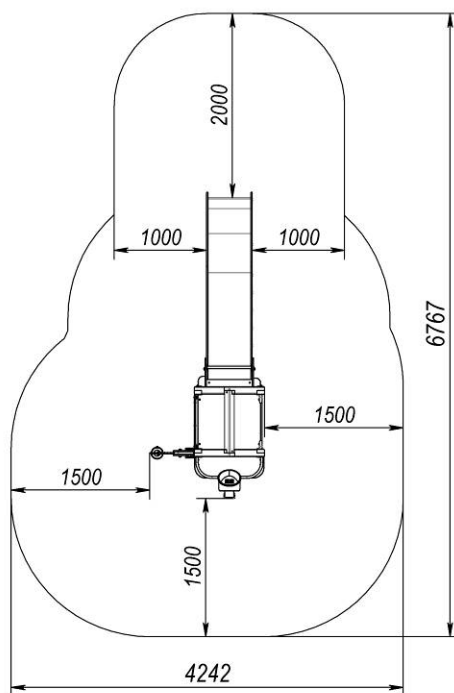
Рисунок 1 -Площа для монтажу та зона приземлення
