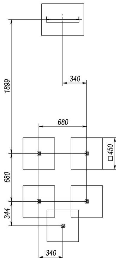
Рисунок 2 – Схема розташування фундаментів
