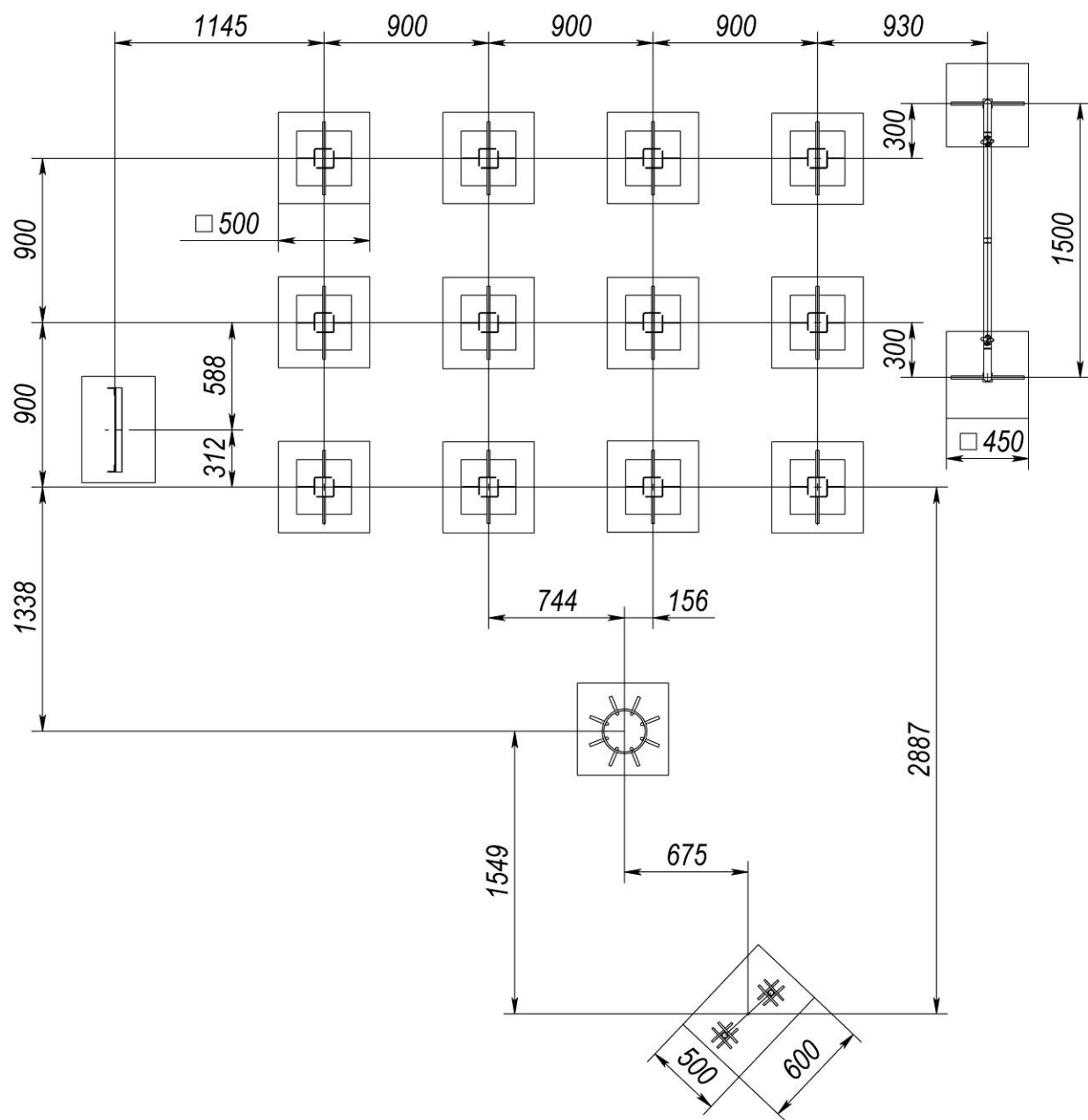
Рисунок 2 – Схема розташування фундаментів
