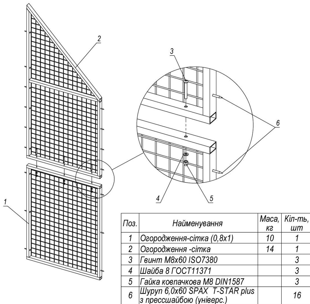
Рисунок 14 – Схема збирання огороження-сітка
