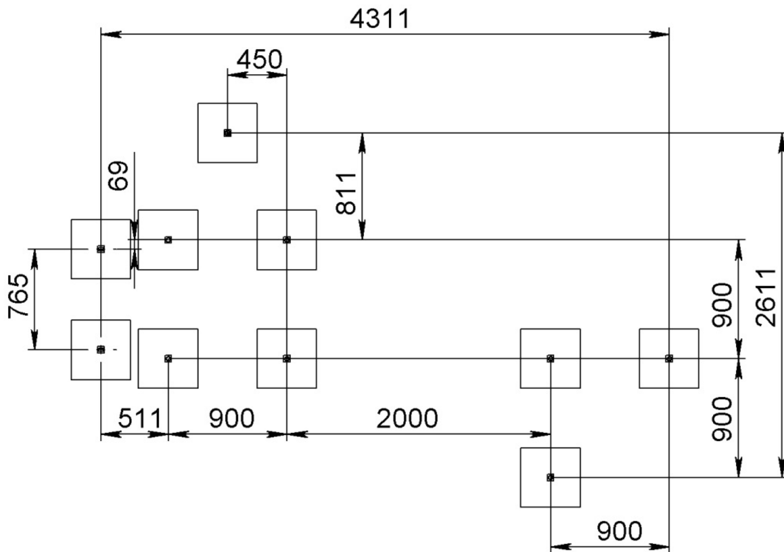
Рис. 11– Схема розташування фундаментів
