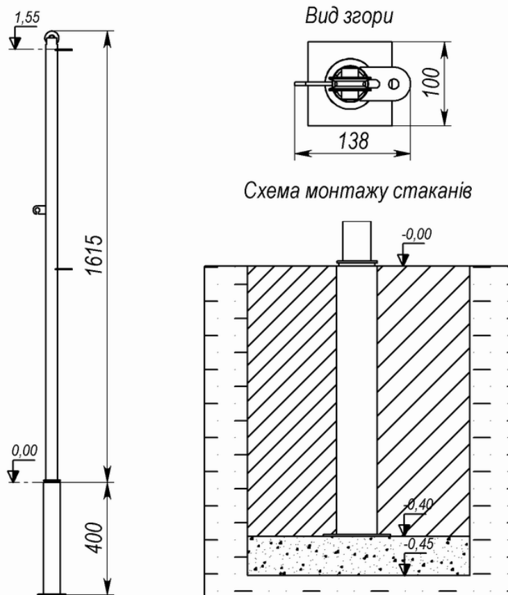
МАЛЮНОК 2 «Габаритні розміри виробу та схема монтажу»
