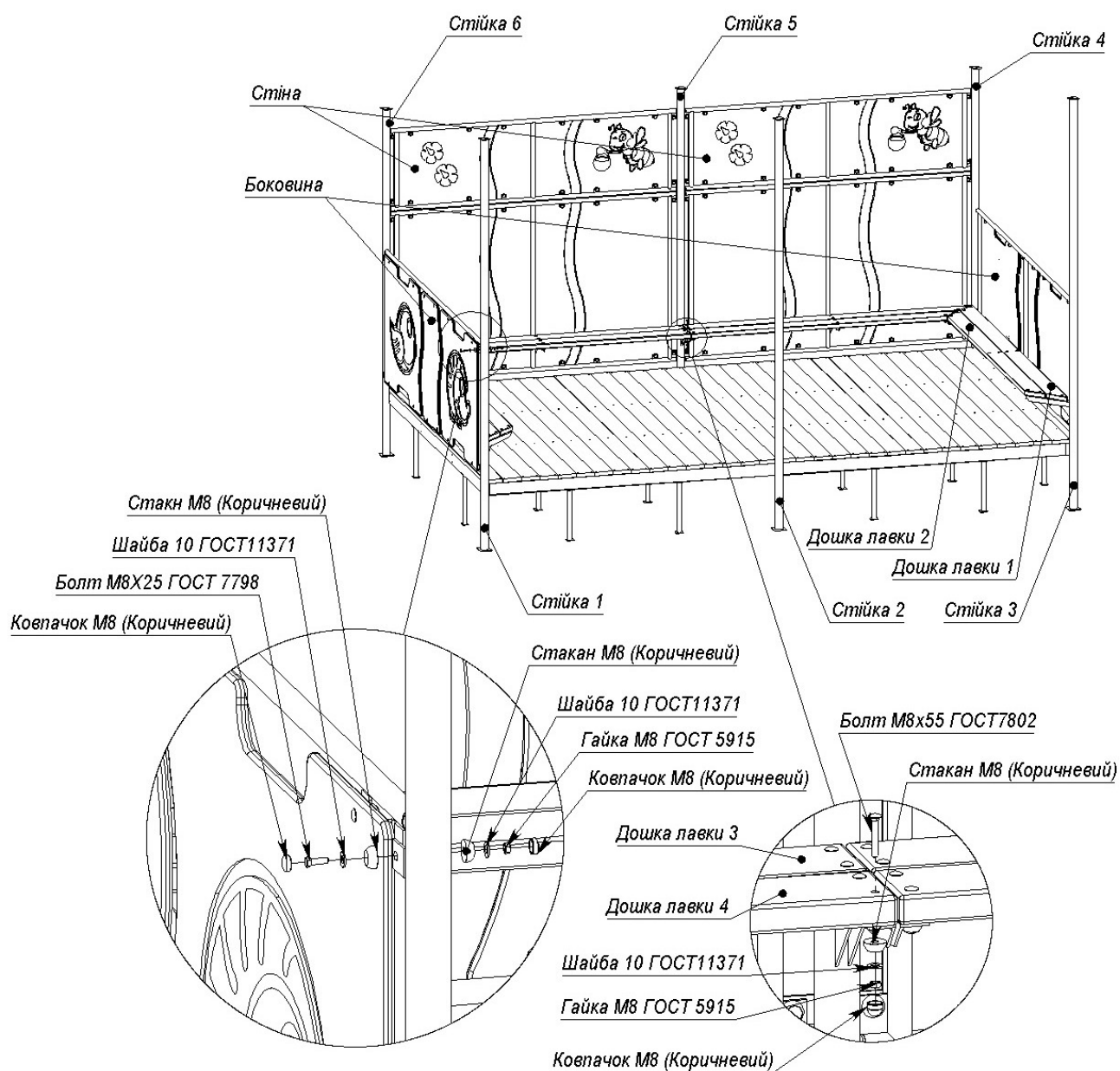
є) Схема встановлення бокових та задньої стіни
