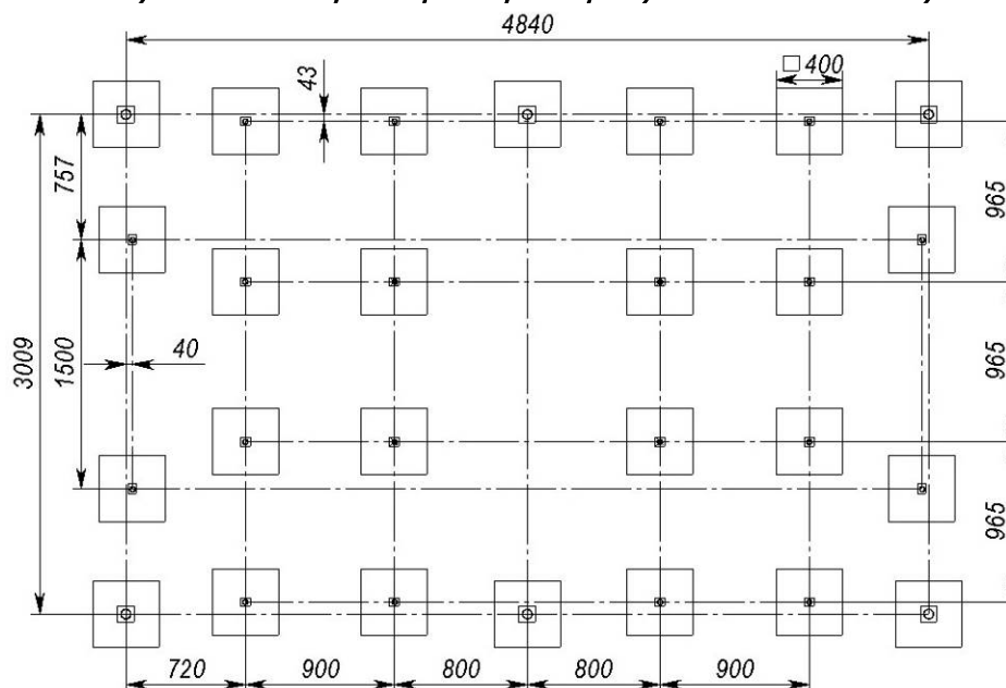
Рисунок 2 «Габаритні розміри виробу та схема монтажу»
