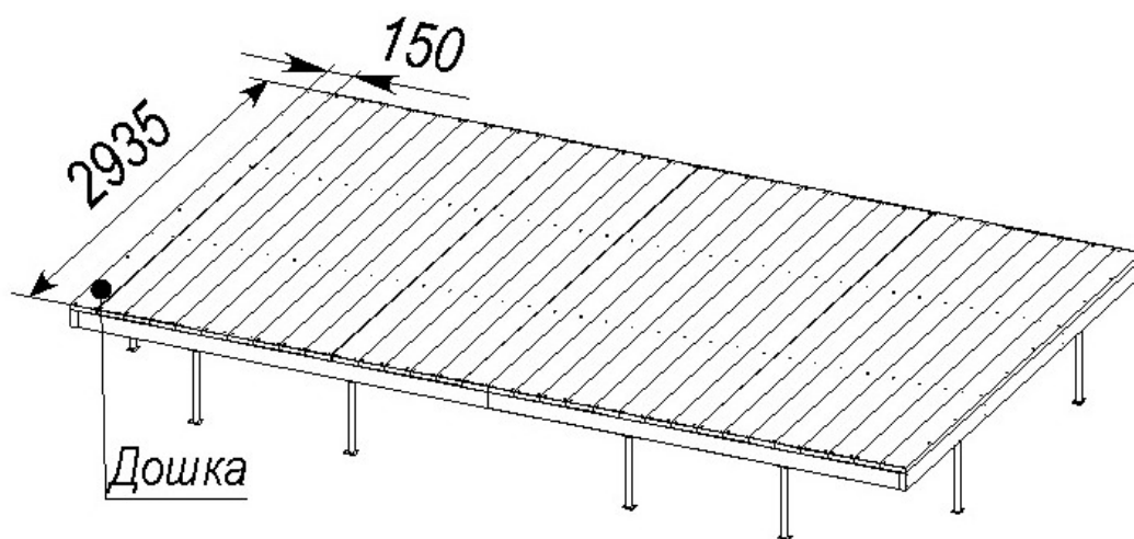
г) Схема збирання підлоги
