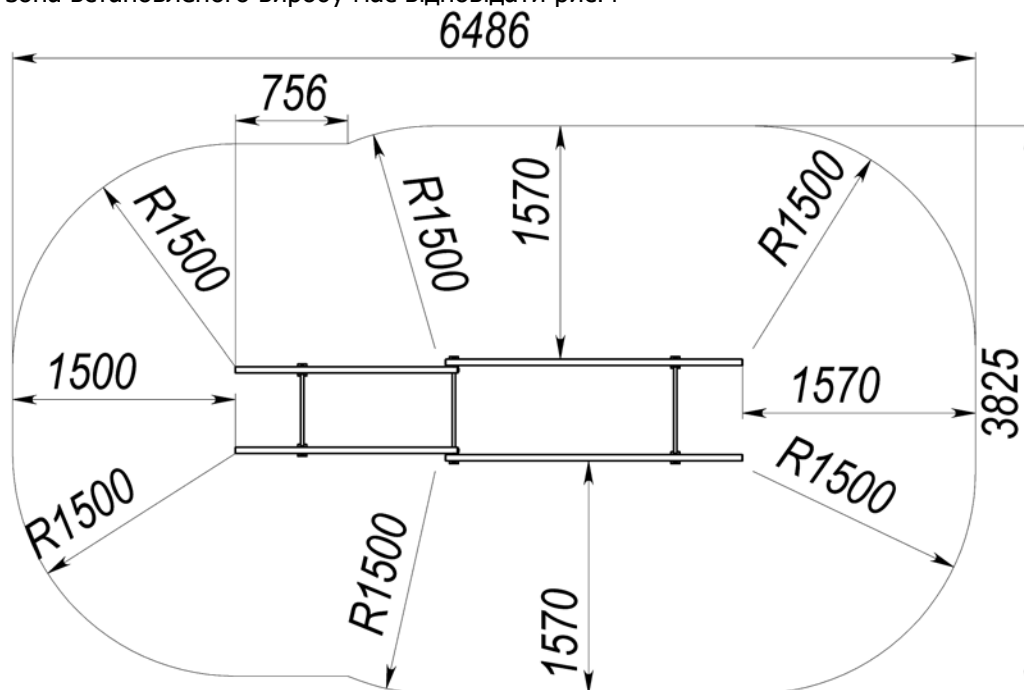
Рис. 4 Зона безпеки
