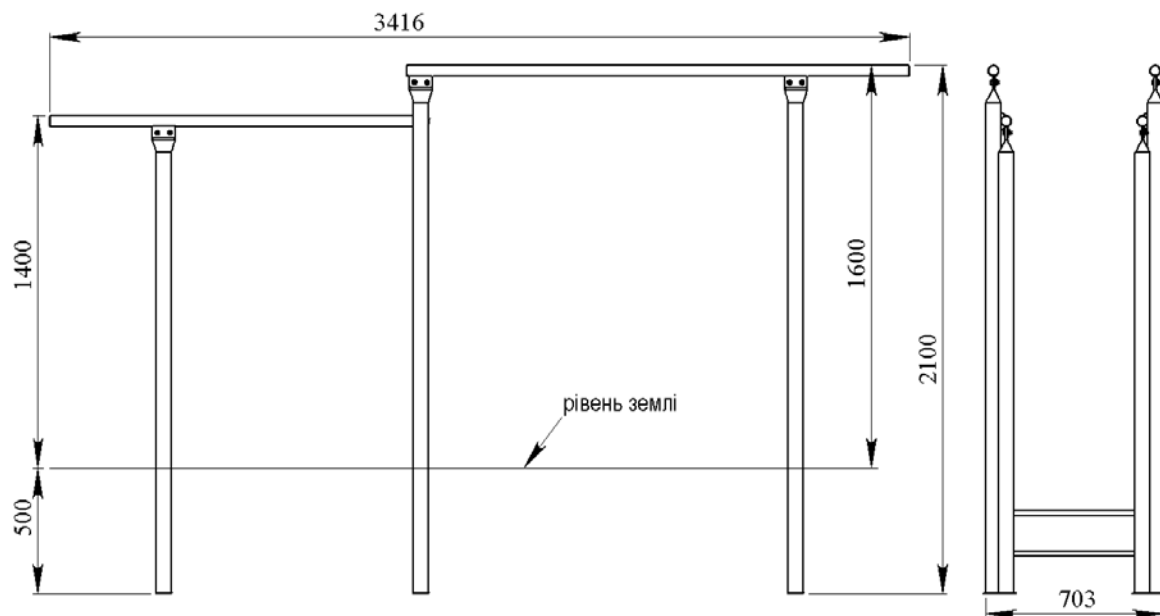
Рис. 2 Габаритні розміри
