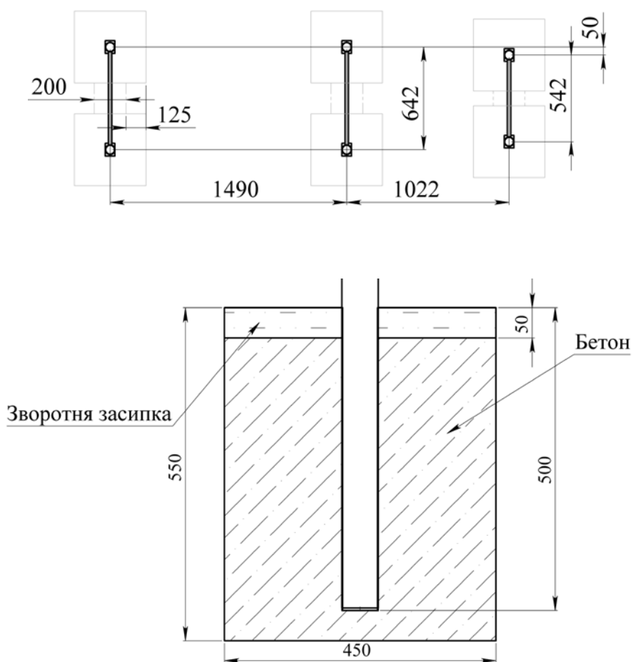
Рис. 3 Схема монтажу фундаментів
