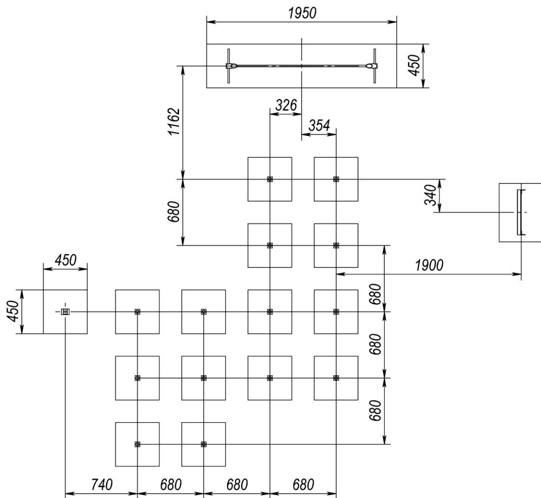
Рисунок 2 – Схема розташування фундаментів
