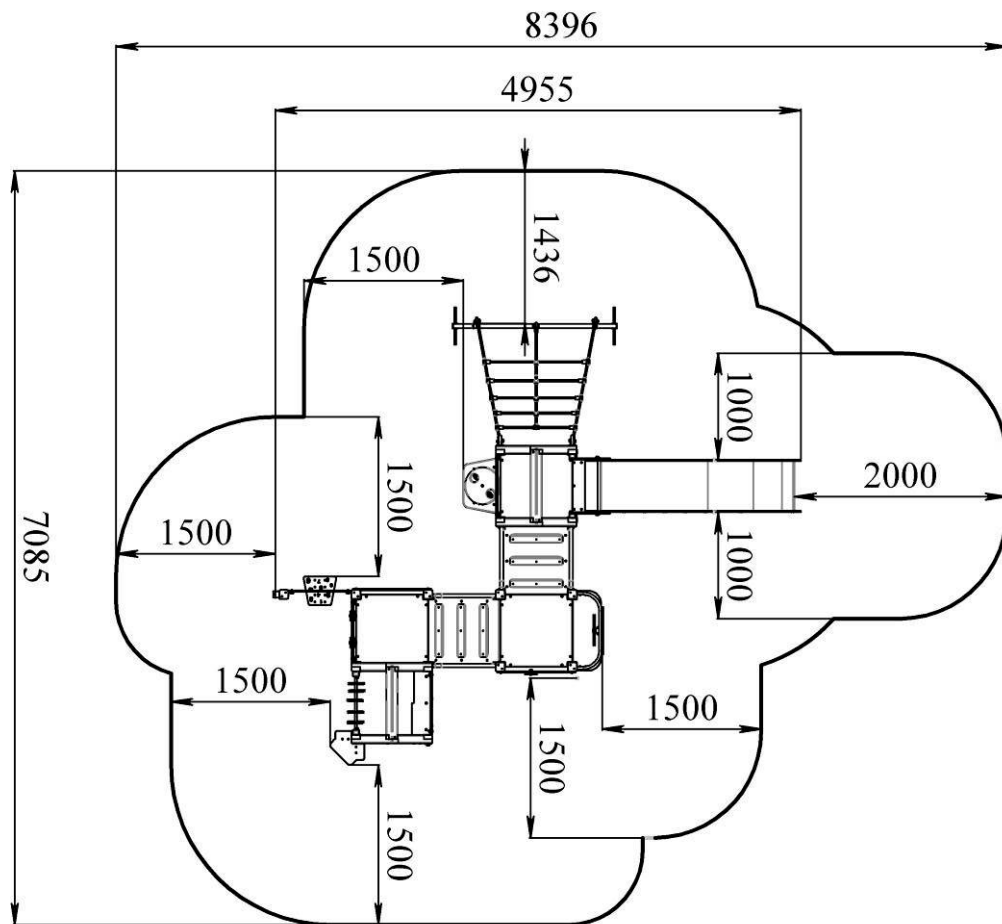
Рисунок 1 -Площа для монтажу та зона приземлення
