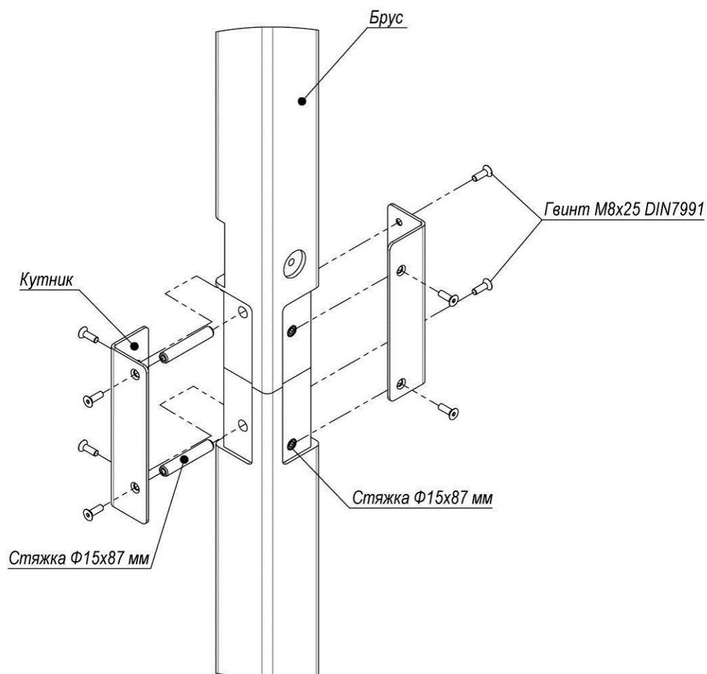
Рисунок 13 – Схема з'єднання двох брусів
