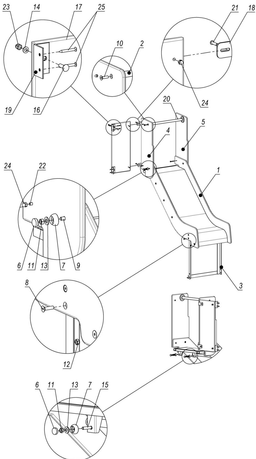
Рисунок 20 – Схема збирання гірки 0,7м з однією перегородкою
