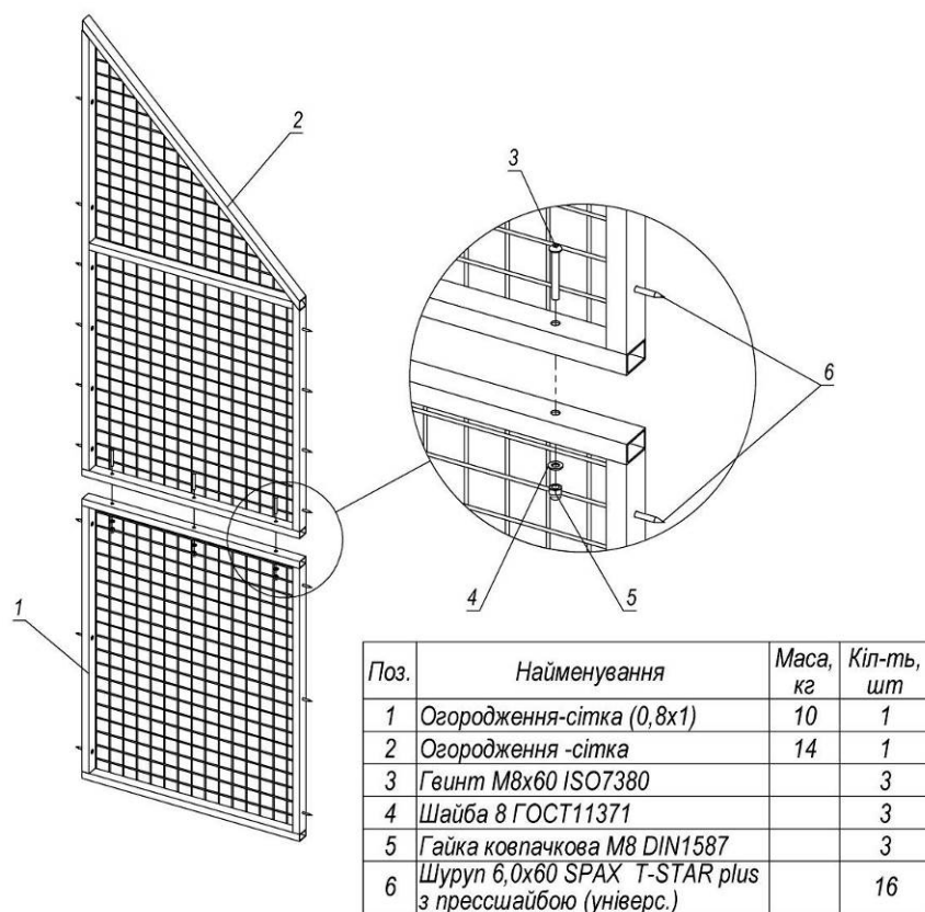
Рисунок 16 – Схема збирання огородження-сітка
