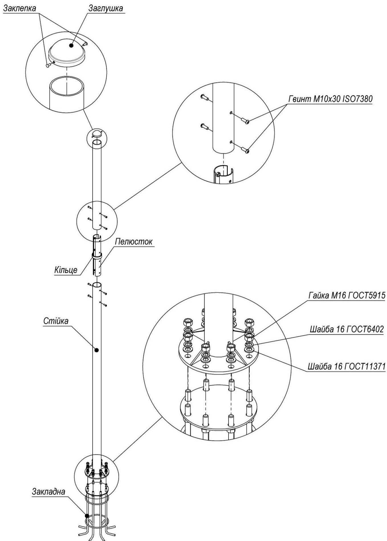
Рисунок 23 – Схема складання Стойки
