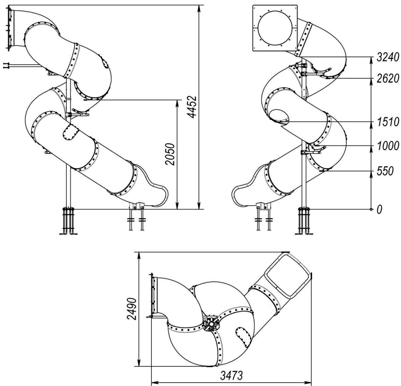
Рисунок 22 – Габаритні розміри
