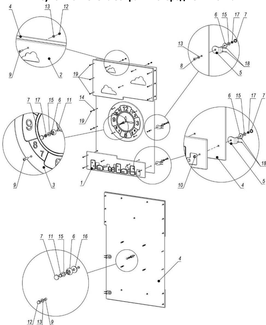
Рисунок 17 – Схема збирання панелі з годинником
