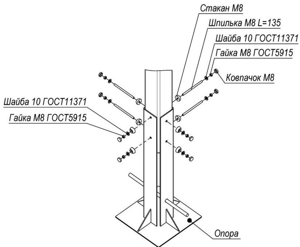
Рисунок 12 – Схема з'єднання опори з брусом
