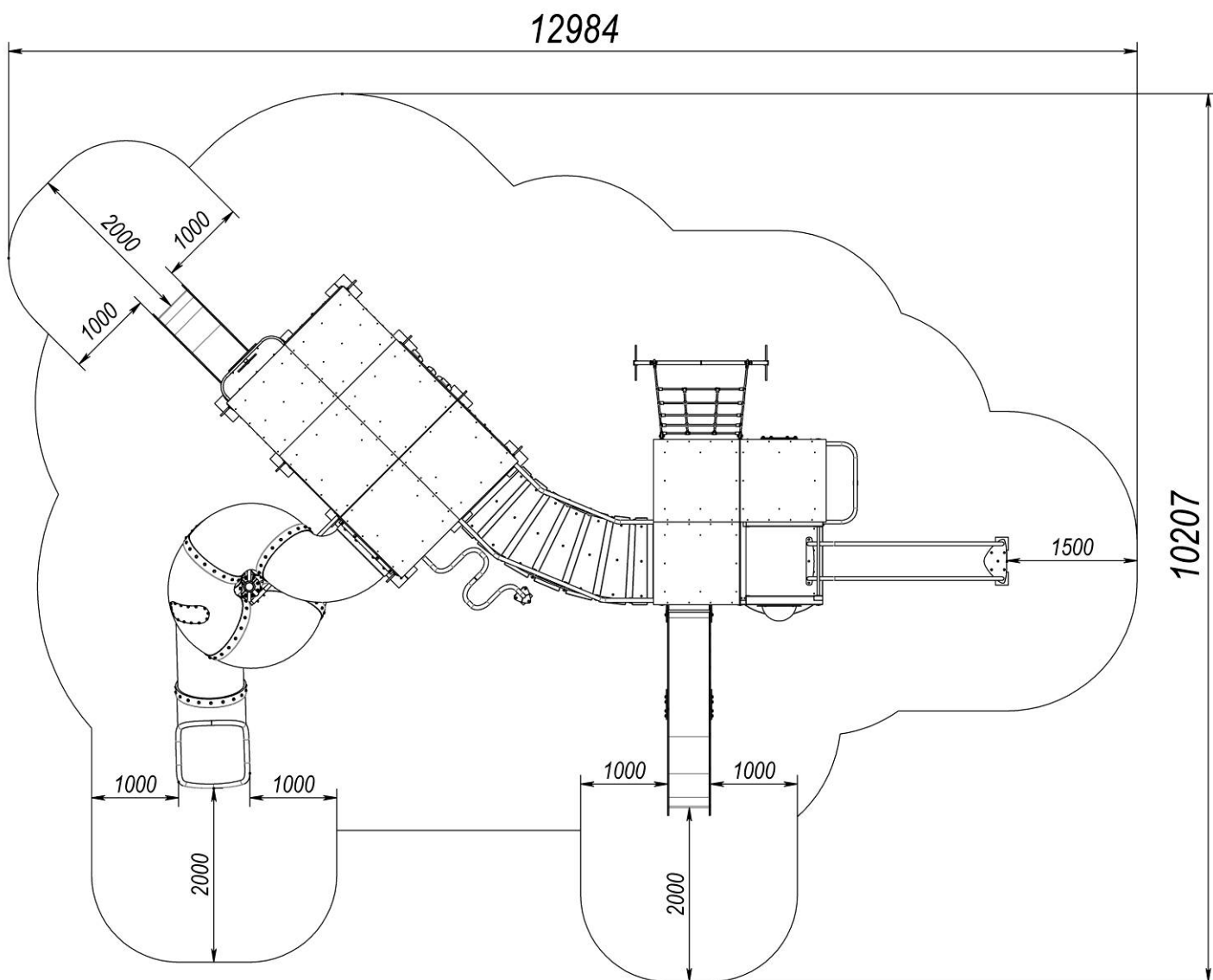
Рисунок 1 – Зона приземлення
