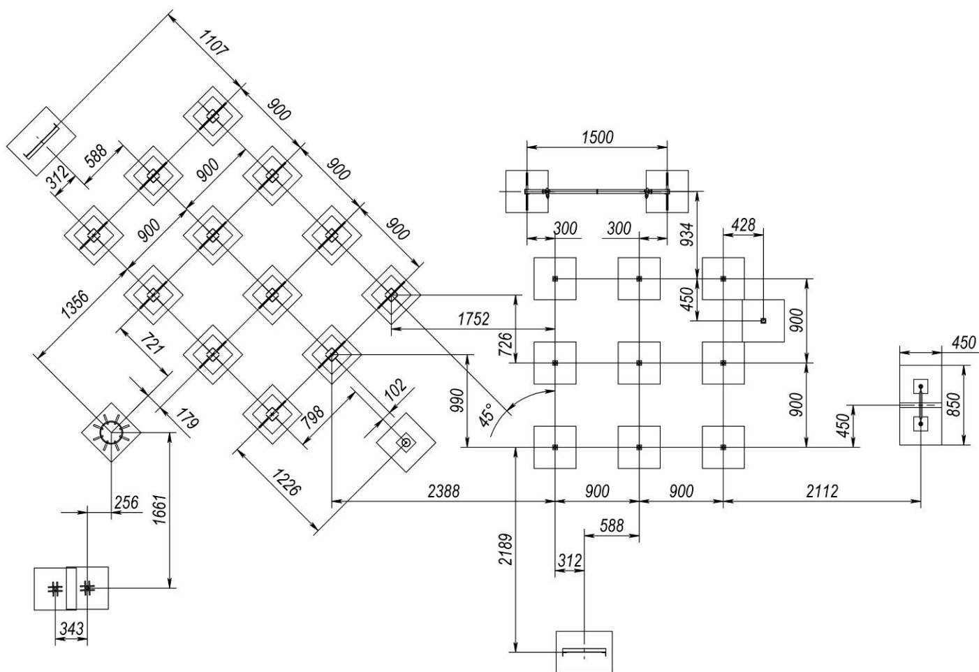
Рисунок 2 – Схема розташування фундаментів
