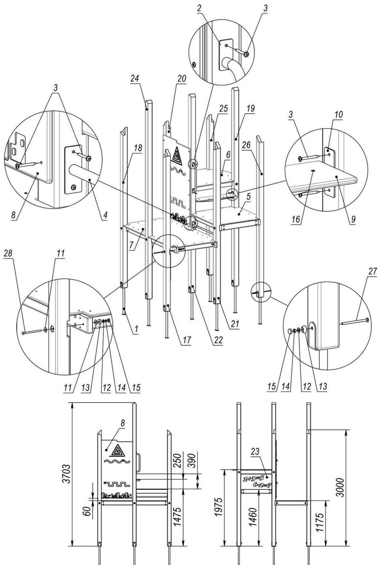
Рисунок 14 - Вежа велика (1,2-2м)
