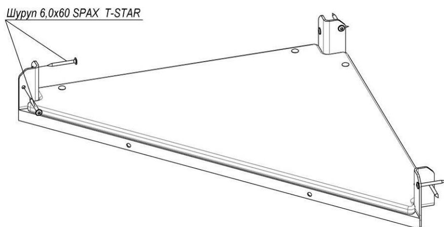
Рисунок 4 – Схема складання платформи
