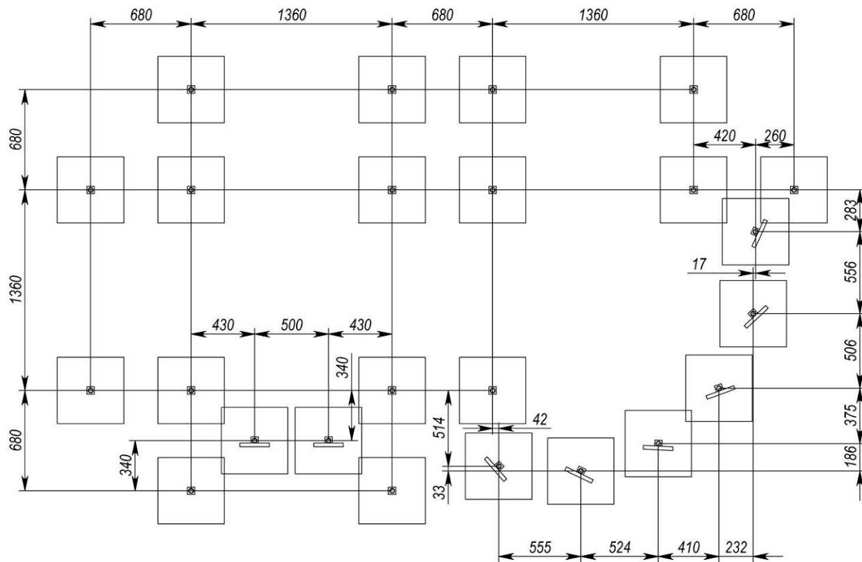
Рисунок 2 – Схема розташування фундаментів
