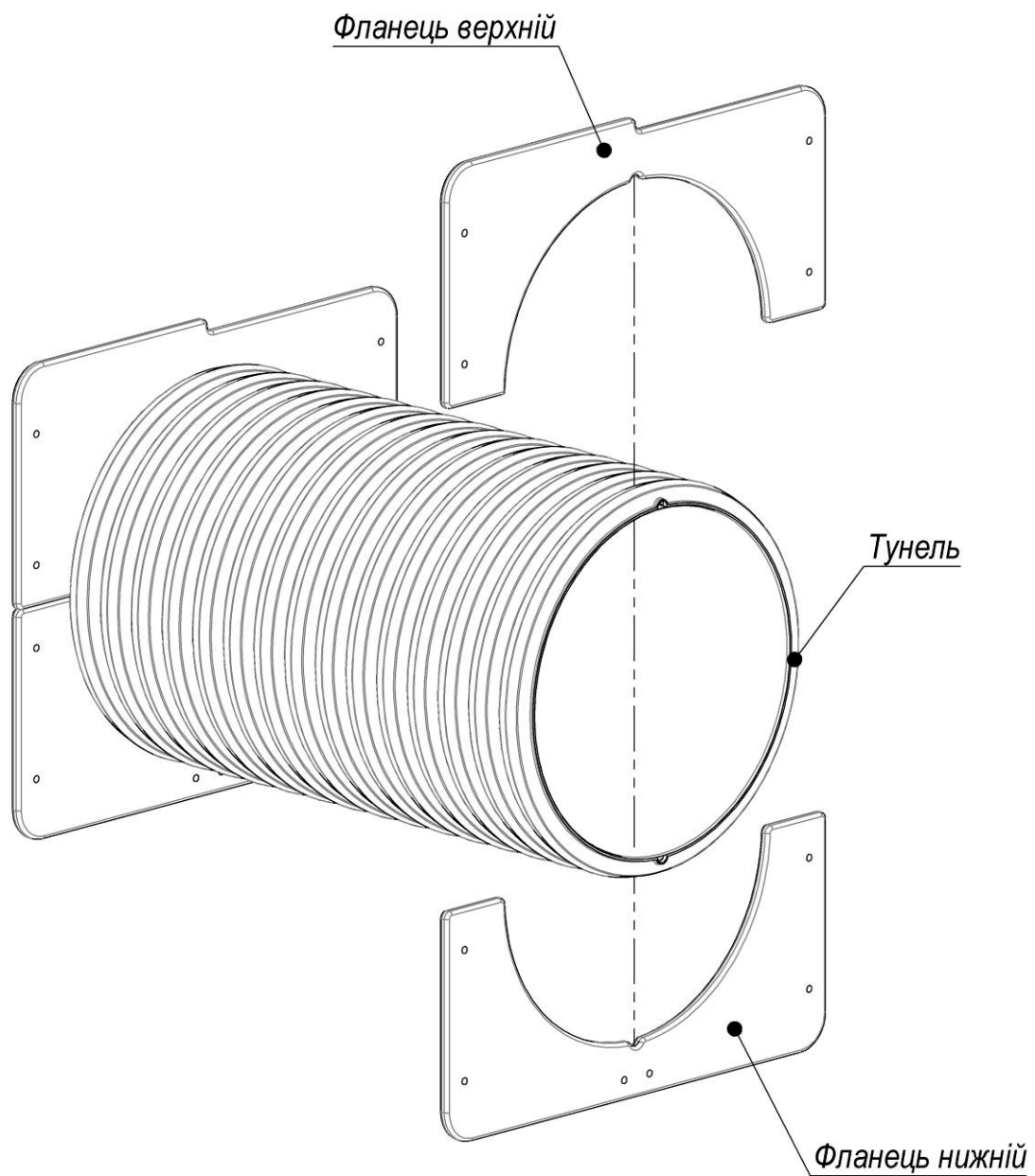
Рисунок 8 – Схема складання тунельного переходу
