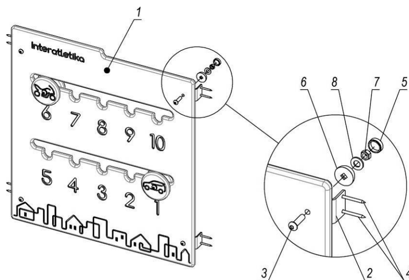
Рисунок 6 – Схема складання пенька
