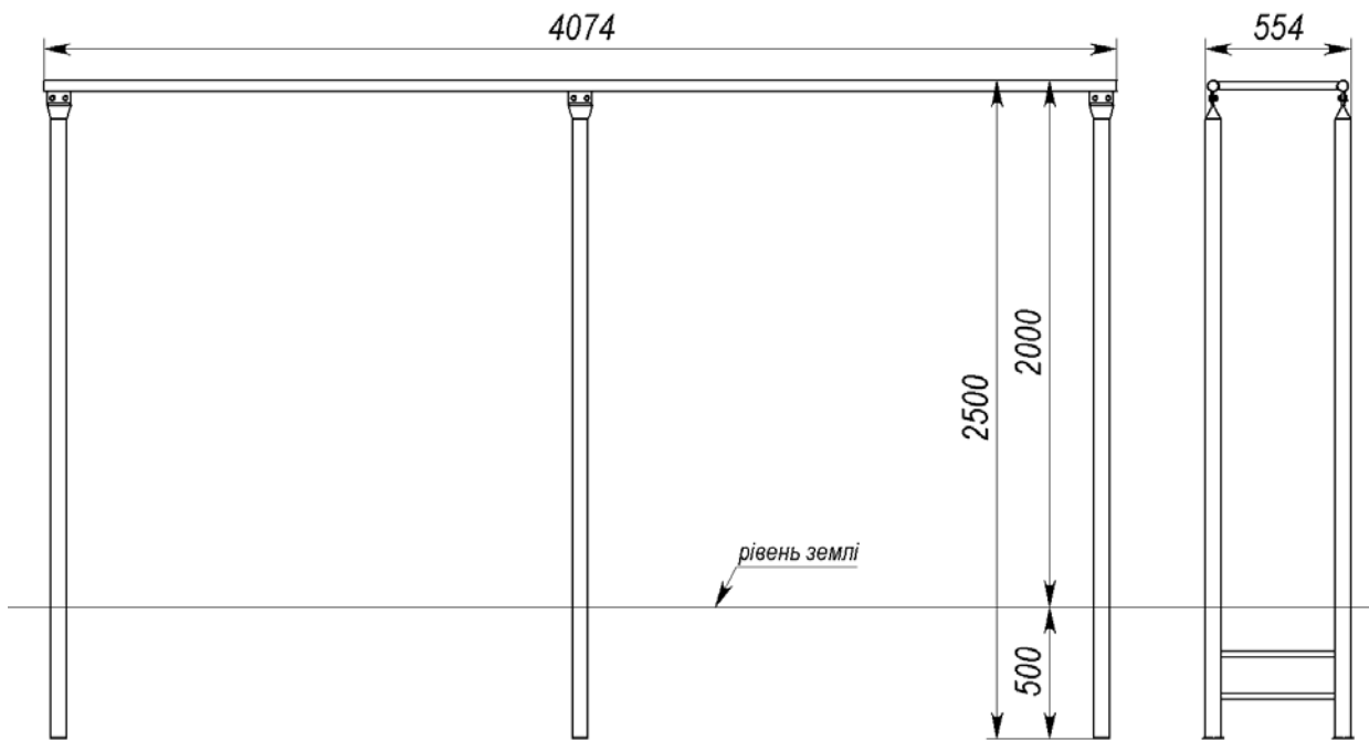
Рис. 2 Габаритні розміри
