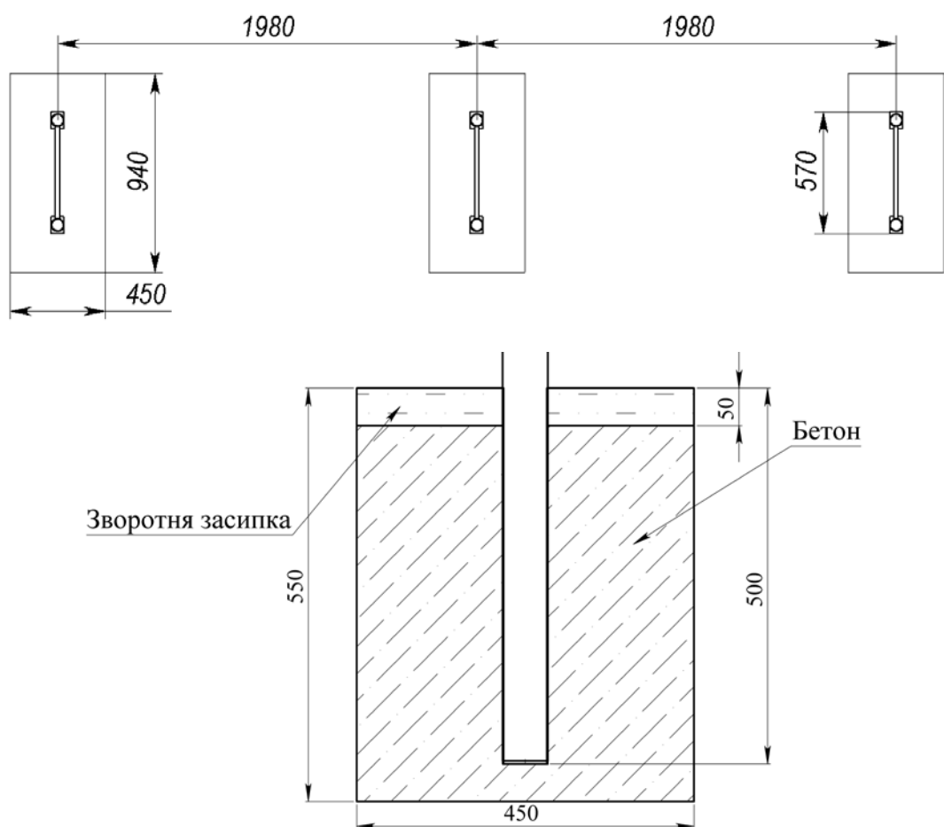
Рис. 3 Схема монтажу фундаментів
