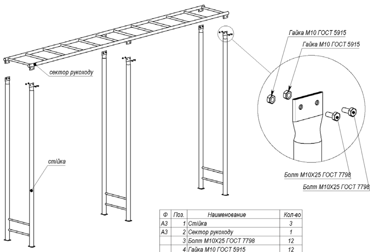
Рис. 1 Комплектація та порядок збирання
