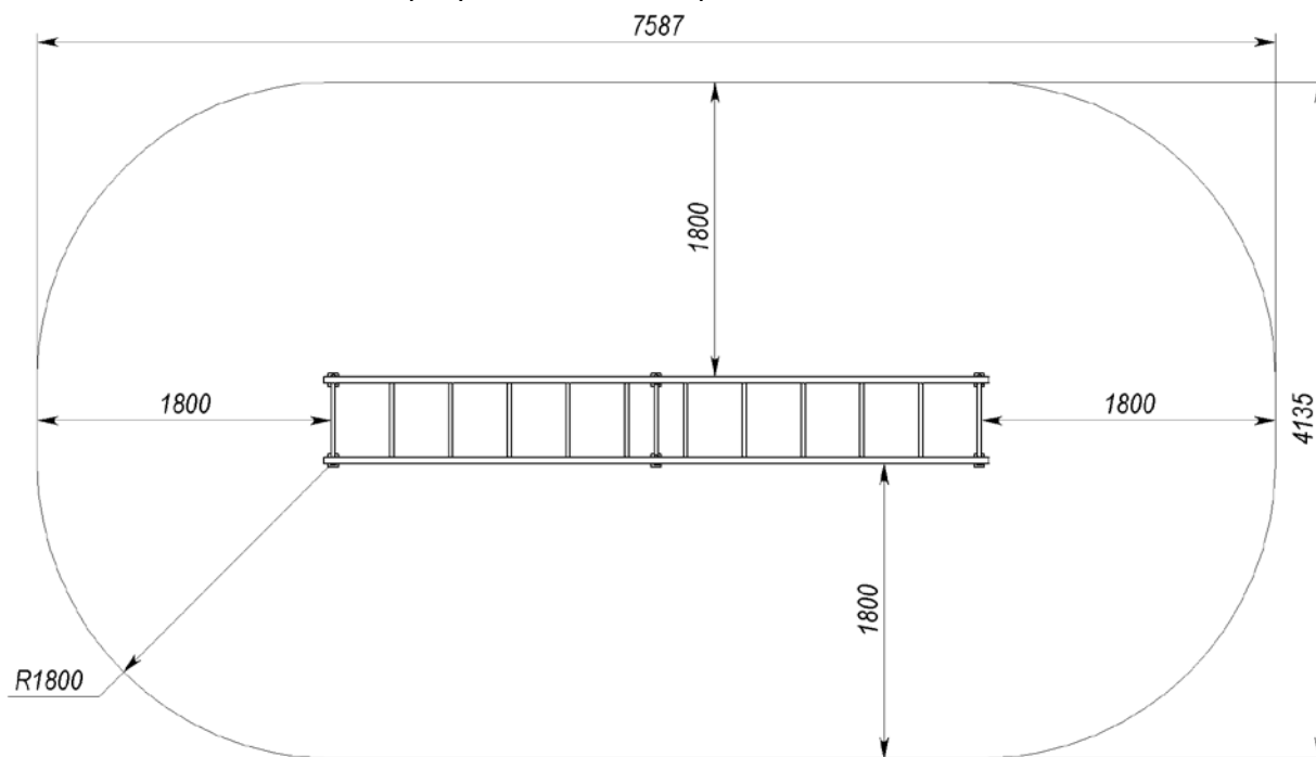
Рис. 4 Зона безпеки
