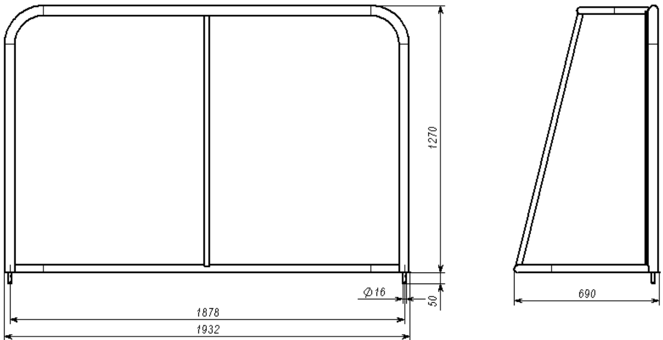
МАЛЮНОК 2 «Габаритні розміри, схема монтажу виробу»
